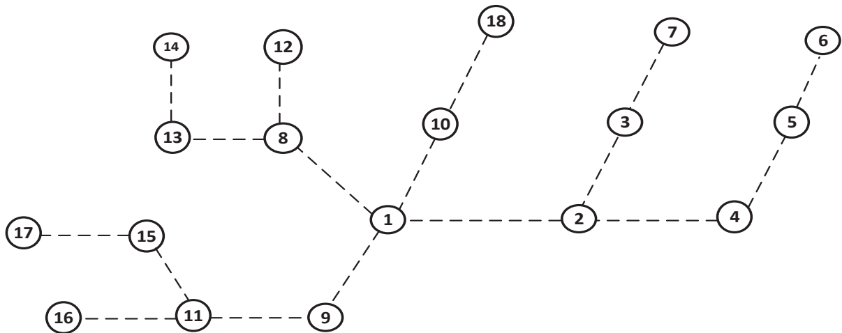
Figure 36 : Topologie du réseau associée au canal dédié aux beacons
