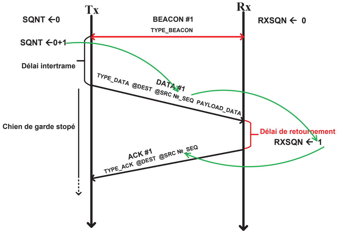
Figure 47 : Diagramme de séquence quand la Data est perdue, il n'y a pas d'acquiescement
