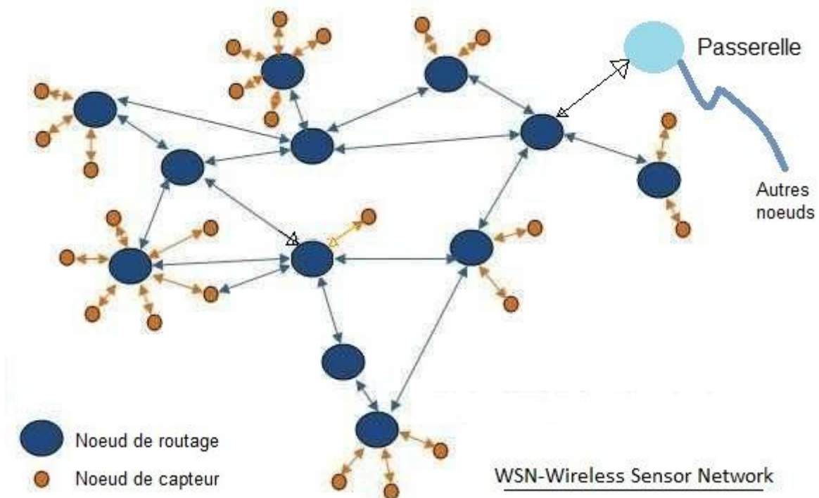
Figure 1.2 Réseau de capteurs
