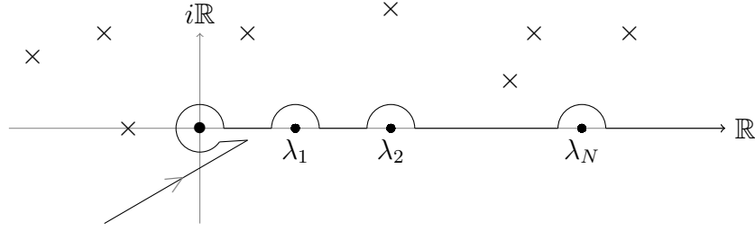
FIGURE 2.1: La courbe \Gamma^\nu(\eta) . \lambda_1, \dots, \lambda_N sont les résonances positives sortantes de H et les croix sont les valeurs propres discrètes de H dans \overline{\mathbb{C}}_+ .
