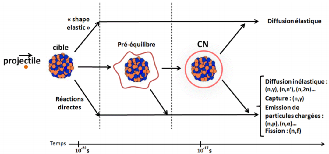
FIGURE 1.1: Représentation de différents mécanismes de réaction. Source : Figure dans [13].
