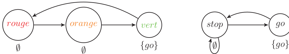
FIGURE 1 – Un exemple d'un modèle de feu tricolore, ainsi que son abstraction dans laquelle les états rouge et orange ont été groupés en un état stop .
