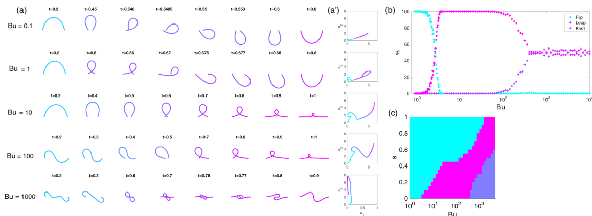
FIGURE 1.8 – Visualisation de l'apparition de différentes formes au cours du buckling (a). Évolution de la forme du filament au cours du temps pour différentes valeurs de Bu . On peut observer les trois formes ( flip , loop et knot ) correspondant aux trois régimes de buckling . (a'). Évolution de l'amplitude des deux premiers modes de Fourier de la courbure du filament pour chacune des simulations présentées en (a). L'intérêt de ces graphiques est développé dans le Chapitre 8. (b). Prédominance de chaque forme en fonction de Bu , exprimée en pourcentage d'apparition sur 500 simulations. (c). Prédominance de chaque forme en fonction de Bu et a .
