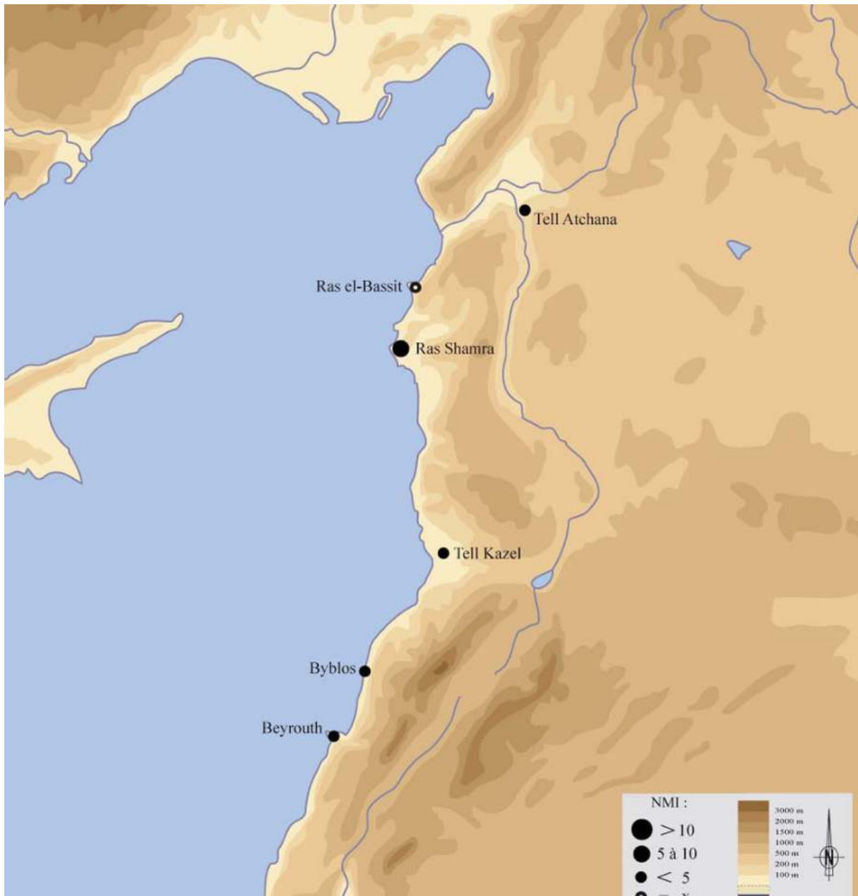
Planche 135. Carte de distribution de la céramique BW au Levant nord.
