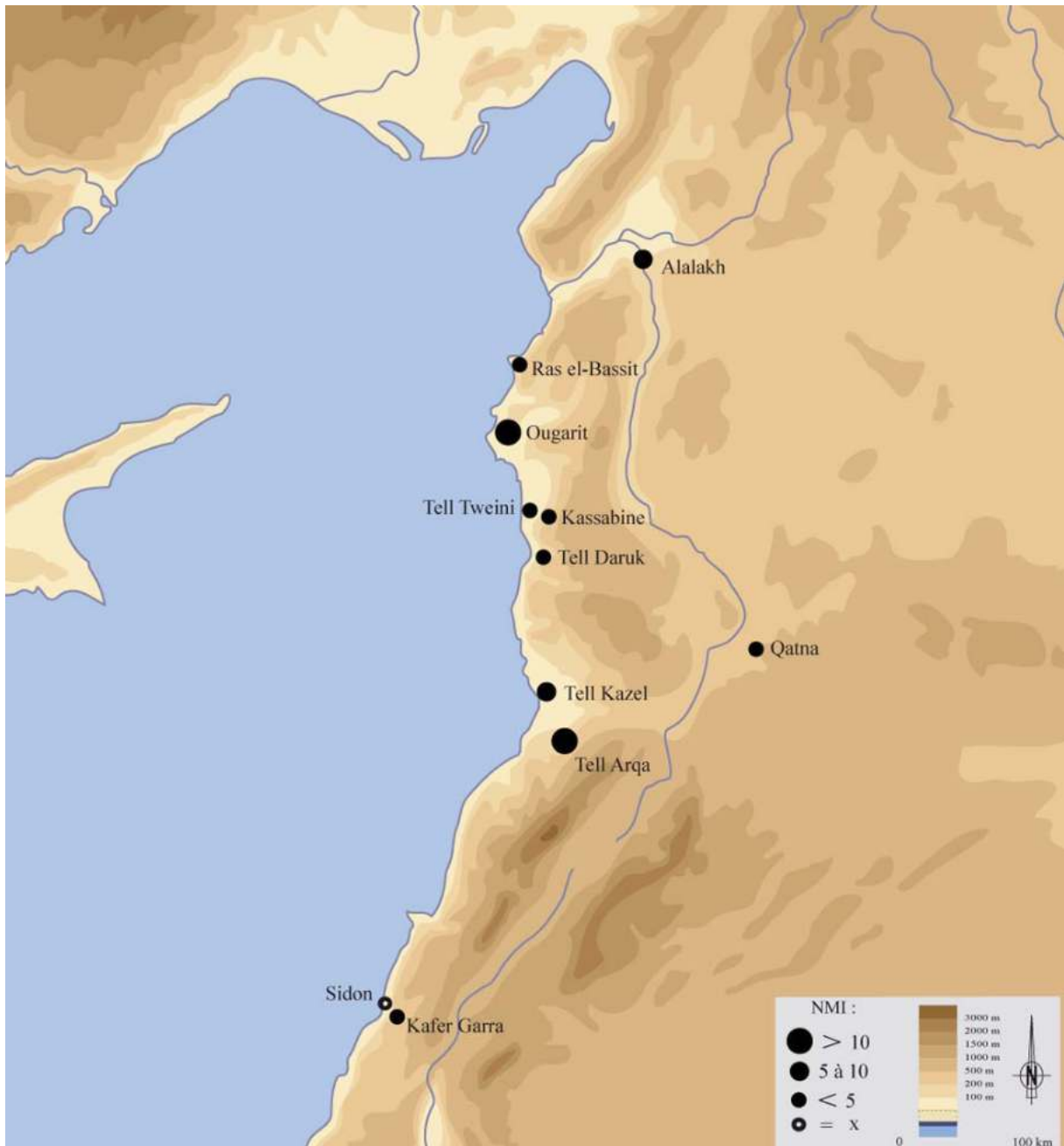
Planche 60. Distribution de la céramique WP CLS au Levant nord.
