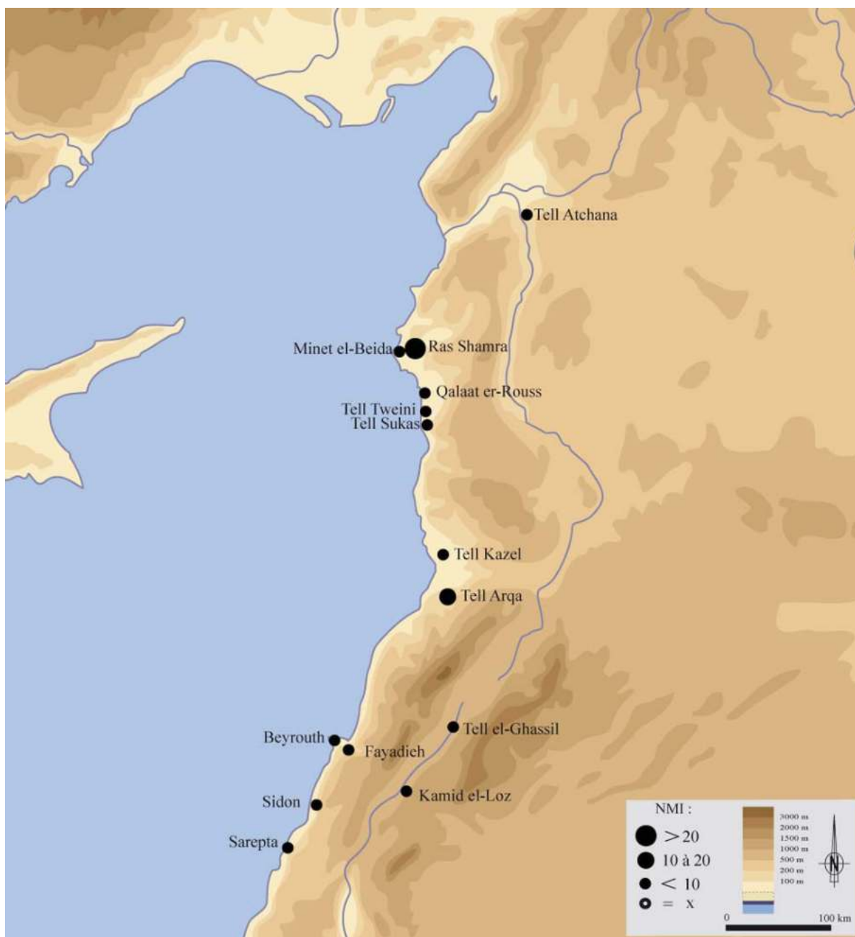
Planche 81. Carte de distribution de la céramique BC au Levant nord.
