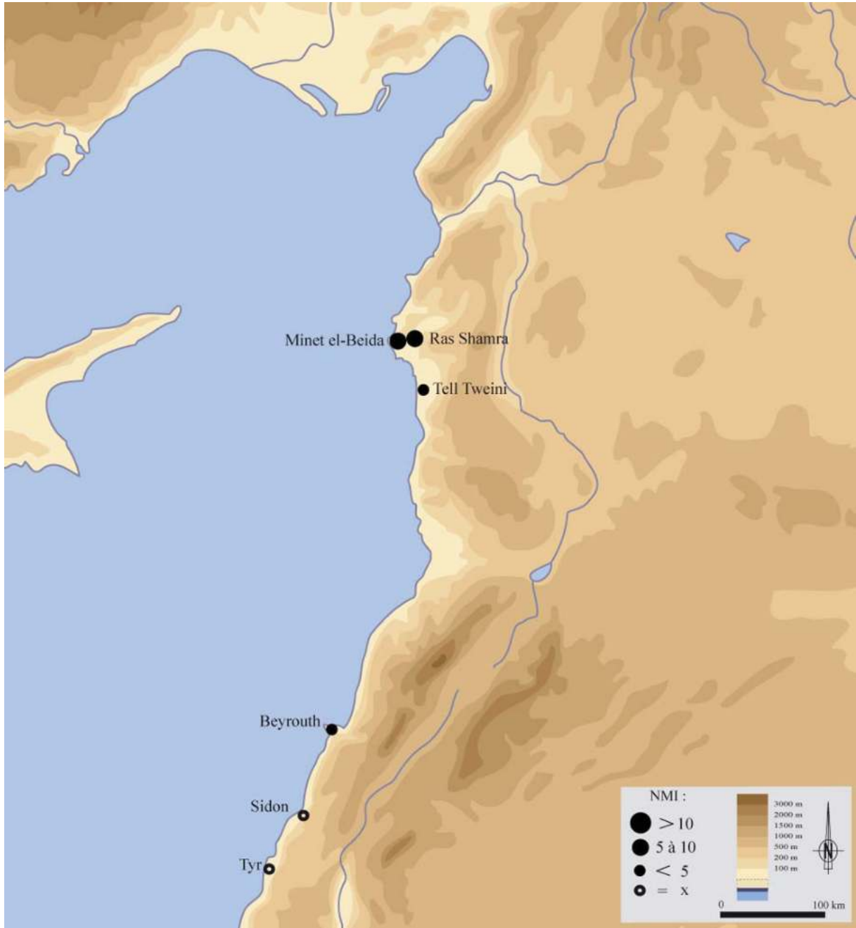
Planche 132. Carte de distribution des pithoi chypriotes au Levant nord.
