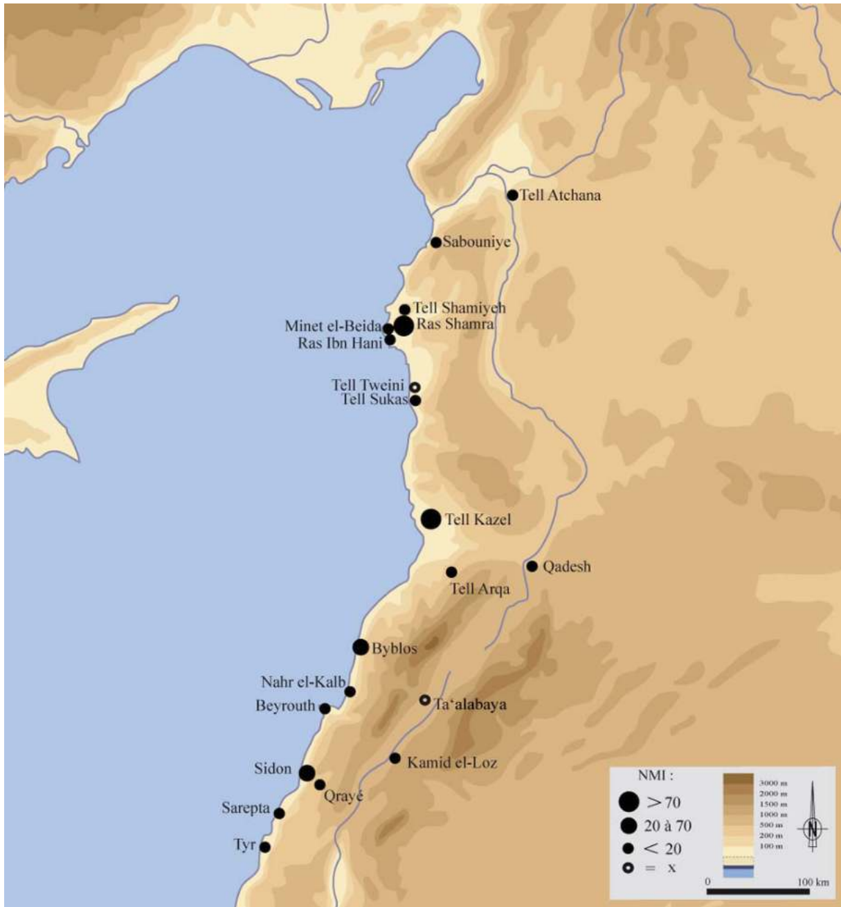
Planche 126. Carte de distribution de la céramique WSh au Levant nord.
