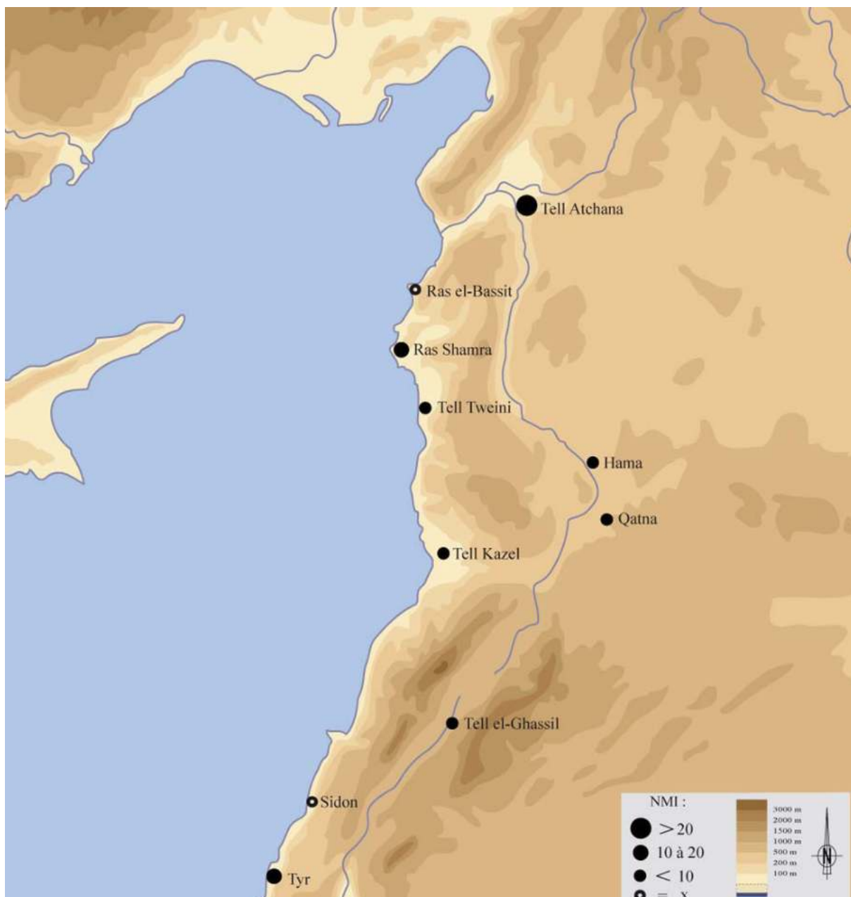
Planche 139. Carte de distribution de la céramique WS I au Levant nord.
