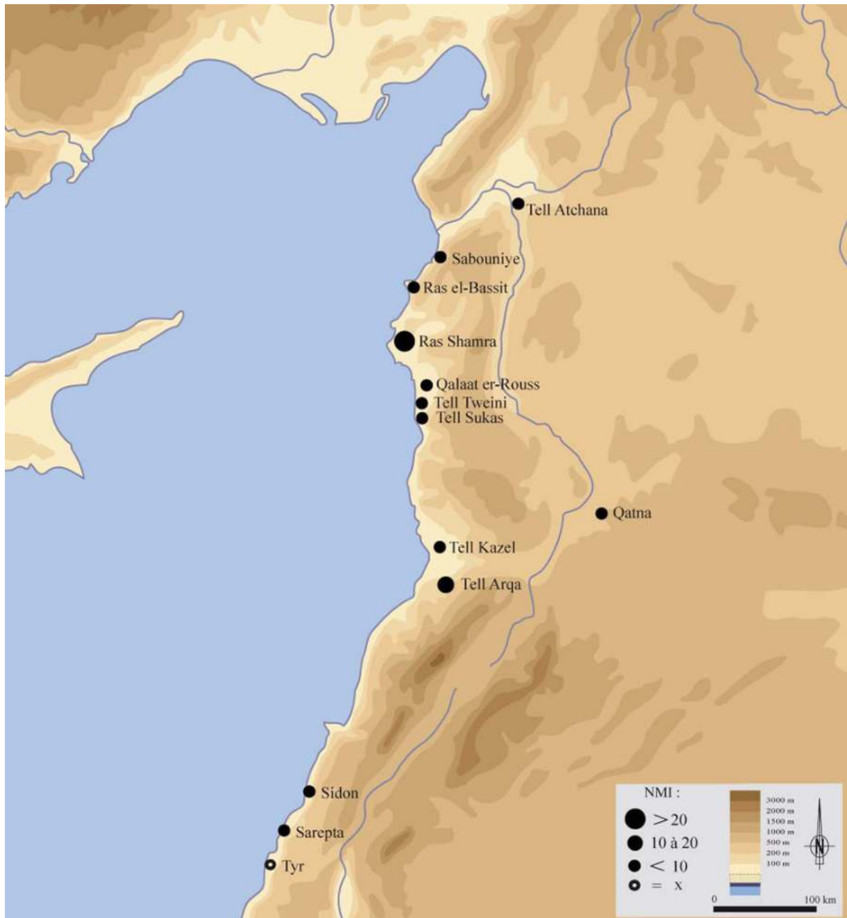
Planche 75. Carte de distribution de la céramique RoB/RoR au Levant nord.
