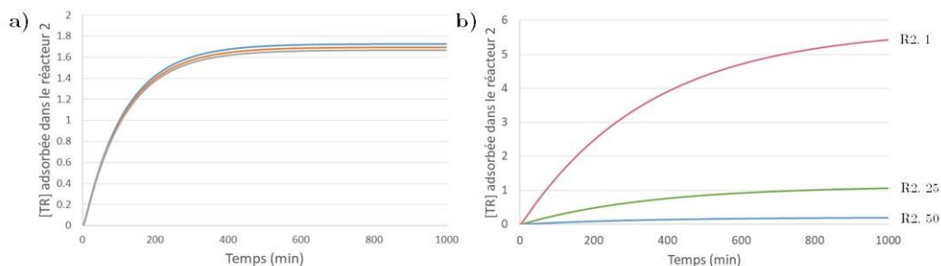
Figure 34 - Modélisations des concentrations en terres rares adsorbées dans la résine selon la section, dans le cas de la configuration 3, avec un débit élevé (a) et un débit divisé par 10 (b)
