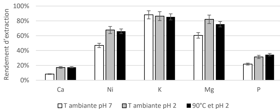
Figure 29 - Effets du pH et de la température sur les rendements d'extraction en nickel et minéraux à partir des feuilles broyées de R. bengalensis
