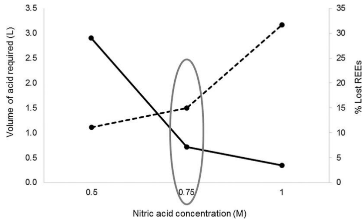
Figure 39 - Volume (trait plein) et perte en terres rares (pointillés) en fonction de la concentration d'acide nitrique nécessaire pour éliminer l'aluminium de la résine Amberlite IRN77 [ACL6]
