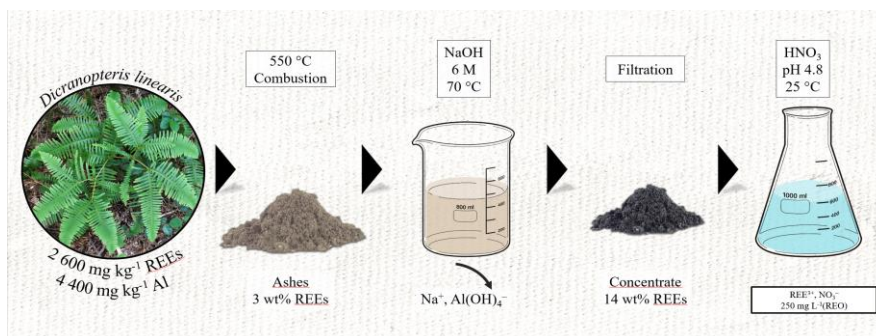
Figure 26 - Résumé graphique du procédé de récupération des terres rares depuis les cendres de D. linearis
