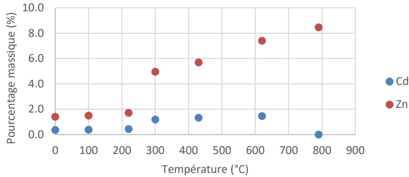
Figure 16 - Pourcentage massique de cadmium et de zinc dans les cendres de N. caerulea selon la température de combustion
