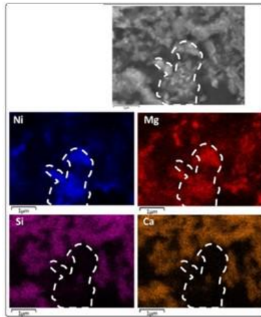
Figure 18 - Analyse SEM-EDX des cendres de feuilles de R. bengalensis brûlées à 900 °C [ACL2]
