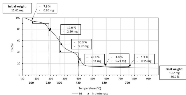
Figure 15 - Profil thermogravimétrique obtenu pour l'hyperaccumulateur de zinc et de cadmium N. caerulea [ACL9]
