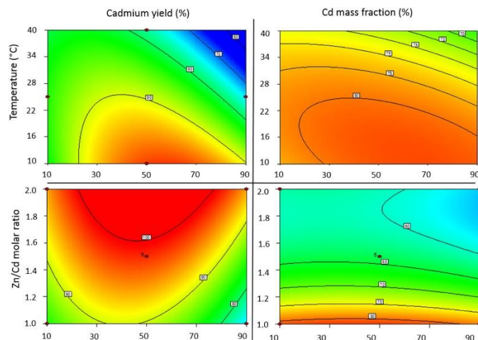
Figure 24 - Surfaces de réponse liées à la récupération du cadmium par cémentation (rendement et pureté) en fonction du ratio molaire Zn / Cd et de la température [ACL9]
