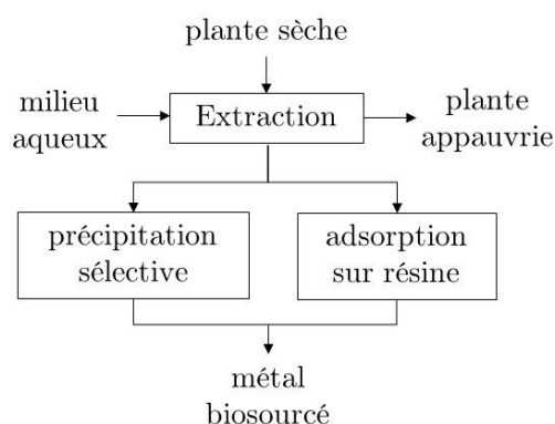
Figure 27 - Démarche générale mise en œuvre pour la récupération d'un métal par hydrométallurgie depuis la biomasse d'un hyperaccumulateur
