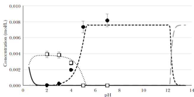
Figure 38 - Spéciation du lanthane dans une solution contenant de l'acide oxalique et de l'EDTA (l'expérience est représentée par des points, les simulations par des lignes) : La^{3+} —, La_2Ox_3 ..... et □, LaEDTA - - - et ●, et La(OH)_2 — -
