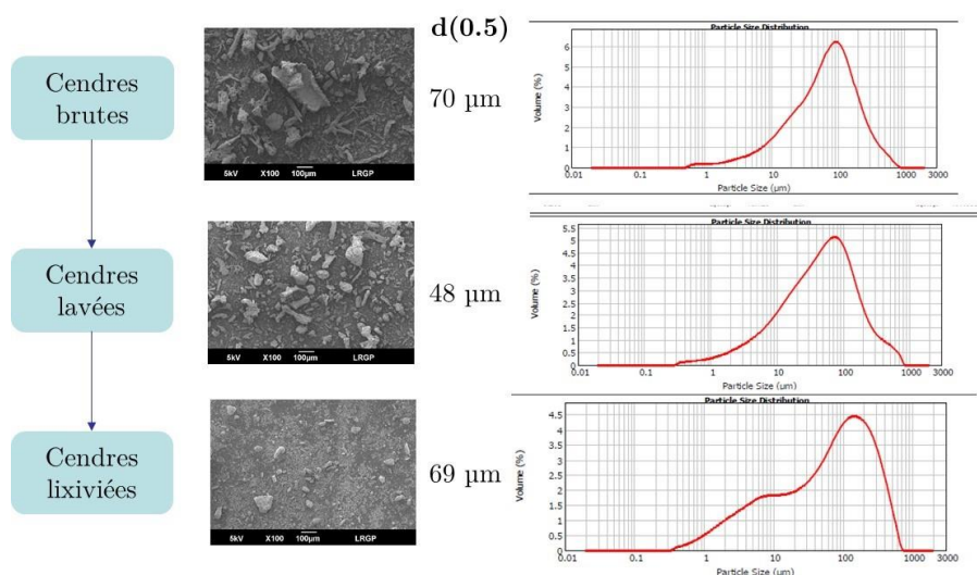
Figure 17 - Évolution morphologique des cendres de l'hyperaccumulateur O. chalcidica au cours du procédé de récupération du Ni
