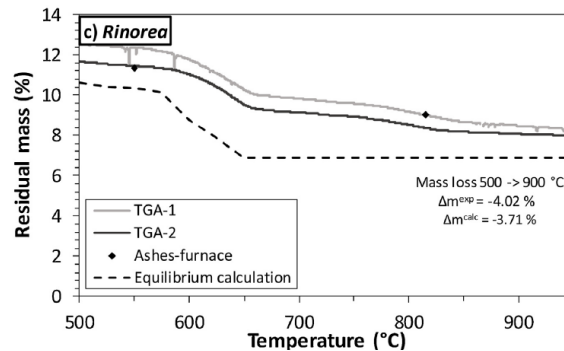
Figure 19 - Simulation de la masse résiduelle lors de la combustion de R. bengalensis et comparaison avec les valeurs expérimentales [ACL2]
