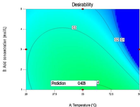
Figure 23 - Surface de réponse de la désirabilité en fonction des conditions de lixiviation des cendres de l'hyperaccumulateur O. chalcidica [ACL8]
