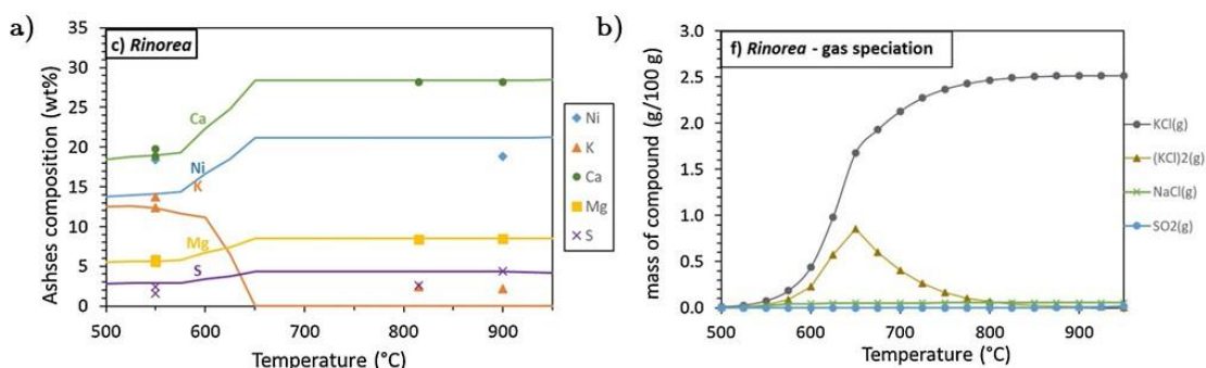
Figure 20 - Simulations du comportement des éléments de R. bengalensis lors de sa combustion en fonction de la température : composition des cendres et comparaison avec l'expérience (a), masse de gaz liés aux inorganiques émise (b) [ACL2]
