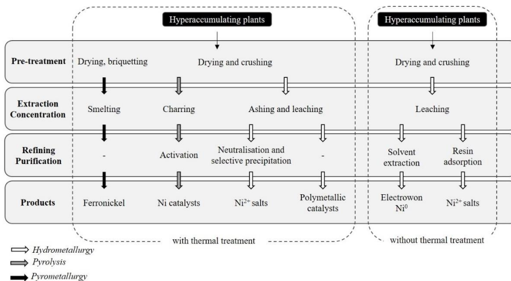
Figure 14 - Les différentes voies de récupération de la biomasse depuis les hyperaccumulateurs de nickel [COSI]
