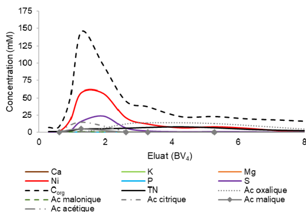
Figure 37 - Courbes caractéristiques de l'élution (HCl 1,6M) d'un extrait d' O. chalcidica avec la résine Dowex M4195
