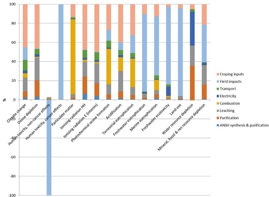
Figure 40 - Contributions environnementales des différentes étapes du procédé de production de l'ANSH par agromine à partir de O. chalcidica avec un transport de la biomasse de 50 km [ACL11]
