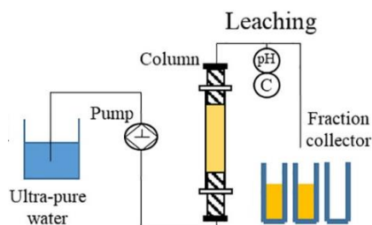
Figure 28 - Schéma expérimental d'un dispositif en colonne d'extraction depuis la biomasse (adaptée de [ACL5])
