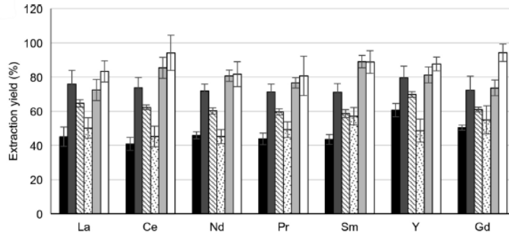
Figure 30 - Taux d'extraction des terres rares dans l'eau ■, l'acide citrique (1 M, pH 1,6)■, l'acide citrique (1 M, pH 4) ▨, le citrate (1 M, pH 8) ▩, H 2 SO 4 (0,25 M) □ et Na 2 EDTA (0,05 M) □ [ACL3]
