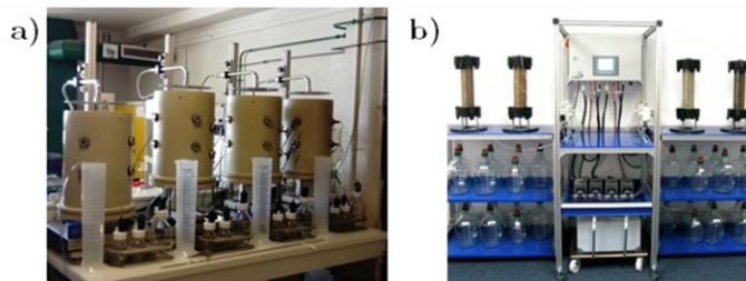
Figure 10 - Photographies de 4 des 12 lysimètres de laboratoires achetés (a) et du dispositif normalisé de lixiviation (b)
