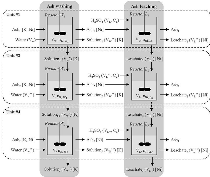
Figure 43 - Schéma de principe de gestion des lots de cendres d'hyperaccumulateurs permettant de diminuer la quantité d'entrants [ACL 7]
