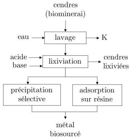
Figure 21 - Démarche générale mise en œuvre pour la récupération d'un métal par hydrométallurgie depuis les cendres d'hyperaccumulateurs
