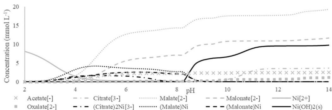
Figure 35 - Simulation de la spéciation du nickel dans les extraits aqueux obtenus avec O. chalcidica en fonction du pH [ACL5]
