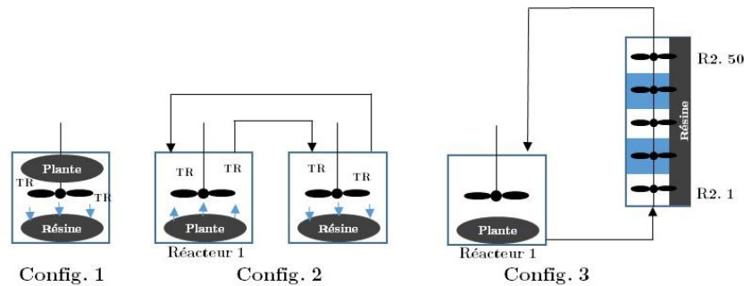
Figure 33 - Schéma des différentes configurations d'extraction des terres rares modélisées [S4]
