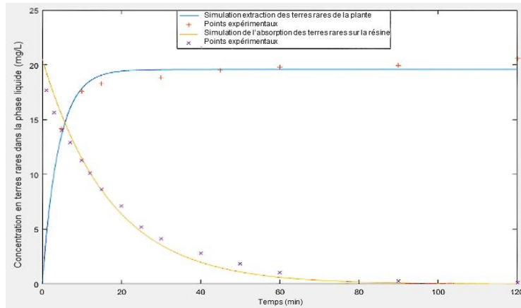
Figure 32 - Cinétiques de transfert des terres rares par mesure de concentrations en phase liquide, de D. linearis à la solution (points expérimentaux en rouge et modélisation en bleu), de la solution à la résine (points expérimentaux en violet, et modélisation en orange)
