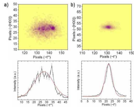
FIG. 3.13 – a) Diffraction coh rente du satellite associ e   l'ODC en (0, 0, 2 - 2\delta) b) Diffraction coh rente du satellite associ e   l'ODS en (0, 0, 1 - \delta) . L'une contient des tavelures, pas la seconde.
