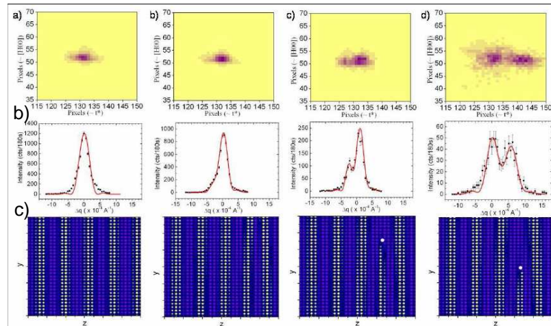
FIG. 3.14 – a) Figure de diffraction du satellite magn tique (0, 0, 1 - \delta) pour diff rentes positions du faisceau sur l' chantillon. Chaque image correspond   une translation de 20\mu m de l' chantillon. Le point remarquable est qu'une fois d doubl s, les pics ne s' largissent pas. b) Profils correspondants aux images 2D de dessus, le long de la direction radiale. Les profils en rouge correspondent aux simulations num riques de la figure de dessous. c) Simulation d'une dislocation magn tique dans le plan (001) . Les fronts d'onde magn tiques sont repr sent s en jaune, les points correspondent aux atomes de Cr. Les simulations ont  t  r alis es sur une bo te de 60*60*60 atomes. La largeur des profils simul s a  t  ajust e par un m me facteur d' chelle pour les ajuster aux largeurs des profils exp rimentaux.
