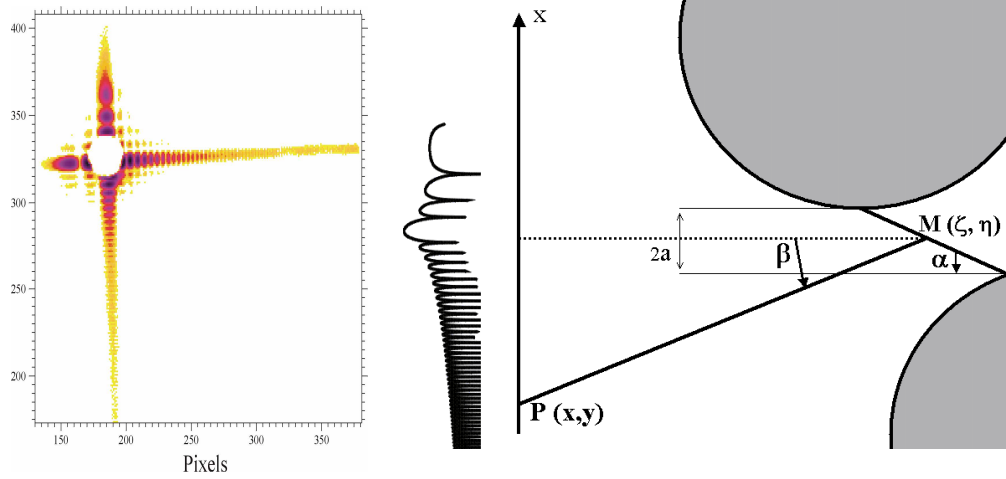
FIG. 2.13 – a) L'asymétrie de la figure de diffraction résulte donc de l'asymétrie de l'objet qui lui a donné naissance. Cliché de diffraction asymétrique lié à b) l'asymétrie des fentes.
