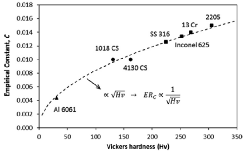
FIGURE 3.8. – Evolution de l'efficacité de coupage en fonction de la dureté Vickers de plusieurs alliages métalliques - D'après Arabnejad et al. [7]
