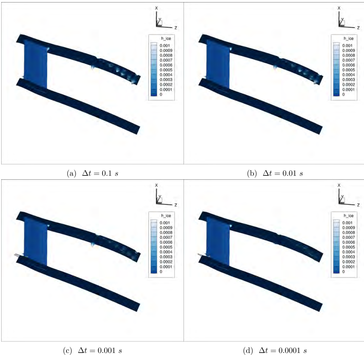
FIGURE 8.9. – Épaisseurs de glace pour une durée de 120s, simulées dans le domaine EGV pour la distribution de référence PSD_1 , avec la méthode de mise à jour des normales pour différents pas de temps
