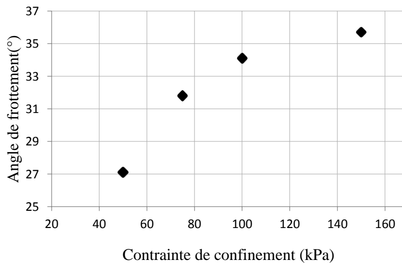
Figure 61 : Angle de frottement en fonction de la contrainte de confinement (FIR = 150%).
