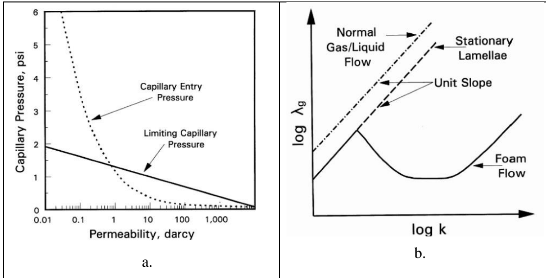
Figure 28 (a) Variation de la pression capillaire d'entrée d'air et la pression capillaire limite P_c en fonction de la perméabilité k du milieu et (b) Variation de la mobilité du gaz \lambda_g en fonction de la perméabilité k du milieu poreux (Khatib et al., 1988).
