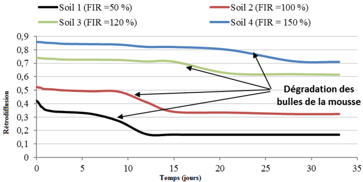
(b) Effet de la granulométrie sur le phénomène de coalescence (région supérieure 10-64 mm)
