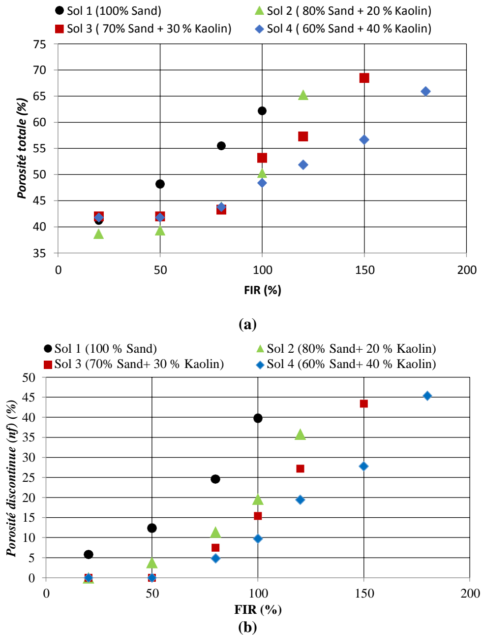
Figure 38 : Effet de la mousse sur la porosité totale et le pourcentage de gaz généré dans le sol traité (%). (a) Effet de FIR sur la porosité totale. (b) Effet de FIR sur le volume de gaz généré dans le sol traité
