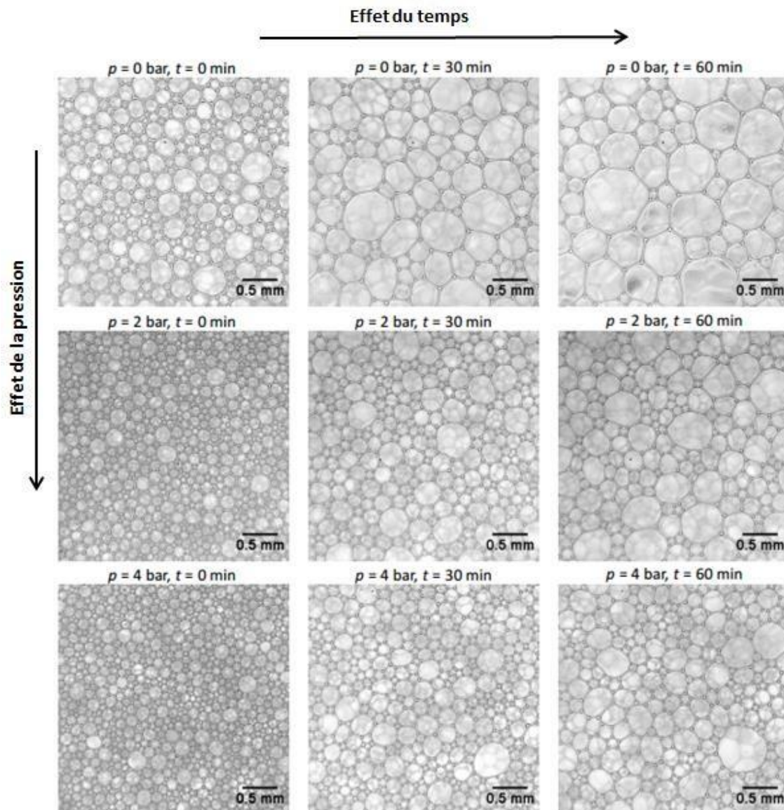
Figure 12 : Vieillesse de la mousse soumise à différentes pressions P (Wu et al. 2018)
