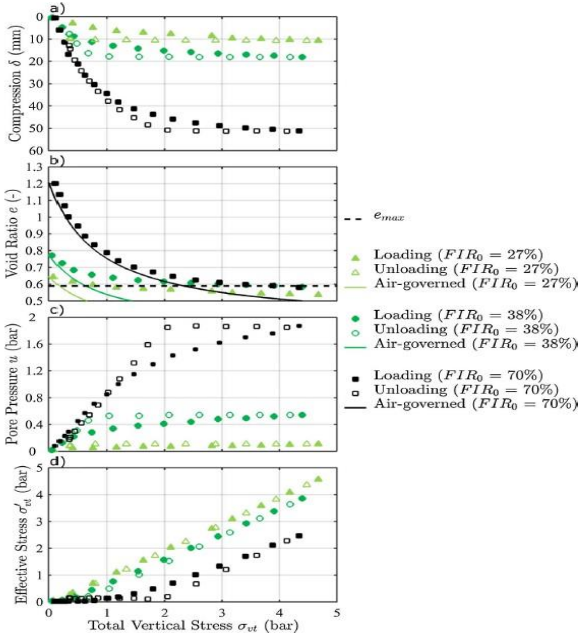
Figure 18 : Essai de compression non drainée sur un échantillon sableux traité avec différents pourcentage de FIR (Mori et al. 2018b)
