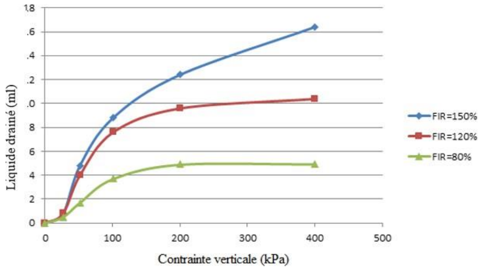
Figure 56 : Effet de la dégradation de la mousse sur le tassement du sol traité. (a) Effet de la compressibilité des bulles de la mousse sur le tassement du sol traité. b) Volume du liquide drainé de la mousse en fonction de la consolidation de la FIR
