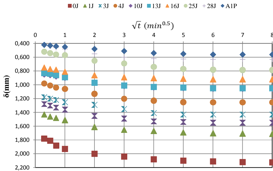
Figure 65 : Tassement en conditions œdométriques sous une contrainte verticale de 52 KPa (0J : premier jour, XJ=X jours, A1P : Sol non traité)
