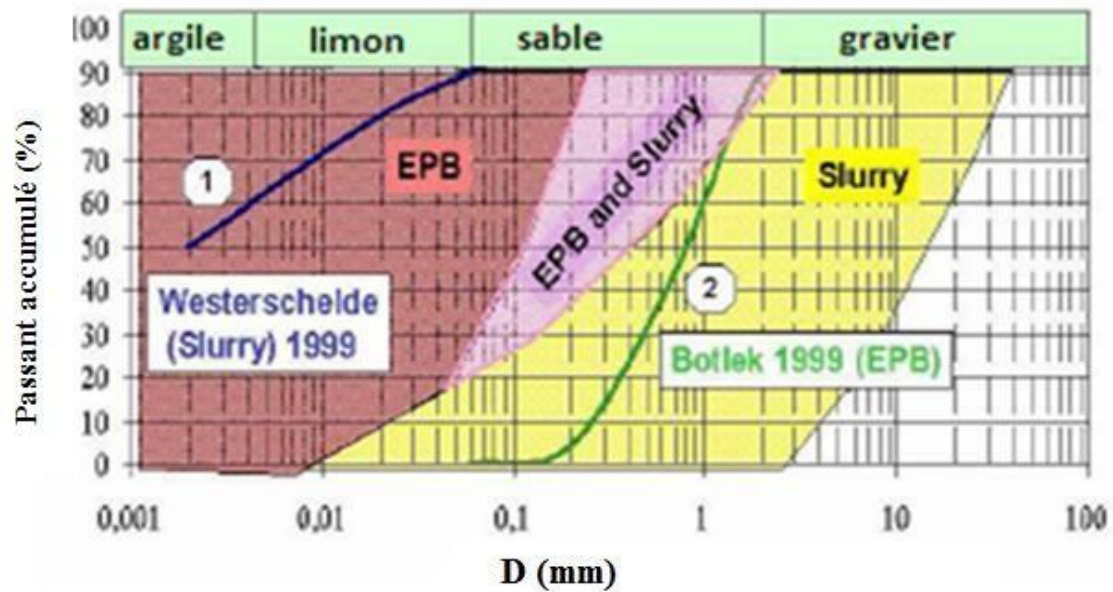
Figure 4 : Domaine d'utilisation des EPB et Slurry (Maidl et al. 2012)
