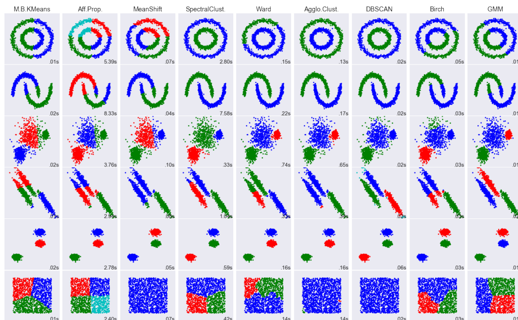
FIGURE 2.11 – Comparaison des techniques de clustering sur plusieurs jeux de données générés tiré de Bob Baxley http://rjbxley.com . (MB Kmeans : Minibatch Kmeans ; Aff. Prop. : Affinity Propagation, Agglo. Clust : Agglomerative Clustering, DBSCAN : Density Based Spatial Clustering of Applications with Noise, GMM : Gaussian Mixture Model)
