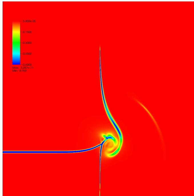
(b) Problème de Riemann (Eqs de Saint-Venant)
