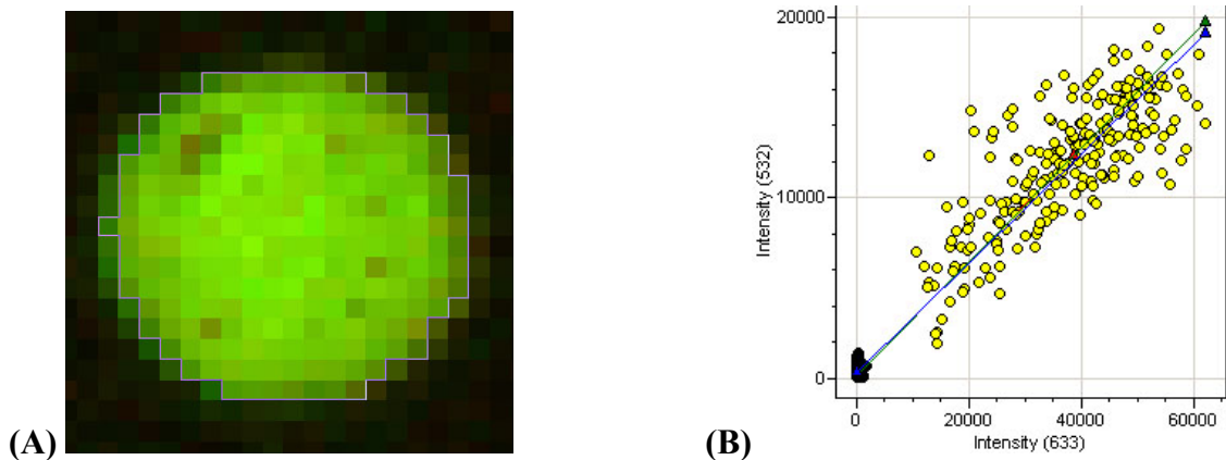
Figure 18. Segmentation et mode de calcul des niveaux d'intensités des spots (d'après le logiciel d'analyse d'images GenepixPro 5.0, Axon Inc. ). (A) Le mode de segmentation appliqué est « irregular feature ». Le spot n'est pas nécessairement circulaire et l'algorithme de segmentation cherche à faire le contour exact du spot. (B) Représentation graphique, pour chaque pixel du spot, des intensités en Cy3 versus les intensités en Cy5 . Quantification du niveau d'intensité des pixels appartenant au signal (jaune) et des pixels appartenant au bruit de fond (noir).
