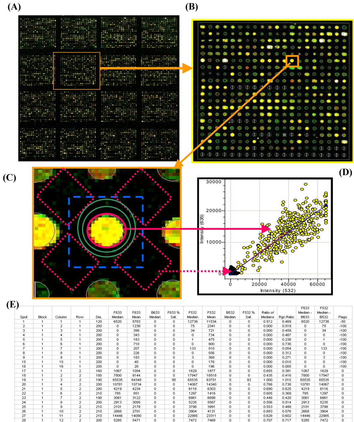
Figure 11. Acquisition des données par les logiciels d'analyse d'images. (A) Extrait d'une image composite de puce à ADN Myochip . (B) Localisation et segmentation des spots : zoom sur un cadran de la puce. La grille de localisation et de segmentation est matérialisée en blanc. Les spots défectueux et les spots non identifiés (absents) sont respectivement marqués d'une croix et d'un trait vertical. Les spots atteignant la saturation sont blancs. (C) Exemples de méthodes de segmentation. Selon Scanalyze, le signal est estimé à l'intérieur du cercle rose et le bruit de fond à l'intérieur du carré bleu. D'après Genepix®, le cercle rose définit les pixels appartenant au signal ; les carrés en pointillé rose matérialisent les zones d'estimation du bruit de fond. Les cercles concentriques vert définissent la zone de calcul du bruit de fond dans les logiciels Imagene® et QuantArray®. La « zone tampon » est définie par l'intervalle entre le cercle rose du spot, les carrés roses et le premier cercle vert ; elle limite l'introduction des valeurs aberrantes (artefacts) dans la mesure des signaux.
