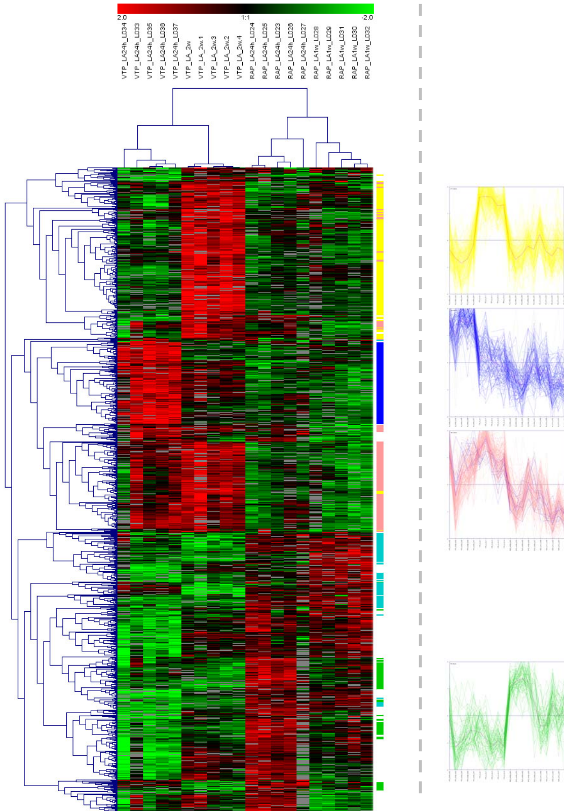
Figure 29. Classification hiérarchique ascendante versus K-moyennes (Etude réalisée à la demande de S. Nattel). (A) Classification hiérarchique ascendante utilisant le coefficient de Pearson non centré comme mesure de similarité et le lien moyen pour algorithme d'agrégation. (B) K-moyennes avec k=10 ; itération=50. Les groupes définis par l'algorithme de classification ascendante identifient clairement les différents échantillons. L'algorithme des K-moyennes apporte des informations complémentaires sur les gènes co-régulés qui ne sont pas toujours directement visibles.
