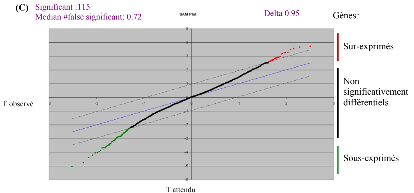
Figure 22. Recherche de gènes différentiellement exprimés, exemple de l'outil SAM pour Excel® (Tusher et al. , 2001)
