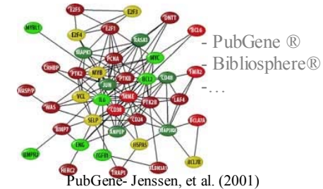
Figure 43. Exemples d'analyses et d'outils disponibles pour l'extraction des connaissances des données de puces à ADN.
