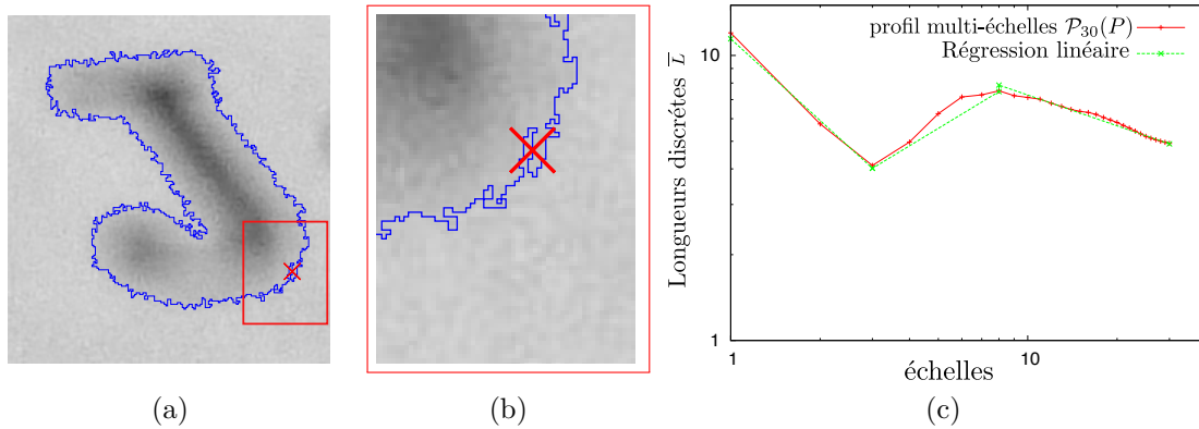
Fig. 3.10 – Illustration de l'échelle standard sur une forme fortement bruitée. L'échelle standard du point représenté par une croix rouge est (8, 30) .
