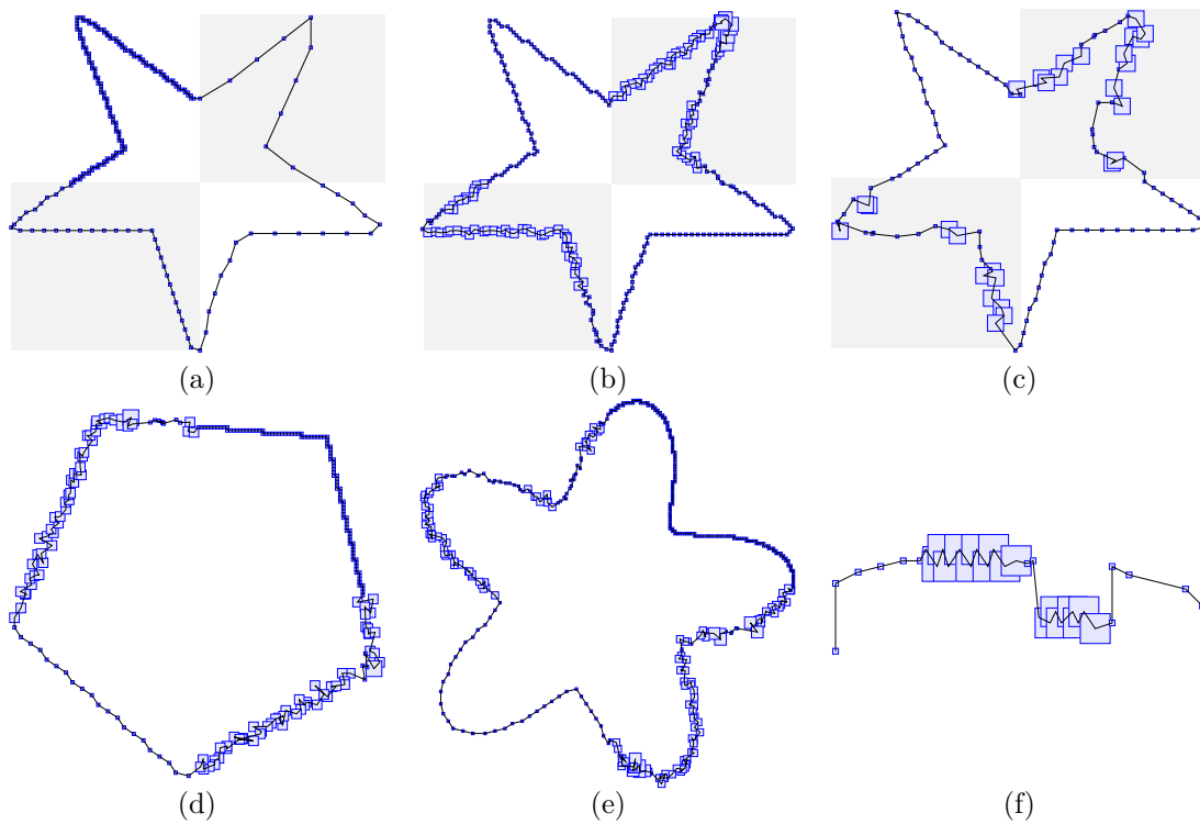
Fig. 3.19 – Résultats de l'épaisseur significative obtenue sur les formes de la figure Fig. 3.15 (première ligne) et résultats sur d'autres contours dont un sur un contour ouvert (image (f)).
