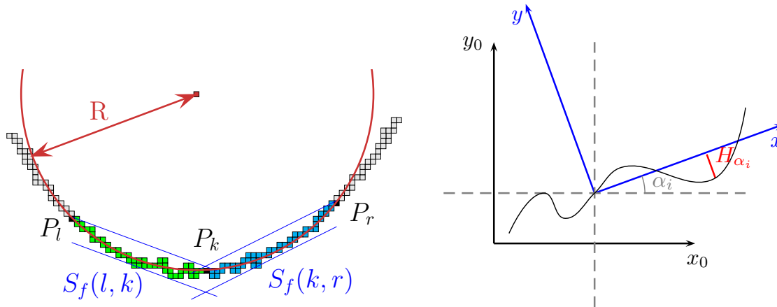
Fig. 4.1 – À gauche : illustration du calcul de la courbure basé sur la méthode du cercle osculateur. Les deux demi-tangentes sont calculées à partir du point P_k à travers un segment flou d'épaisseur 4. À droite : illustration de la notion de visual curvature .
