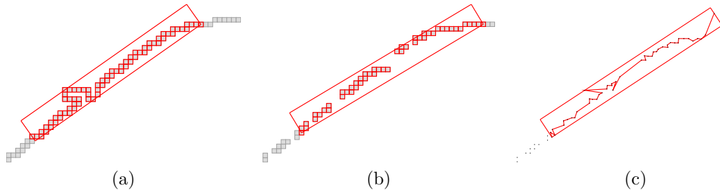
Fig. 1.4 – Exemple de segments flous définis sur différents types de support : (a) sur une séquence de points discrets avec coordonnées non forcément croissante, (b) sur une séquence déconnectée, (c) sur un contour à coordonnées non forcément entières.
