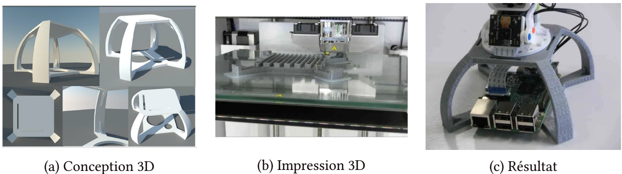
FIGURE 2.3 – Socle alternatif pour ErgoJr, réalisation élèves de Mr C Casseau [13]
