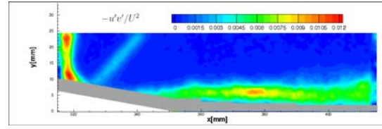
(d) u'v' : z = -14 mm.
