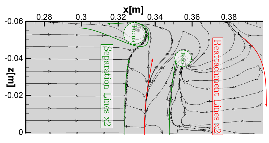
(c) ZDES.
