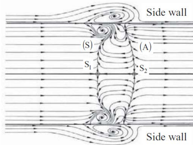
Figure A.3: Topologie 3D des lignes de frottements d'une interaction onde de choc / couche limite dans une veine rectangulaire, issu de Babinsky and Harvey [6].
