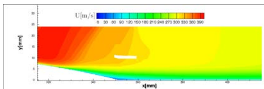
(k) U: z = -26 mm.
