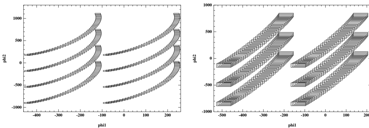
Figure 5.9 Faisceaux optimaux pour PX=2 et PX=8
