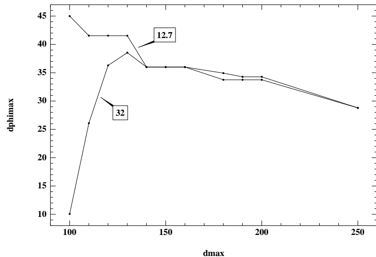
Figure 3.9 Influence sur \delta\phi de la distance minimale entre deux antennes
