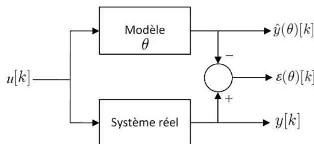
FIGURE 4.2 – Erreur de sortie
