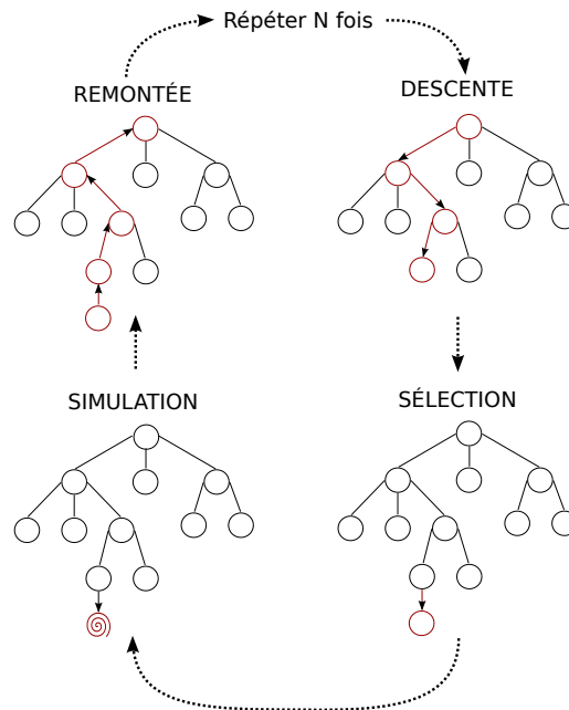
FIGURE 5.1 – Étapes de l’algorithme UCT.
