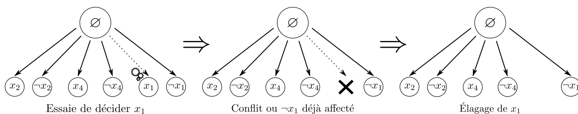
FIGURE 5.5 – Conflit ou littéral déjà affecté à une valeur opposée lors de la descente dans UCTSAT.
