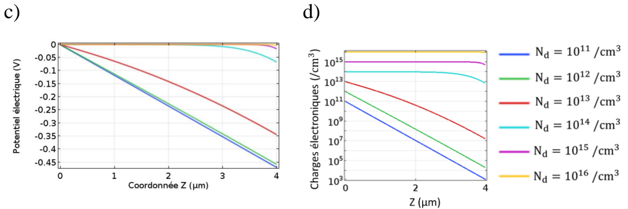
Figure 4-69: Résultats de simulation FEM obtenus en fonction du dopage du NF : a) répartition du champ électrique le long du NF non dopé; b) répartition du champ électrique le long du NF à différents niveaux de dopage; c) répartition du potentiel piézoélectrique ; d) répartition des charges électroniques.
