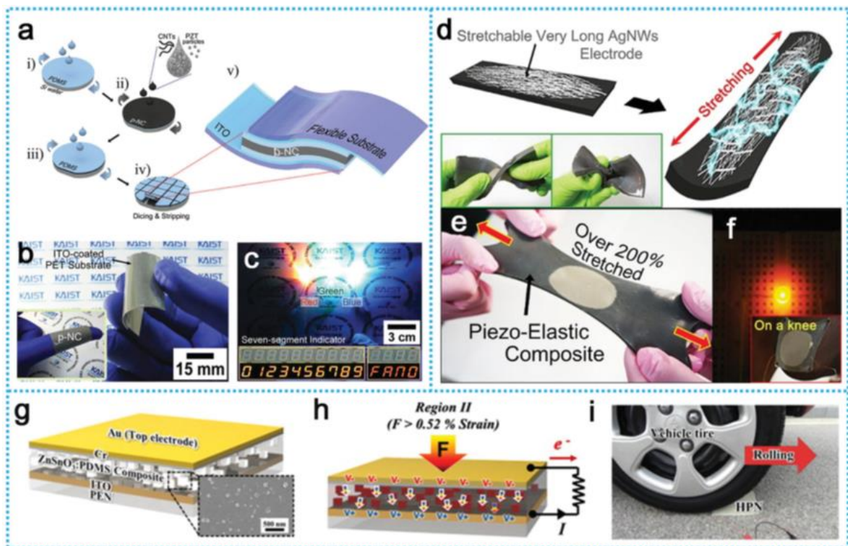
Figure 3-38: Etat de l'art de différents nano-composites (NCG). a-c) Les NCG à base de nanoparticules de PZT [37]. d-f) Les NCG à base de nanoparticules de PMN-PT [58]. g-i) Les NCG à base de ZnSnO_3 . [57]
