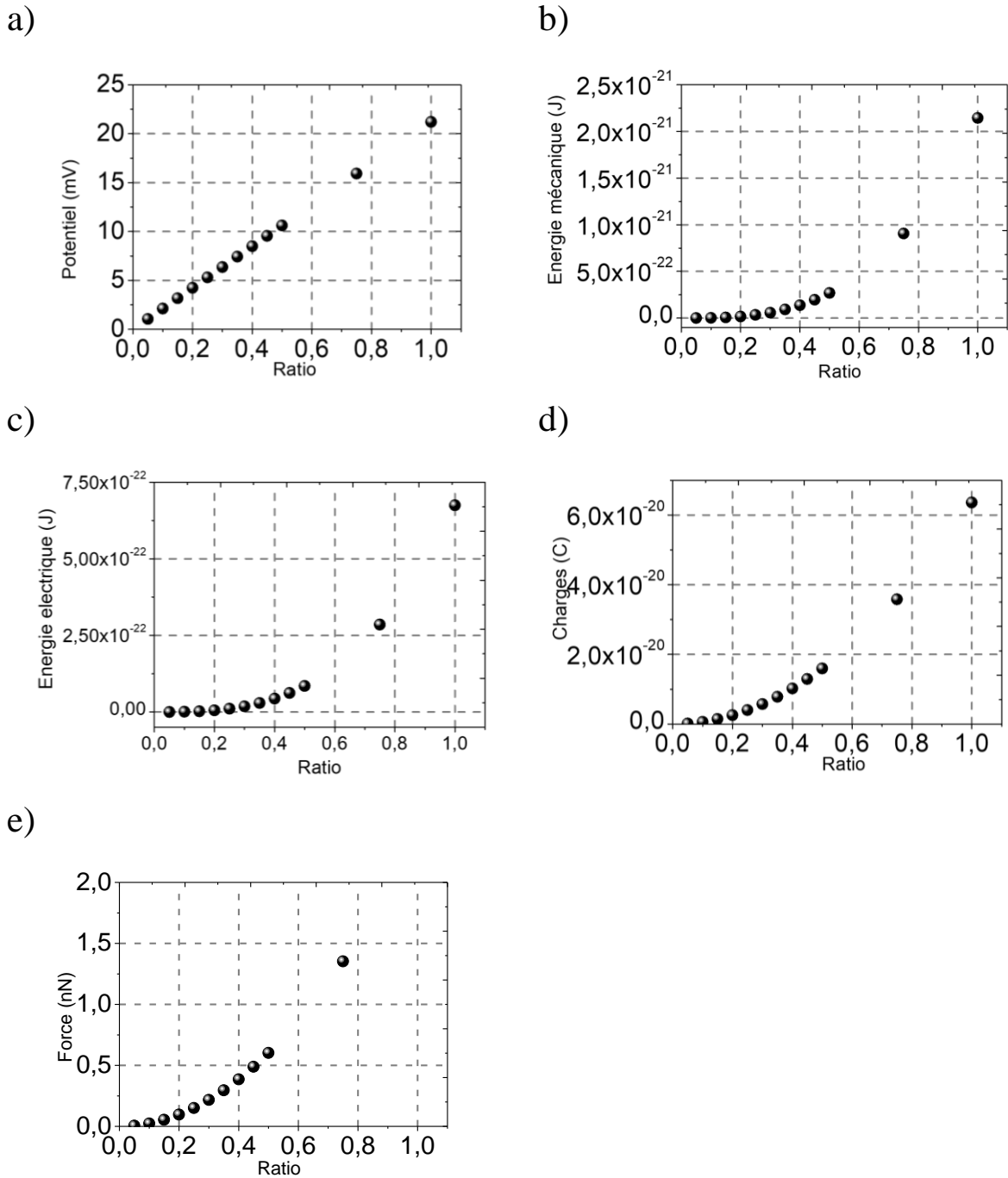
Figure 4-59: Variation des grandeurs électriques et mécaniques du NF en fonction du ratio diamètre supérieur sur diamètre inférieur : a) potentiel électrique, b) énergie mécanique, c) énergie électrique, d) charge électrique, e) force appliquée au NF.
