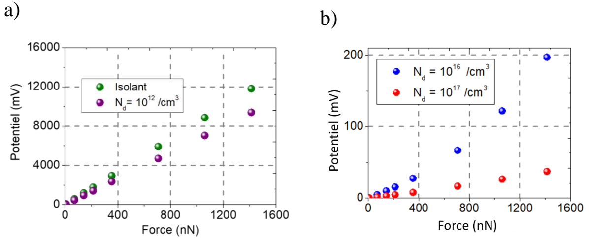
Figure 4-73: Effet de la variation de la force sur le potentiel électrique généré, pour différents niveaux de dopage. a) Cas isolant et d'un faible niveau de dopage. b) Cas d'un fort niveau de dopage.
