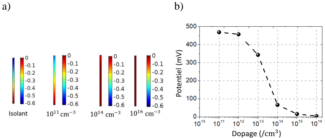
Figure 4-68: Les résultats correspondant à l'étude en fonction du dopage du dopage du NF. a) la répartition du potentiel obtenu, b) le potentiel récupéré au sommet du NF en fonction de la variation du niveau de dopage.
