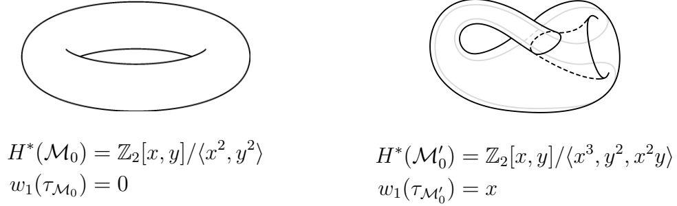
Figure I.10: Les anneaux de cohomologie de \mathcal{M}_0 et \mathcal{M}'_0 sur \mathbb{Z}_2 , et les premières classes de Stiefel-Whitney de leurs fibrés tangents respectifs \tau_{\mathcal{M}_0} et \tau_{\mathcal{M}'_0} .
