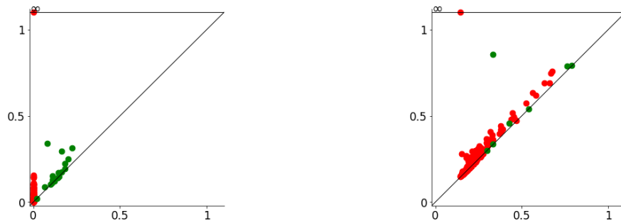
Figure I.3: Gauche : Diagramme de persistance de la filtration de Čech V[X] . Droite : Diagramme de persistance de la filtration-DTM W[X, m, 1] .
