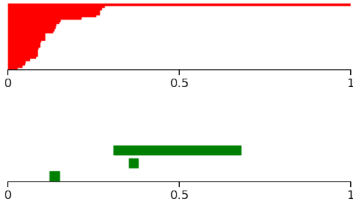
Un code-barres de persistance
