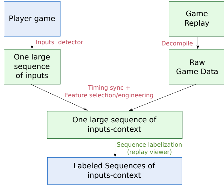
Рис. 6.3: Data augmentation
