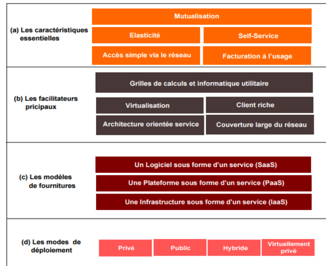
Figure 35 : Aperçu général du Cloud.
