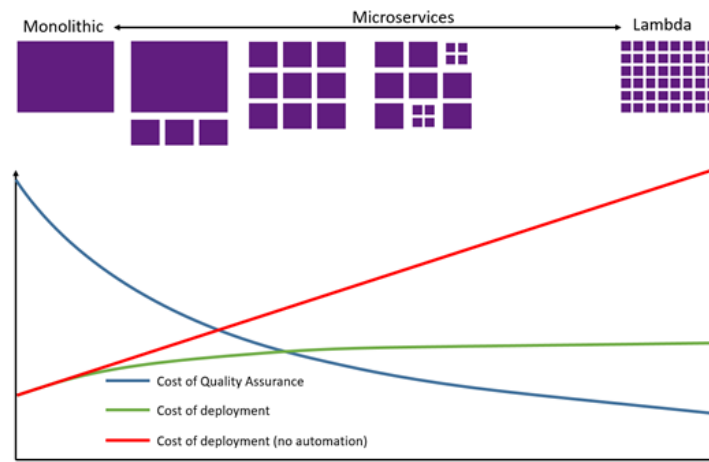
Figure 52 : Détermination de la granularité des services en fonction des coûts.
