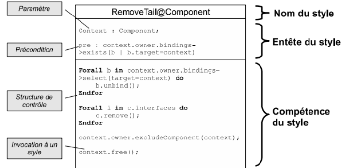
Figure 14 : Nom, entête et compétence d'un style d'évolution.
