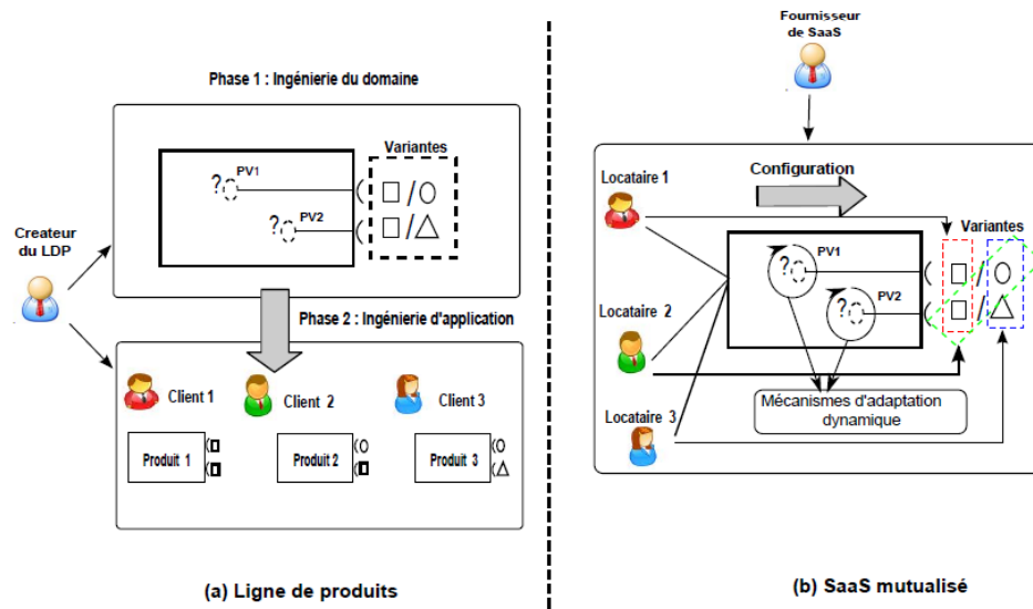
Figure 47 : La variabilité dans les LDP Vs. la variabilité dans les applications SaaS mutualisées
