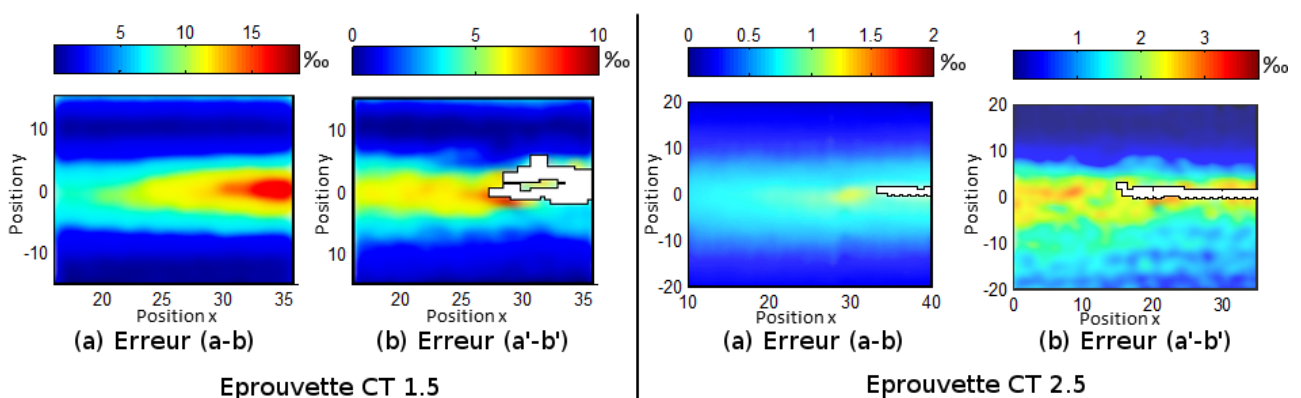
Fig. 2.14 – Écart à la linéarité sur u_x lors des phases de rechargement
