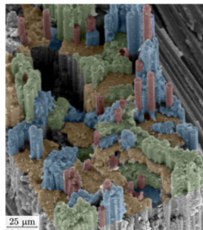
(c) Profil de rupture d'un stratifié 0-90 carbone-epoxy [Pimenta and Pinho, 2014]
