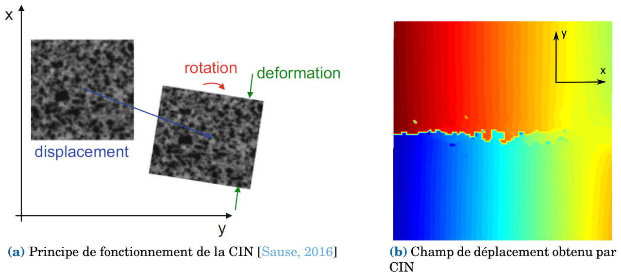
Fig. 1.3 – Principe et mise en place de la CIN
