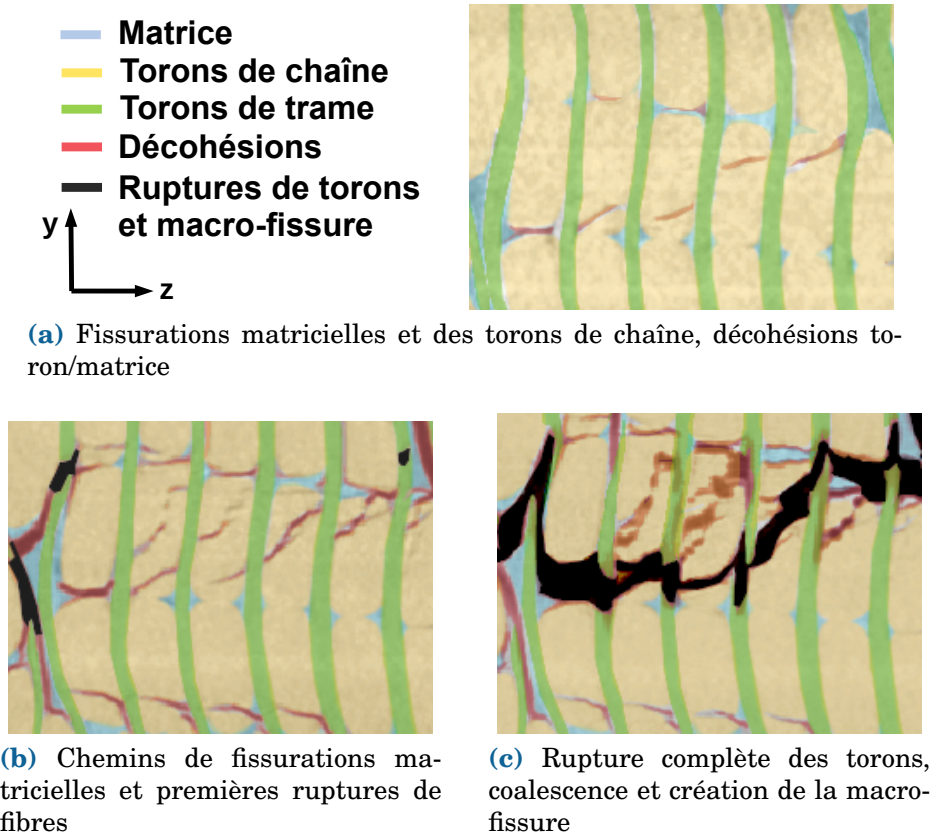
Fig. 2.17 – Scénario de rupture des composites tissés 3D obtenu par \mu -tomographie sur éprouvette CT
