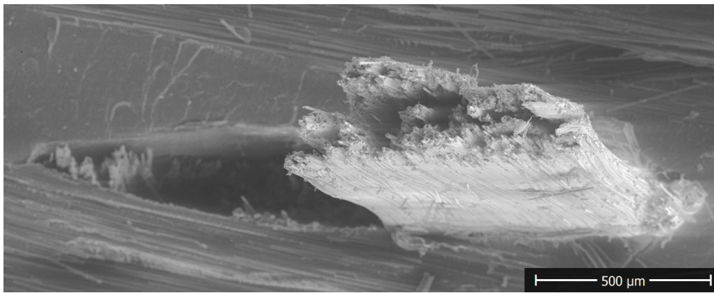
(a) Vue MEB d'un toron rompu sur composite tissé 3D
