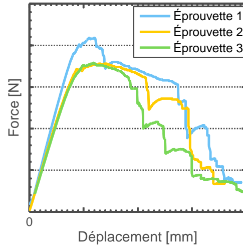
Fig. 1.40 – Courbes Force / Déplacement obtenues sur composite tissé 3D avec RCT équilibré
