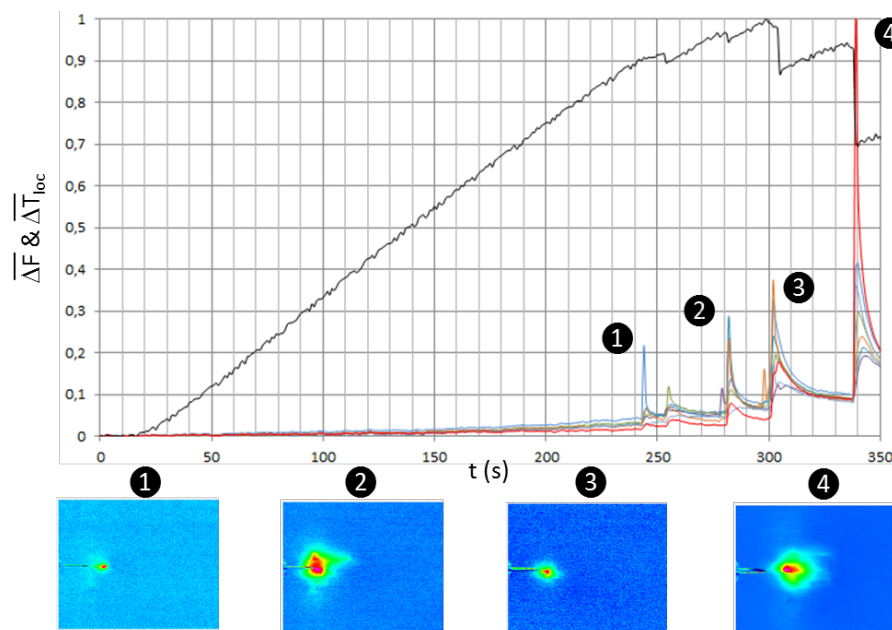
Fig. 1.22 - Évolution de l'échauffement en cours d'essai et comparaison avec la courbe force/déplacement
