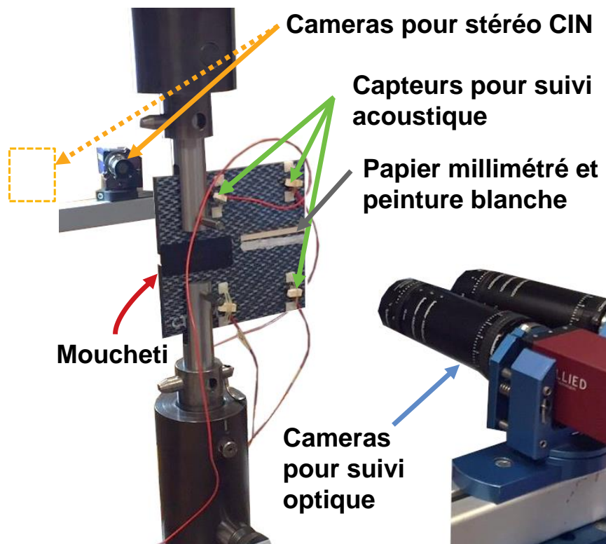
Fig. 1.13 – Mise en place des essais CT et des techniques d'instrumentation associées
