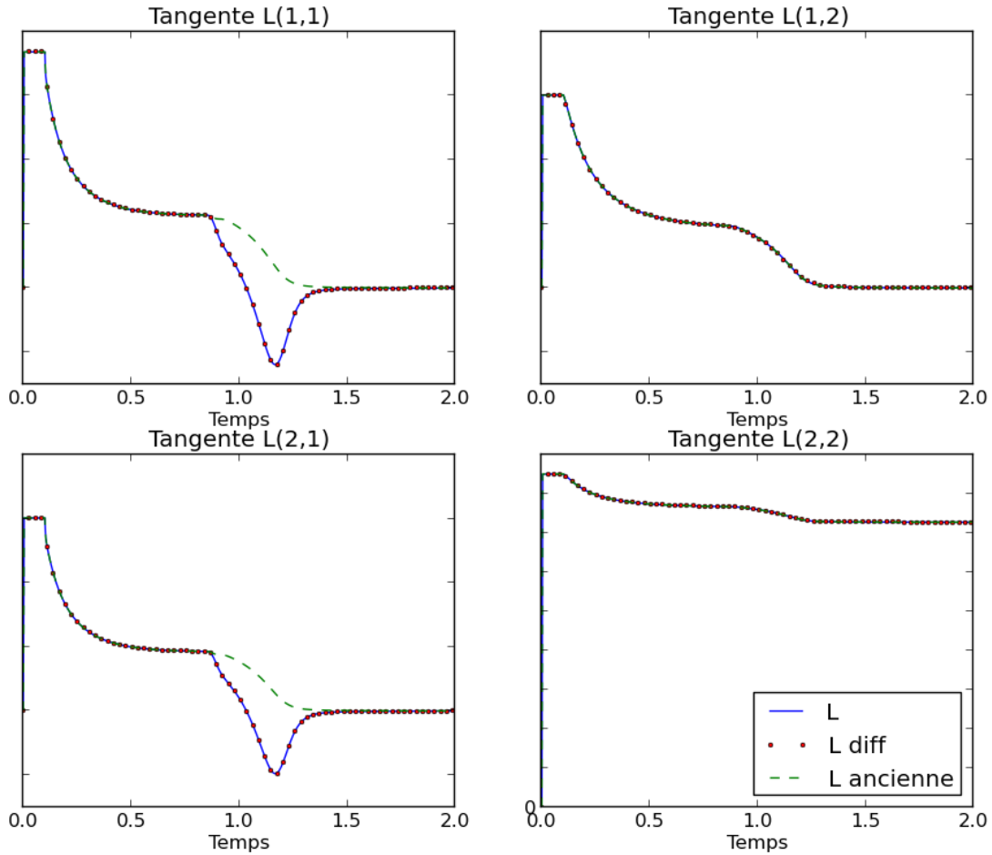
Fig. B.2 – Comparaison des tangentes calculées et par différences pour une régularisation par taux limité
