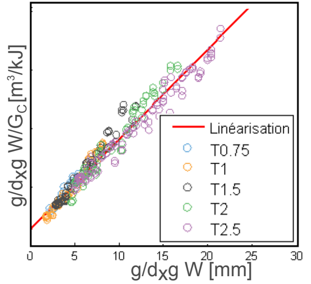
Fig. 2.24 – Identification des paramètres de rupture sur CT par linéarisation (Éq. 2.57)
