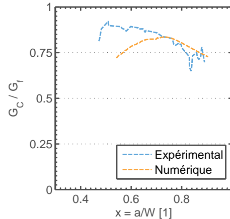
Fig. 3.30 - Comparaison de la forme des courbes \mathcal{R} expérimentales et obtenues numériquement sur éprouvettes CT
