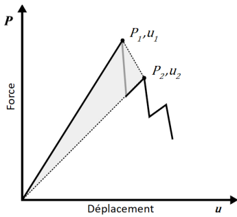
Fig. 1.2 - Interprétation graphique de la méthode des aires [Laffan et al., 2010a]
