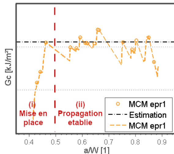
Fig. 1.33 – MCM appliquée en tout point sur CT T1.5
