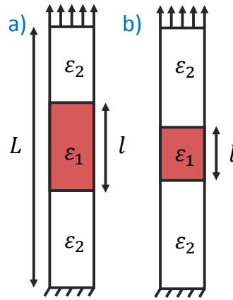
Fig. 3.3 - Perte d'unicité globale sur une barre
