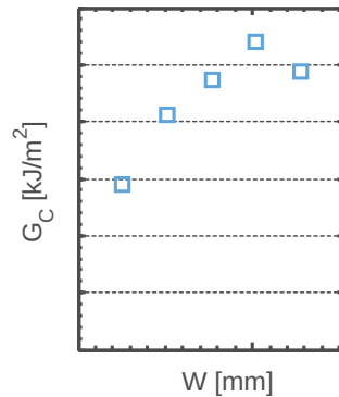
Fig. 3.24 - Évolution de G_C sur un modèle Non Local avec endommagement retardé
