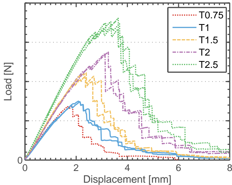
Fig. 1.29 – Courbe force/déplacement sur essais CT RCT1 pour différentes tailles homothétiques d'éprouvettes
