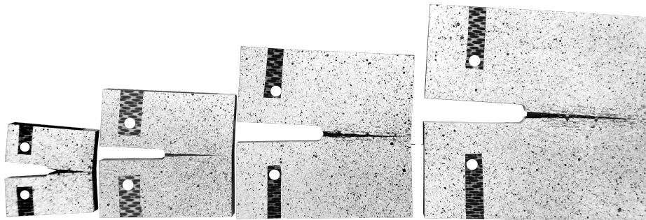
Fig. 1.12 – Éprouvettes CT homothétiques après rupture : Tailles 1, 1.5, 2 et 2.5
