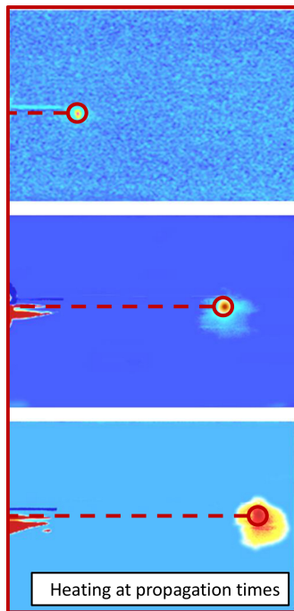
Fig. 1.23 – Mise en place du suivi de la fissure par thermographie infrarouge passive
