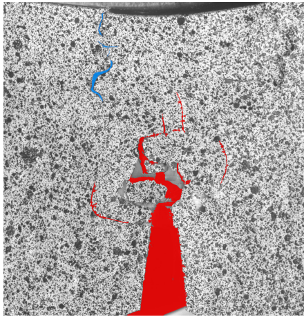
Fig. 1.39 – Profil de fissure sur composite tissé 3D sur RCT4 équilibré. Rouge : macro-fissure en traction, Bleu : rupture en compression
