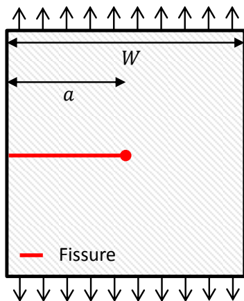
Fig. 2.2 - Fissure en MLER
