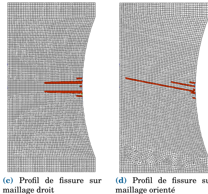
Fig. 3.16 – Résultats de simulations numériques sur le modèle non-régularisé sur éprouvette Diabolo
