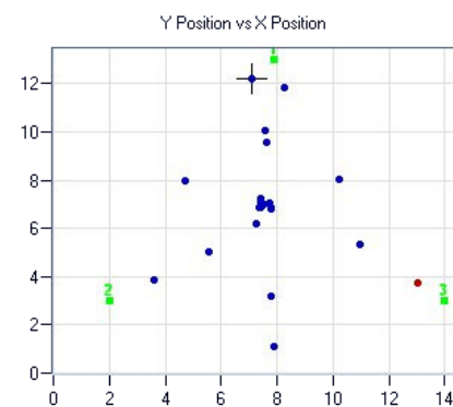
(b) Localisation d'évènements acoustiques [Mistras, 2011]
