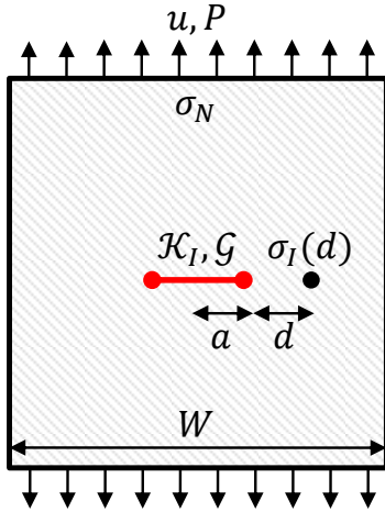
Fig. 2.1 - Exemple de structure et quantités mécaniques associées
