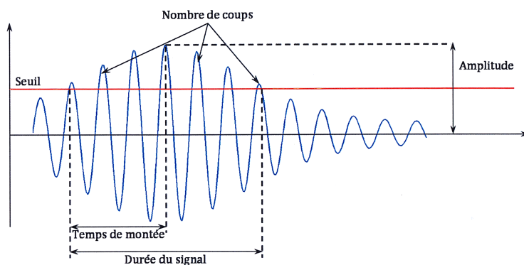
(a) Critère de description de l'onde [Hurmane et al., 2016]
