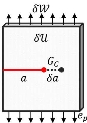
Fig. 1.1 - Schéma de propagation de fissure en théorie de Griffith
