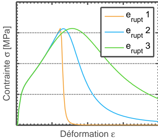
Fig. 3.31 - Variation des courbes Contraincte/Déformation avec e_{rupt} sur RCT1
