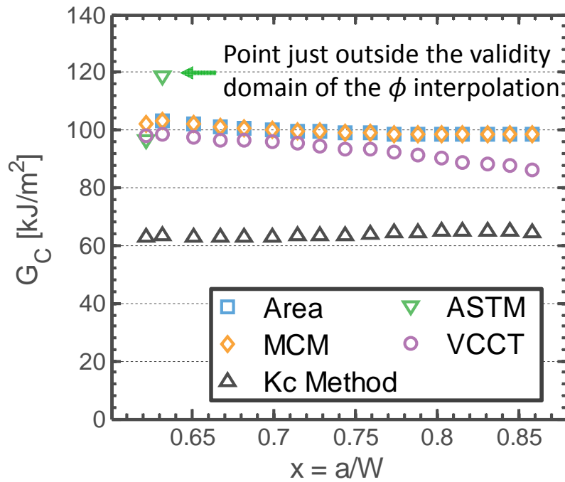
Fig. 1.28 – Application des méthodes d’estimation de G_C sur un cas test numérique utilisant des zones cohésives avec une valeur arbitraire de G_C = 100 \text{ kJ/m}^2
