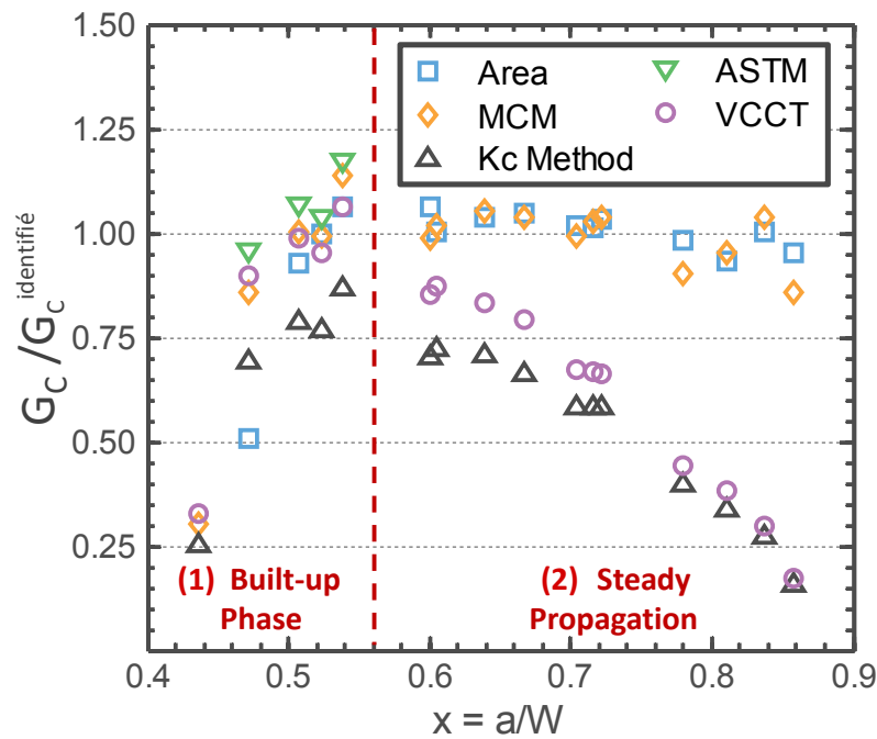
Fig. 1.27 - Évolution de G_C obtenue par les différentes méthodes d'estimation
