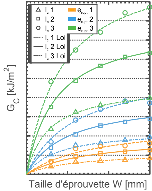
Fig. 3.32 - Variation de G_C avec e_{rupt} , l_c et W et identifications de l'Éq. 3.69
