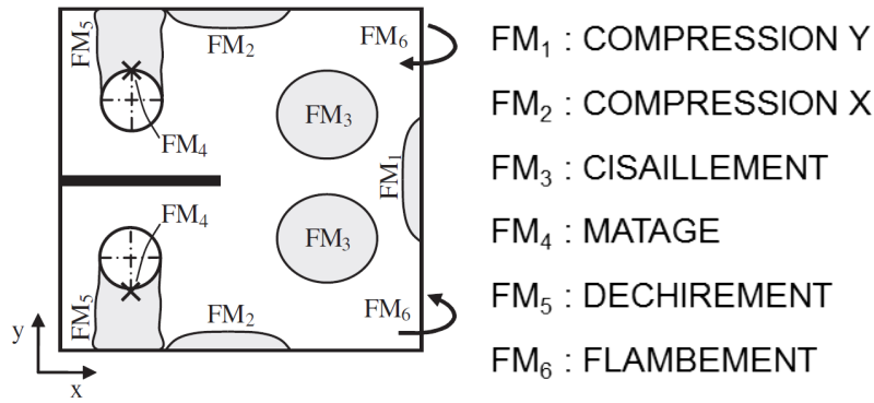
Fig. 1.9 – Modes de ruine des éprouvettes CT tels que proposé par Blanco [Blanco et al., 2014]
