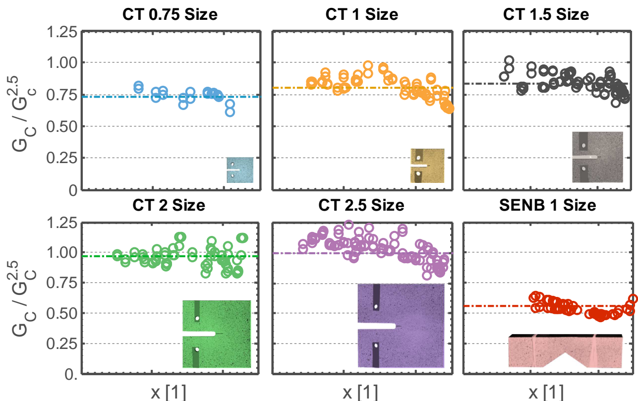
Fig. 1.35 – Valeurs plateau des courbes de résistance sur essais CT et SENB
