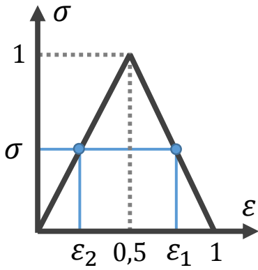
Fig. 3.2 - Perte d'unicité locale sur un problème adoucissant
