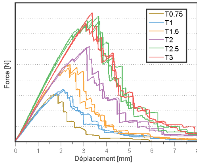
Fig. 1.38 – Courbes Force/Déplacement obtenues pour un facteur d'échelle T3 et comparaison avec les courbes précédentes
