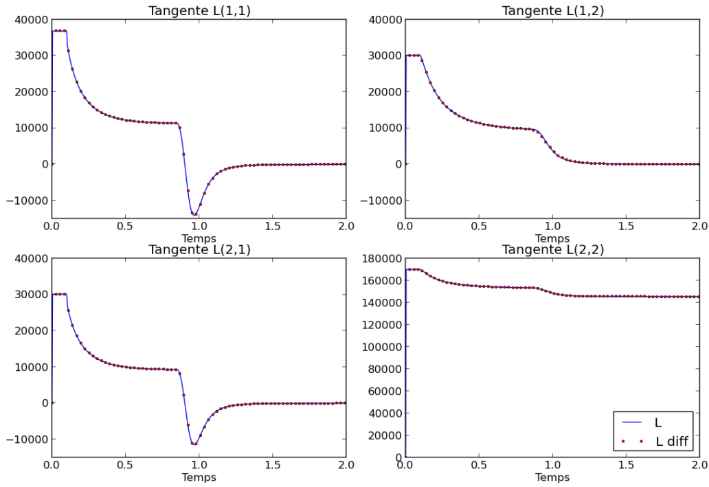
Fig. 3.13 – Comparaison des tangentes calculées et par différences sur le modèle simplifié non-régularisé
