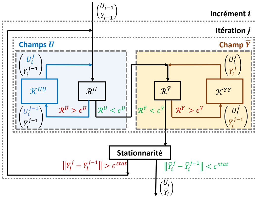
Fig. C.2 - Résolution alternée des modèles non-locaux
