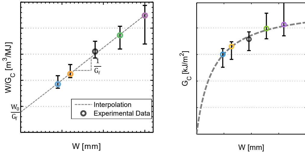
(a) Interpolation linéaire sur données expérimentales CT (Éq. 2.49)
