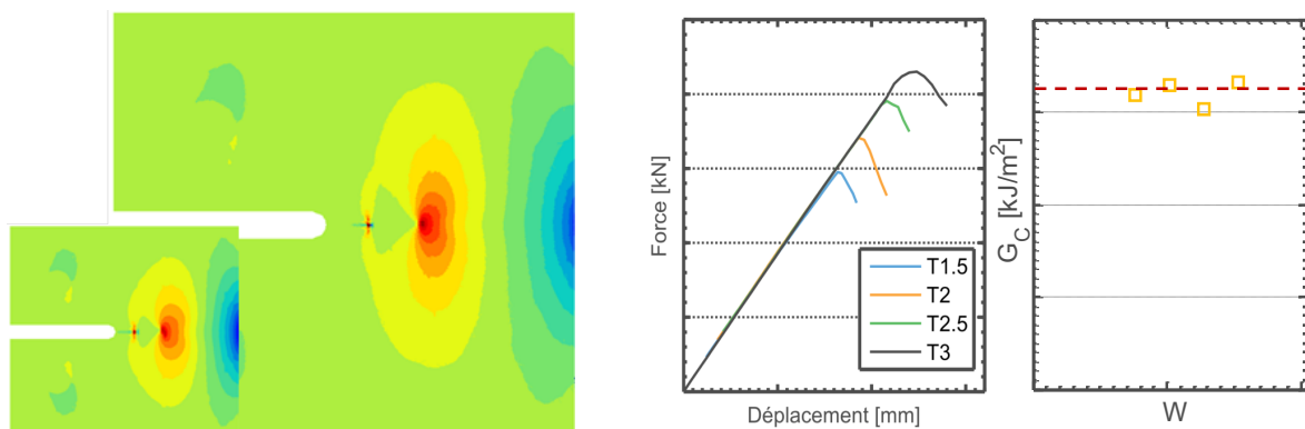
(a) Forme des champs de contraintes sur éprouvettes homothétiques de taille 1 et 2
