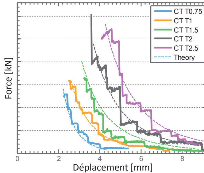
Fig. 2.26 – Comparaison des courbes forces déplacement expérimentales et du modèle (Éq. 2.64 et 2.64)
