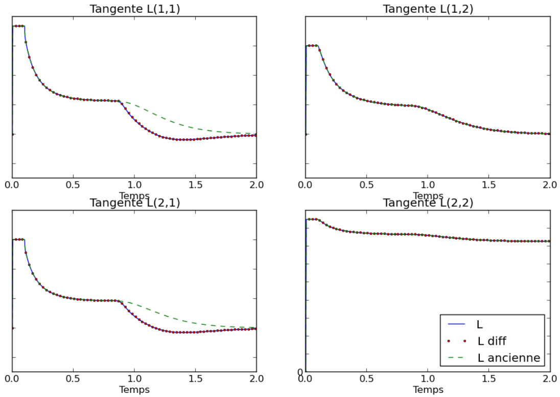
Fig. B.1 – Comparaison des tangentes calculées et par différences pour une régularisation par effet retard
