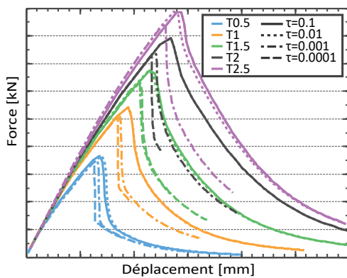
Fig. 3.23 - Courbes Force / Déplacement sur un modèle Non Local avec endommagement retardé
