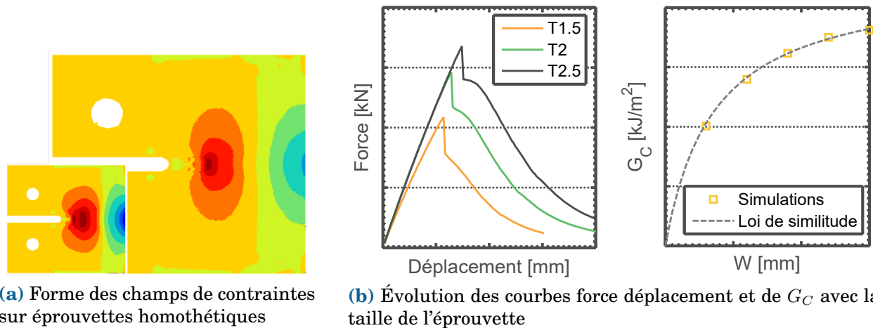
Fig. 3.22 - Effet d'échelle numérique obtenu avec un modèle Non-Local
