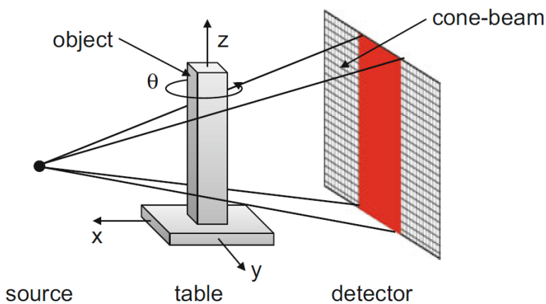
(a) Principe de la tomographie par rayons-X [Sause, 2016]
