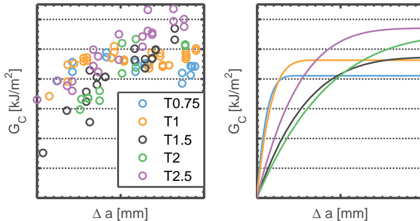
Fig. 1.34 - Valeurs plateau des courbes de résistance sur essais CT
