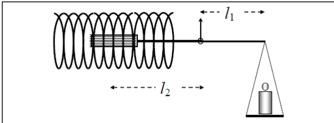
Figure 7: Schéma de l'électrodynamomètre de Pellat
