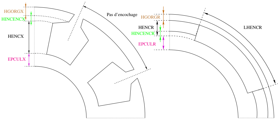
3.1.2: Stator ou rotor bobiné interne
