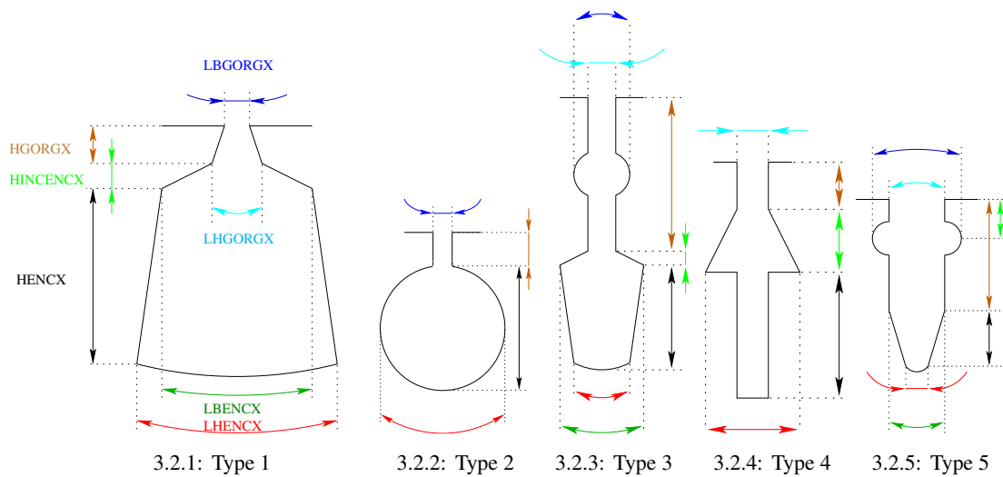
FIG. 3.2 – Exemples de géométries d'encoches possibles en utilisant le jeu de paramètres proposés.
