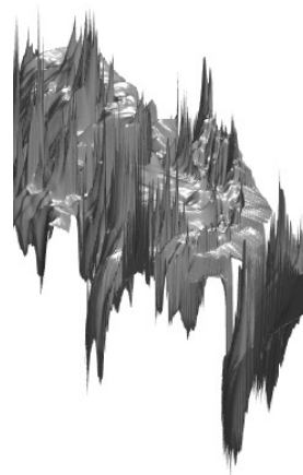
Algorithme du point fixe (sans régularisation) [127].
