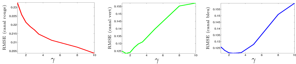
FIGURE 4.8 – Étude quantitative de l'influence du paramètre \gamma menée sur le même jeu de données que celui de la figure 4.5, avec \varrho = 1000 .
