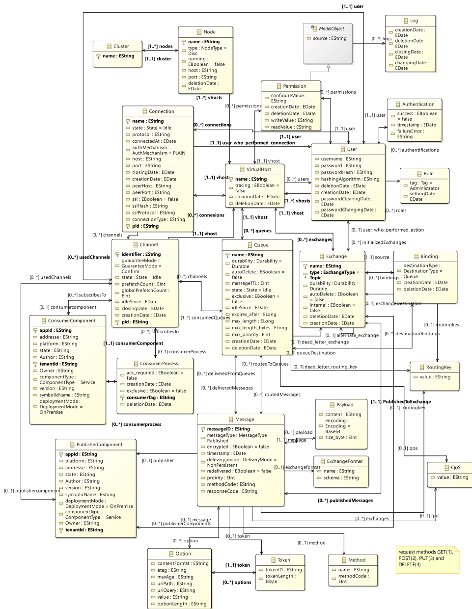
FIGURE 3.3 – Le Métamodèle Pulse
