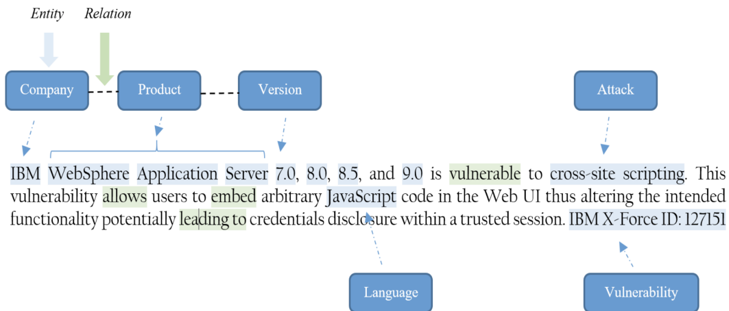
FIGURE 3.8 – Principe de la reconnaissance d’entités nommées et de l’extraction de relations
