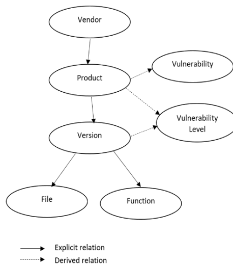
FIGURE 3.10 – Ontologie utilisée pour identifier les vulnérabilités
