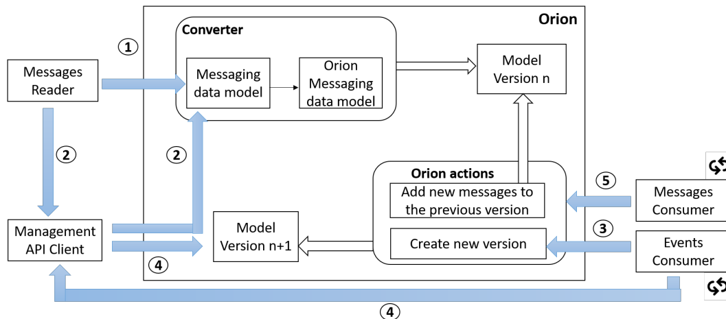
FIGURE 3.2 – Processus de gestion de version avec Pulse
