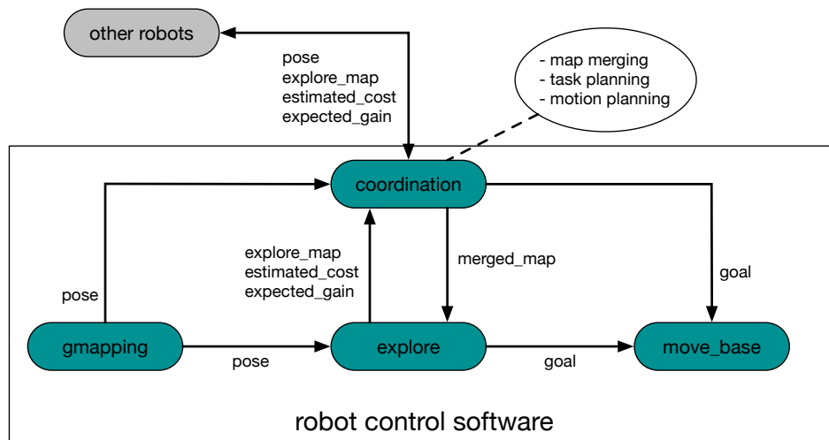
FIGURE 4.3 – Architecture logicielle d'un robot
