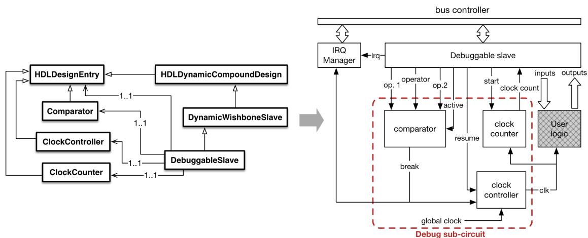
FIGURE 4.7 – Exemple d'un circuit généré
