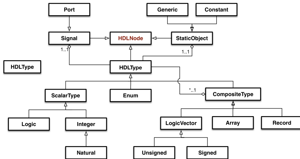
FIGURE 4.6 – Métamodèle OoRC
