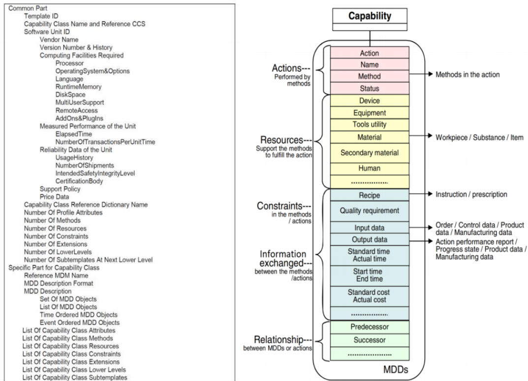
FIGURE 2.6 – Profil de Capacité de l'ISO 16100
