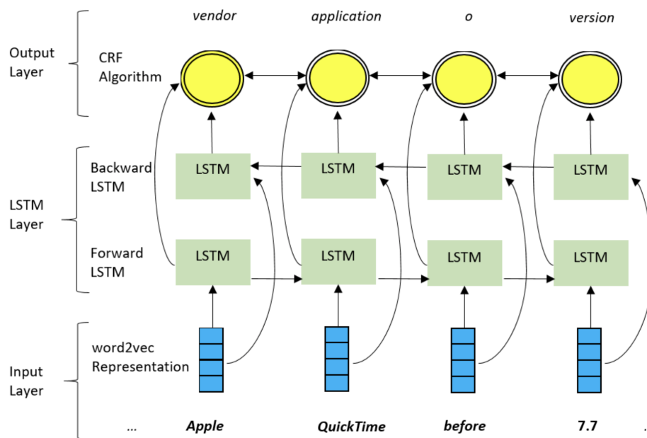
FIGURE 3.11 – Fonctionnement de l'architecture LSTM-CRF
