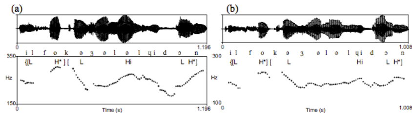
Figure I.A.5. Contour de f_0 pour la phrase 'Il faut que je le lui donne' contenant 4 clitics, produite par les loc. 4F (a) et 3F (b).
