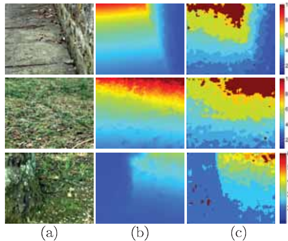
FIGURE 3.6 – Reconstructions de cartes de profondeur par DBNs : (a) image couleur, (b) carte de profondeur stéréo (référence), (c) DBNs parcimonieux. Source [CN-4]
