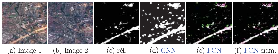
FIGURE 2.14 – Jeu de données OSCD (extrait sur Montpellier) et détection de changements par réseaux convolutifs, en utilisant les 13 canaux des images Sentinelle 2. (d) CNN ; (e) FCN avec concaténation des images en entrée ; (f) FCN siamois. Dans les images (e) et (f), blanc indique les vrais positifs, noir les vrais négatifs, vert les faux positifs, et magenta les faux négatifs. Source : [CI-38, CI-42].
