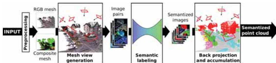
FIGURE 3.11 – Algorithme SnapNet : génération de vues virtuelles à partir du nuage de points, segmentation sémantique en 3D, re-projection en 3D pour classification du nuage de points. Source : [RI-10].
