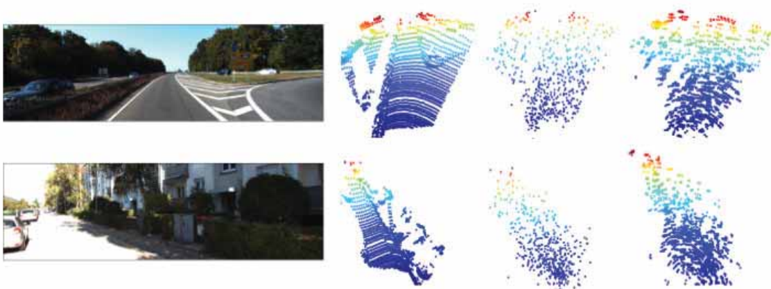
FIGURE 4.6 – Prédiction de nuages de points 3D avec une seule image : image originale RGB du jeu KITTI [228] pour la conduite autonome, nuage de points LiDAR correspondant, prédiction du nuage squelette par réseaux de neurones et transport optimal, densification par réseaux de neurones. Source : [229].
