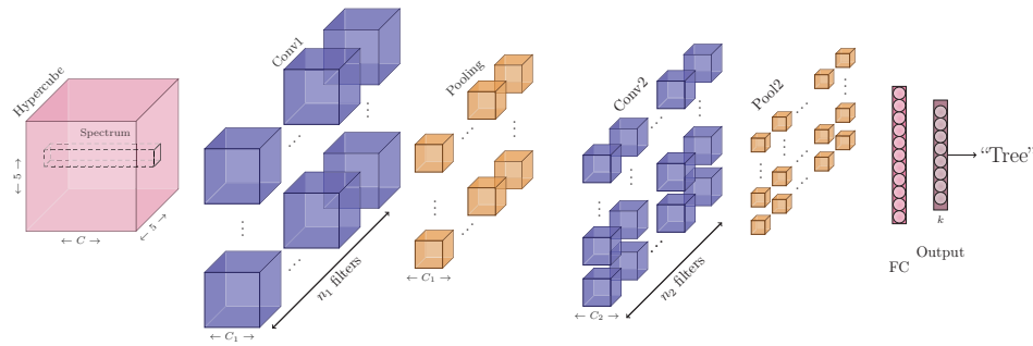
FIGURE 2.13 – Réseau de neurones 3D pour la classification de données hyperspectrales disponible dans DeepHyperX . Il reproduit l’architecture proposée dans [140] et alterne convolutions 3D et couches de max-pooling 3D. Source : [RI-16].
