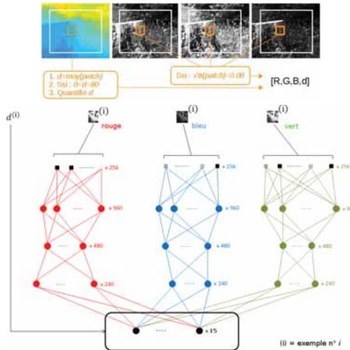
FIGURE 3.5 – Schéma de sélection de fenêtres ( patch [R, G, B, d] dans un triplet d’images RGB chromatique et la carte de profondeur obtenue par stéréo (en haut) et architecture globale du DBN à 3 canaux avec contrainte de parcimonie pour encoder l’information locale (en bas). Source : [CN-4].
