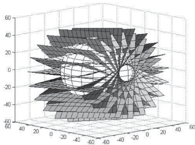
FIGURE 3.1 – Plans de coupe par micro-rotations du microscope confocal dans le repère de la cellule. Des artefacts tels que le "trou noir" autour de l'axe de rotation peuvent apparaître en raison de la dérive de la cellule. Source : [RI-1].
