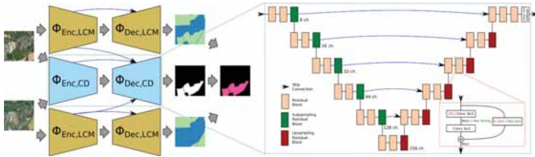
FIGURE 2.15 – Réseau de neurones multitâche pour la détection de changement sémantique. Source : [RI-18].
