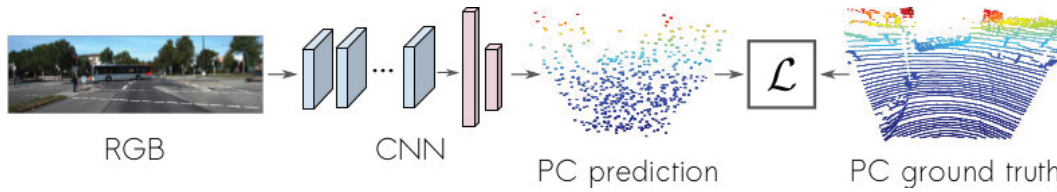
FIGURE 4.5 – Architecture de réseau de neurones pour la prédiction de nuages de points mono-image. Source : [229].
