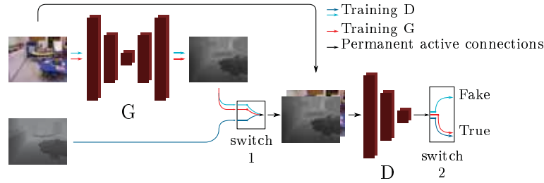
FIGURE 3.8 – D3-Net avec pénalité LS-GAN, où le générateur G est le réseau de la figure 3.7. Source : [CI-41].
