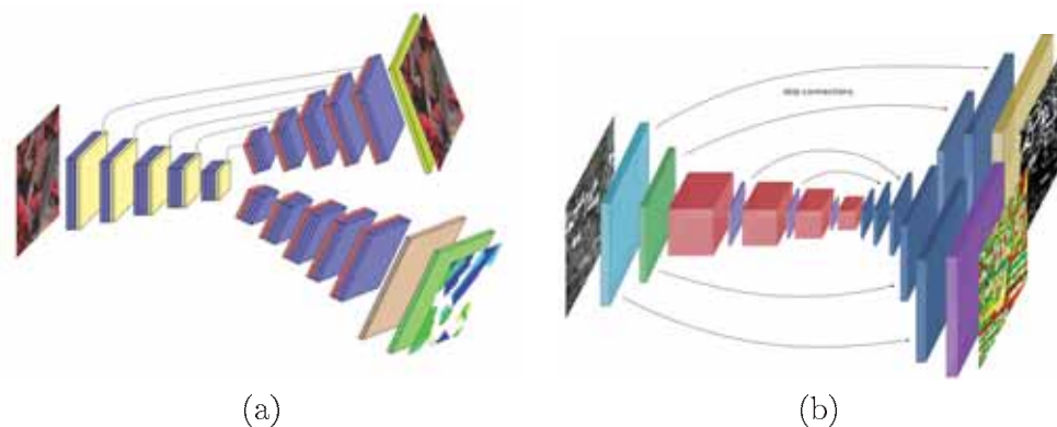
FIGURE 4.2 – Réseaux multitâches pour la compréhension de scènes à large échelle. (a) Architecture semi-supervisée pour la segmentation sémantique large échelle, capable d’apprendre sur des données annotées ou pas. (b) Architecture de modèle d’apprentissage multitâche pour la régression de hauteur et la classification sémantique. Sources : [CN-12, RI-20].
