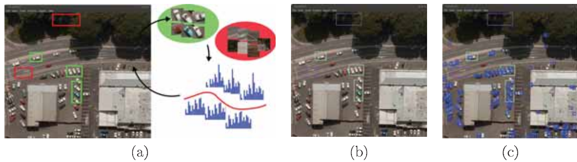
FIGURE 2.2 – Classification interactive d’objets en télédétection. (a) Boucle interactive : sélection d’exemples dans l’image via une interface ergonomique ; extraction de patches et indexation (par HOG-LBP) ; classification des patches de la ou des images entières. Exemple : (b) sélection de zones contenant l’objet recherché (ici, véhicules) ; (c) classification (carrés bleus) des patches de l’image contenant des véhicules. Source : [CI-18].
