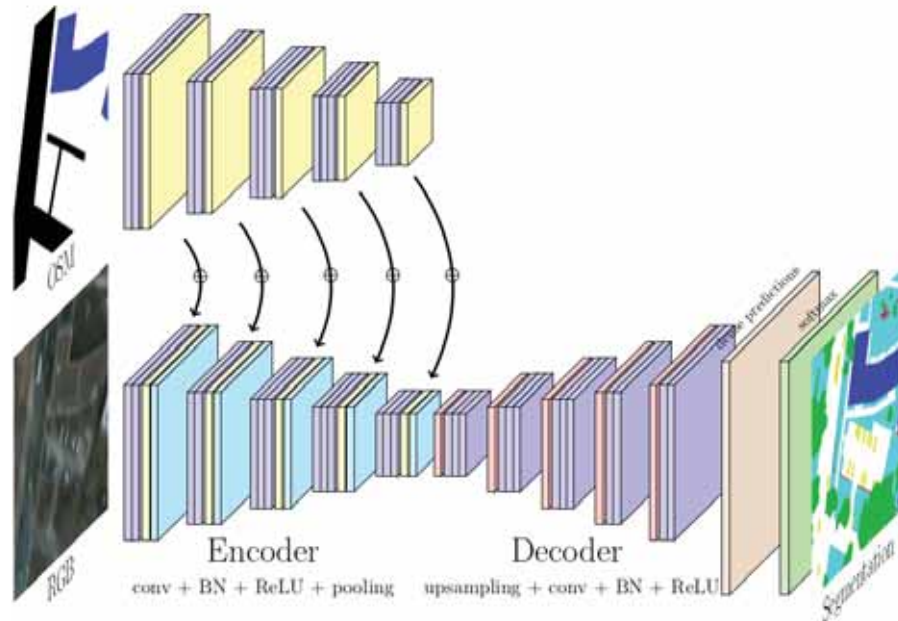
FIGURE 2.10 – Réseau de neurones pour l'apprentissage joint à partir de données fortement hétérogènes. Source : [CI-32].
