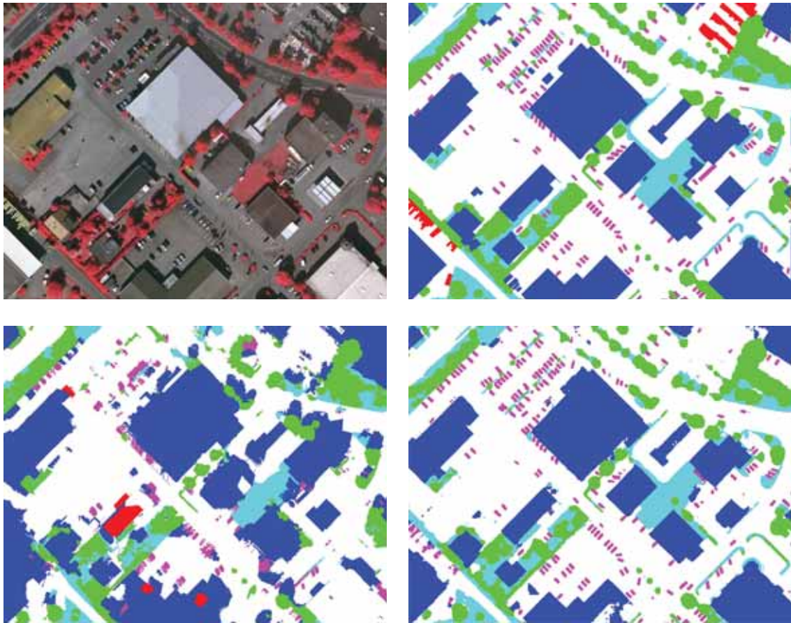
FIGURE 2.6 – Cartographie automatique par réseaux de neurones entièrement convolutifs ((FCNs)) encodeurs-décodeurs SegNet. En haut, image IR/R/G et données de référence associées issues de la base ISPRS Vaihingen. En bas, résultats de l’approche de base (superpixels et CNN [CI-23]) puis segmentation sémantique par SegNet [RI-7]. Source : [RI-7].
