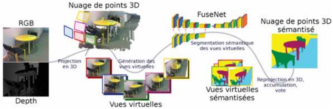
FIGURE 1.12 – Résumé graphique de l’algorithme SnapNet-R(obot) pour la segmentation sémantique de données RGB-D par augmentation de données cohérentes en 3D. Source : [48].
