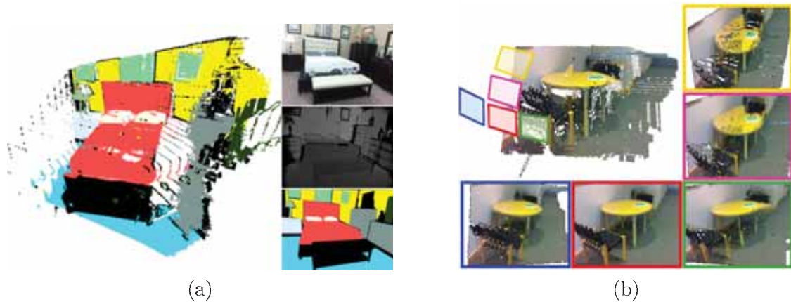
FIGURE 1.11 – [Augmentation de données cohérente avec la 3D pour données RGB-D issues de la base SUNRGBD [49]. (a) Données RGBD monovue comparées aux données 3D équivalentes. (b) Échantillonnage des points de vue pour l'augmentation de données cohérente avec la 3D. Source : [CI-34].
