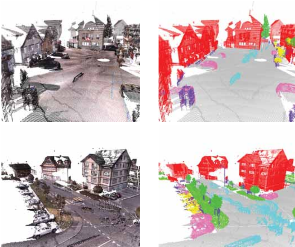
FIGURE 3.13 – Résultats de segmentation sémantique 3D par SnapNet : (gauche) nuage de points 3D colorés (scènes de Semantic3D [193]) et (droite) nuage segmenté selon les classes bâtiment, route, terrain naturel, véhicules, mobilier urbain, végétation haute et basse, artefacts de scan.
