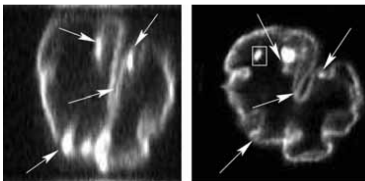
FIGURE 3.3 – Coupes selon le plan xz (l'axe optique est vertical) du volume estimé 3D : à gauche par microscope avec coupes selon l'axe vertical en Z, à droite par microscope avec micro-rotations et reconstruction avec PSF. Source : [RI-1].
