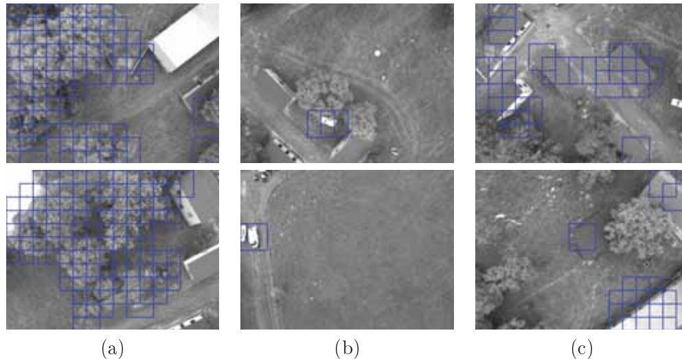
FIGURE 1.10 – Analyse de scène par drone : classification dans la vidéo. Les résultats de détection (carrés bleus) sont obtenus directement dans la vidéo de la caméra embarquée après transformation géométrique. (a) : classification d’arbres ; (b) : classification de véhicules ; (c) : classification de bâtiments. Source : [CI-16].
