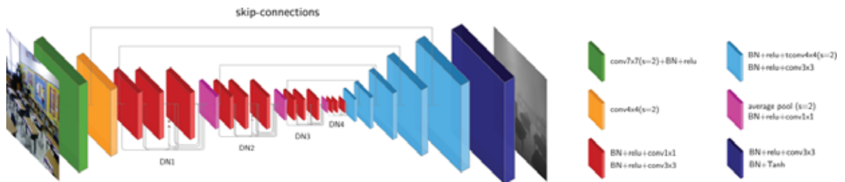
FIGURE 3.7 – Architecture Deep Depth-from-Defocus Network (D3-Net) pour l’estimation de carte de profondeur. Source : [CI-41].
