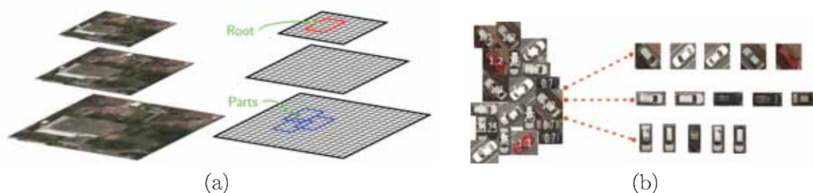
FIGURE 2.4 – Modèles à parties déformables (DPM) en télédétection : (a) modèle multiéchelle avec représentation globale ( racine ) et locale par parties ; (b) catégorisation des exemples selon l’apparence présente dans les DPM et reprise dans les DtMM afin de créer un mélange de modèles. Sources : [CI-17, CI-21].
