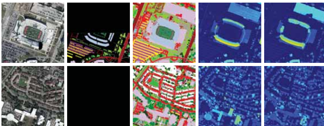
FIGURE 4.4 – Cartographie sémantique et prédiction de la 3D locale par apprentissage multitâche. De gauche à droite, donnée image RGB issue du DFC2018 sur Houston, référence sémantique et prédiction (noir signifie une absence d'information), référence d'élévation et prédiction. Source : [RI-20].
