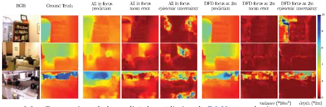
FIGURE 3.9 – Comparaison de la qualité de prédiction de D3-Net sur des images avec et sans flou de défocalisation (plan focal à 2m) : cartes de profondeur, erreur moyenne et incertitude épistémique [188] sur des données NYUv2 [68]. Source [CI-40]
