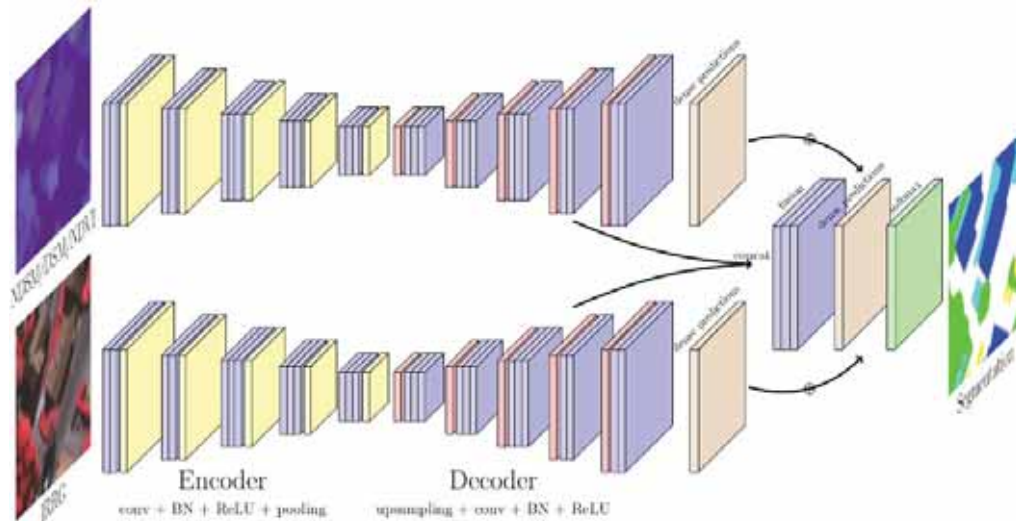
FIGURE 2.8 – Réseau de neurones multimodal avec correction résiduelle. Source : [CI-25].
