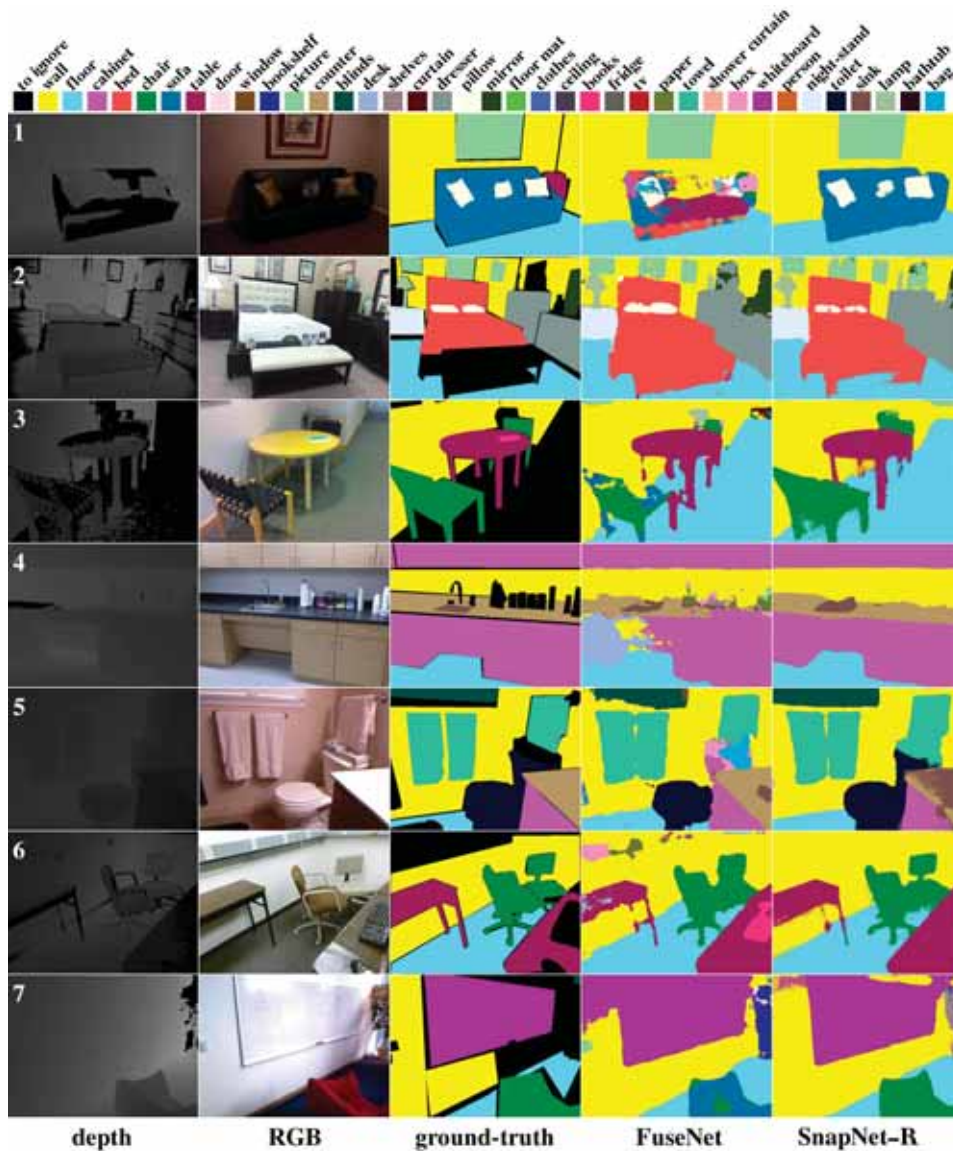
FIGURE 1.13 – Résultats de SnapNet-R pour la segmentation sémantique sur des images de la base SUNRGBD . Source : [CI-34].
