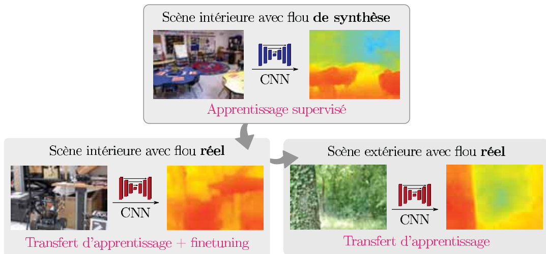
FIGURE 3.10 – Estimation de profondeur sur données floues synthétiques et réelles, en intérieur et extérieur. Les résultats montrent la flexibilité d'adaptation des modèles de Deep-DFD entraînés avec un jeu de données en intérieur avec flou synthétique, adapté par fine-tuning sur des données avec flou réel en intérieur, et finalement testés sur des scènes extérieures réelles sans ré-entraînement. Source [CI-40].
