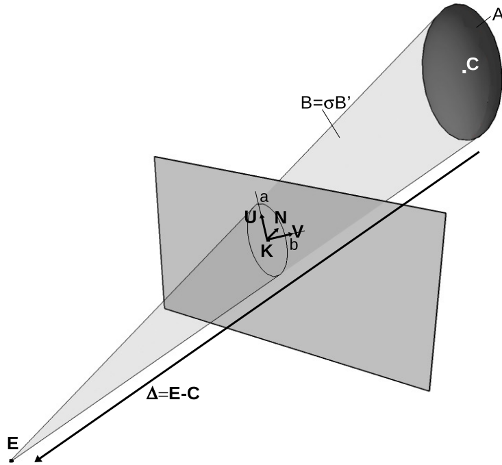
FIGURE 2.5 – Illustration du plan image, du centre de projection, de l'ellipsoïde, et de son ellipse projetée.
