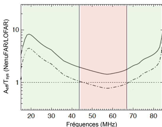
FIGURE 7.6 – Rapport des sensibilité de NenuFAR et du cœur de LOFAR. Le tracé en pointillé représente NenuFAR_1 avec 54 mini-réseaux (mi 2019) et la courbe du dessus en trait plein représente NenuFAR complet avec 96 mini-réseaux (figure modifié de Zarka et al. (2015)).
