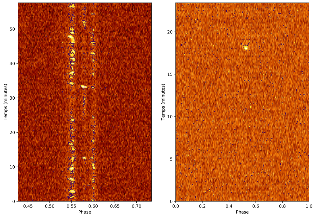
FIGURE 4.3 – Observation de deux pulsars à changement de modes avec NenuFAR. À gauche, B1237+25 où l'on aperçoit une composante centrale apparaît dans un mode puis disparaître dans l'autre (voir dans Backer (1970)). À droite, se trouve B0823+26 pour lequel un des modes est 1000 fois plus intense (visible à 17 minute) que l'autre (pulsar étudié dans Sobey et al. (2015)).
