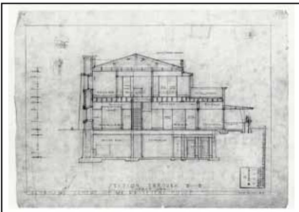
Longitudinal section (1:50)
