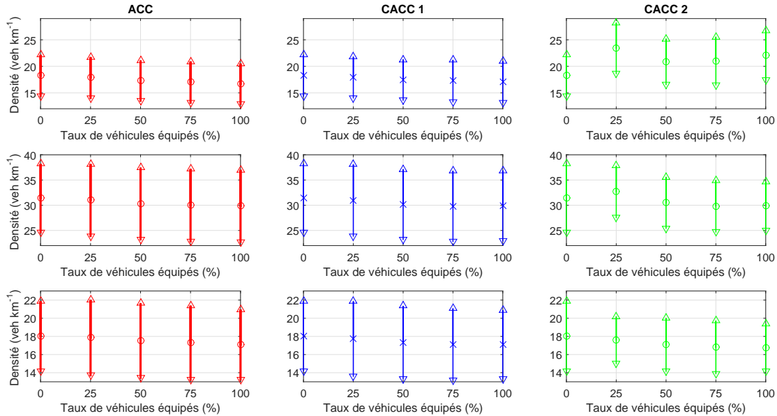
FIGURE 3.42 – Densité de véhicules pour le cas de ralentissement, avec un débit de 1500 veh h -1 d'entrée sur la voie principale, en fonction du taux de véhicules équipés. En amont du ralentissement sur la voie principale en haut, en amont du ralentissement dans la section de ralentissement au milieu et en aval du ralentissement en bas
