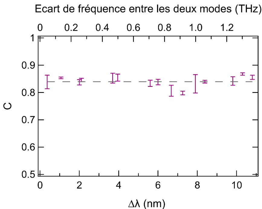
Figure 5.11 : Evolution de la constante de couplage de Lamb mesurée sur un VECSEL à PQs, en fonction de l'écart spectral et fréquentiel entre les deux modes. Les barres d'erreur représentent l'écart type de toutes les valeurs mesurées pour l'écart spectral correspondant. La ligne pointillée grise correspond à C_0 = 0,84 [301].
