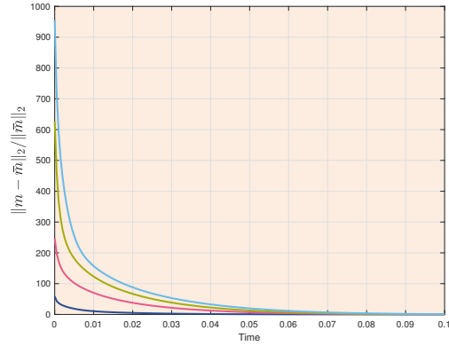
(d) H(x, p) = (\sin(2\pi x_2) + \sin(2\pi x_1) + \cos(4\pi x_1))|p|^3/3 + (1 + \cos(2\pi x_1))|p|^2/2
