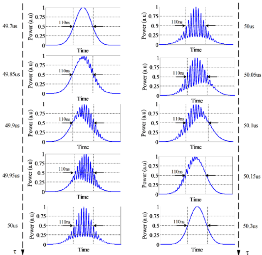
图 4.2 声光斩波器触发信号周期对射频调制脉冲的影响：激光在环形腔内的单次传输时间为 50 \mu\text{s} ，触发周期从 49.7 \mu\text{s} 提高到 50.3 \mu\text{s} ，光纤放大器增益为 6
