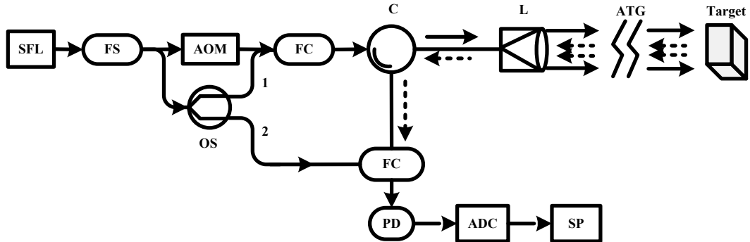
图1.29 大气湍流对激光相干探测影响实验系统框图
