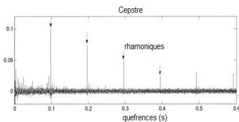
FIGURE 1.7 – la récurrence d'un défaut à 10Hz (roue primaire) est traduite par un peigne de Dirac de fondamental à 100 ms
