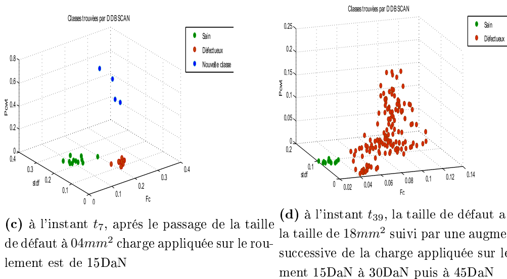
FIGURE 5.25 – Classifications des observations reçues des roulements en différents états et sous charge variable
