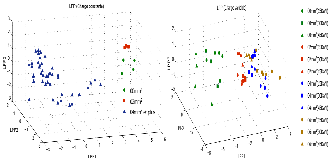
(a) L'application de LPP sur des données ex-traits de roulements sains et défectueux sous la même charge (b) L'application de LPP sur des données ex-traits de roulements sains et défectueux sous différentes charges
