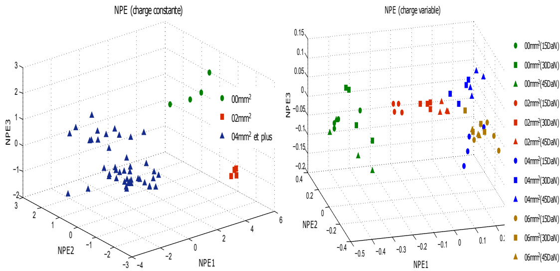
(a) L'application de NPE sur des données ex-traits sur des roulements sain et défectueux sous la même charge (b) L'application de NPE sur des données ex-traits sur des roulements sain et défectueux sous différentes charges
