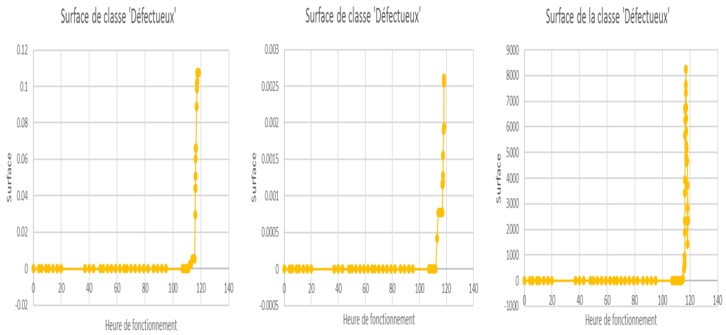
(a) La surface de la classe 'Défectueuse' par DFSDBSCAN (b) La surface de la classe 'Défectueuse' par ESDBSCAN (c) La surface de la classe 'Défectueuse' par DDBSCAN
