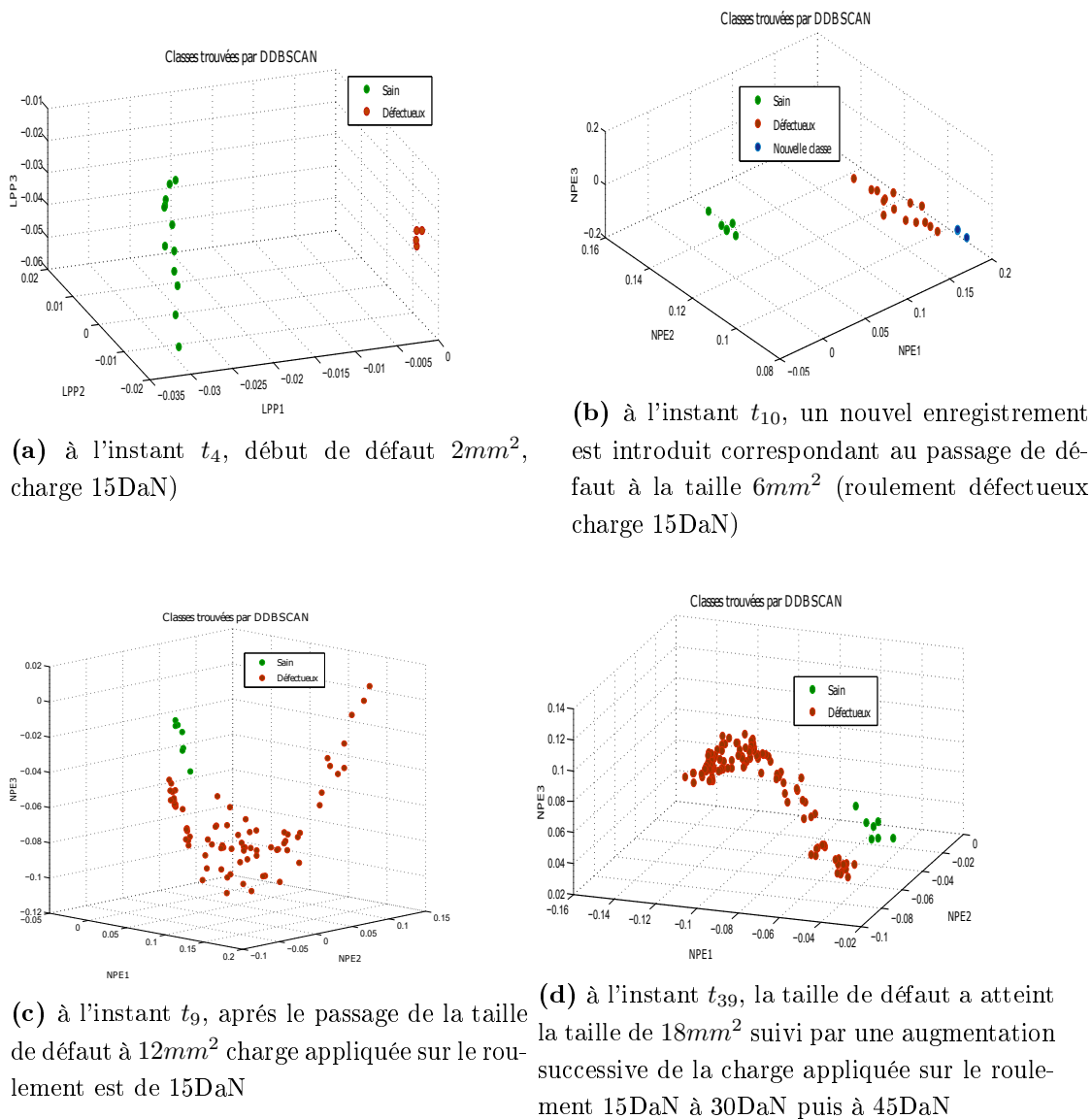
FIGURE 5.24 – Classification des observations reçues pour des roulements sous charge variable et avec un niveau de dégradation avancé
