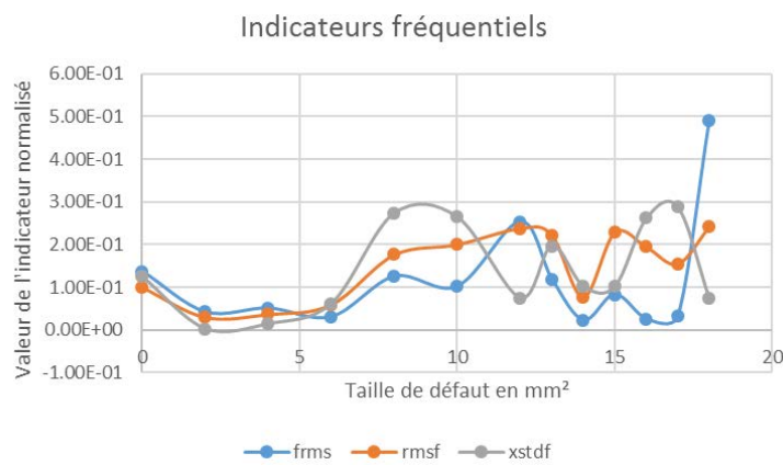
FIGURE 5.6 – les indicateurs fréquentiels calculés à partir de la puissance de spectre
