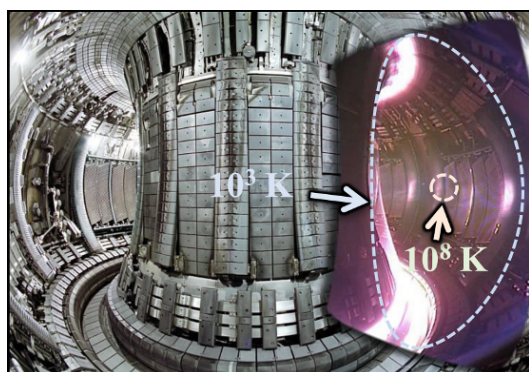
FIGURE A.1 – Composition de photographies de l'intérieur d'un tokamak. Les températures du cœur et du bord sont indiquées en ordre de grandeur. Photo : CCFE, EFDA-JET.
