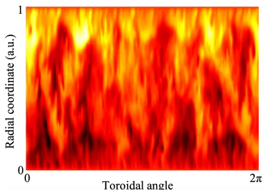
FIGURE A.2 – Illustration de la turbulence. Fluctuations du potentiel électrique obtenu dans une simulation TERESA.
