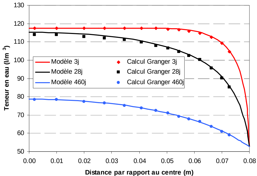
Figure III-10 : Profils des teneurs en eau à différentes dates
