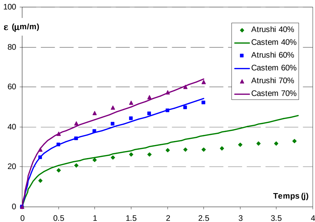
Figure III-21 : Déformation de fluage propre en traction pour plusieurs taux de chargement
