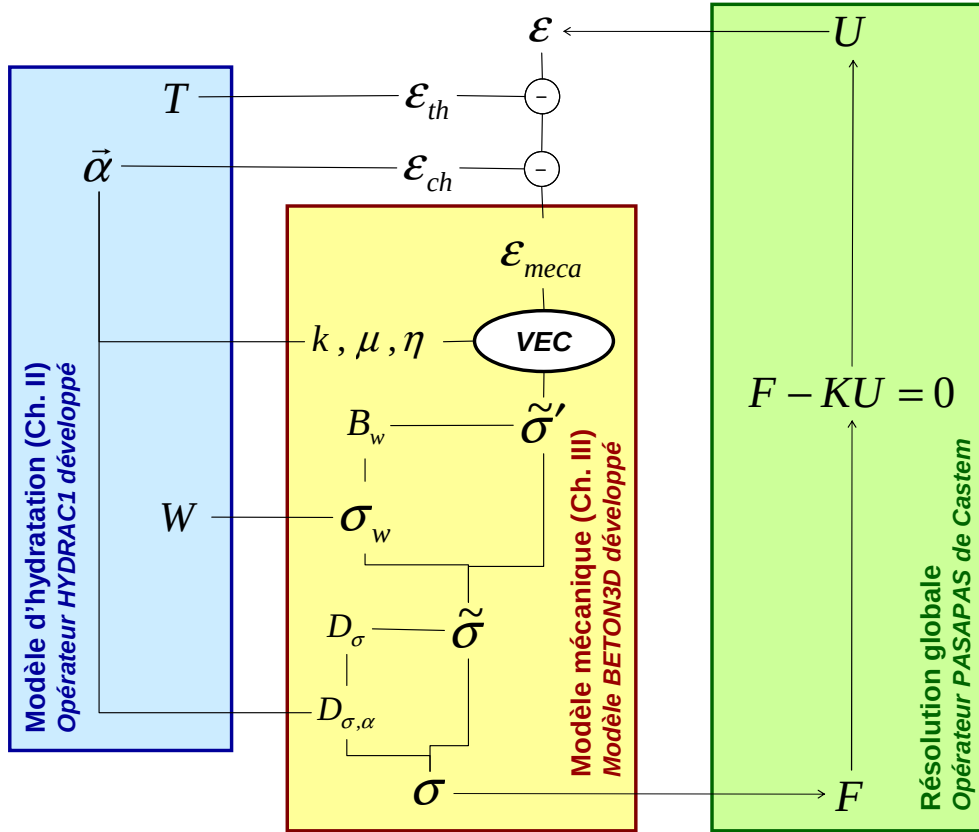
Figure III-4 : Principe de résolution du modèle mécanique au jeune âge proposé
