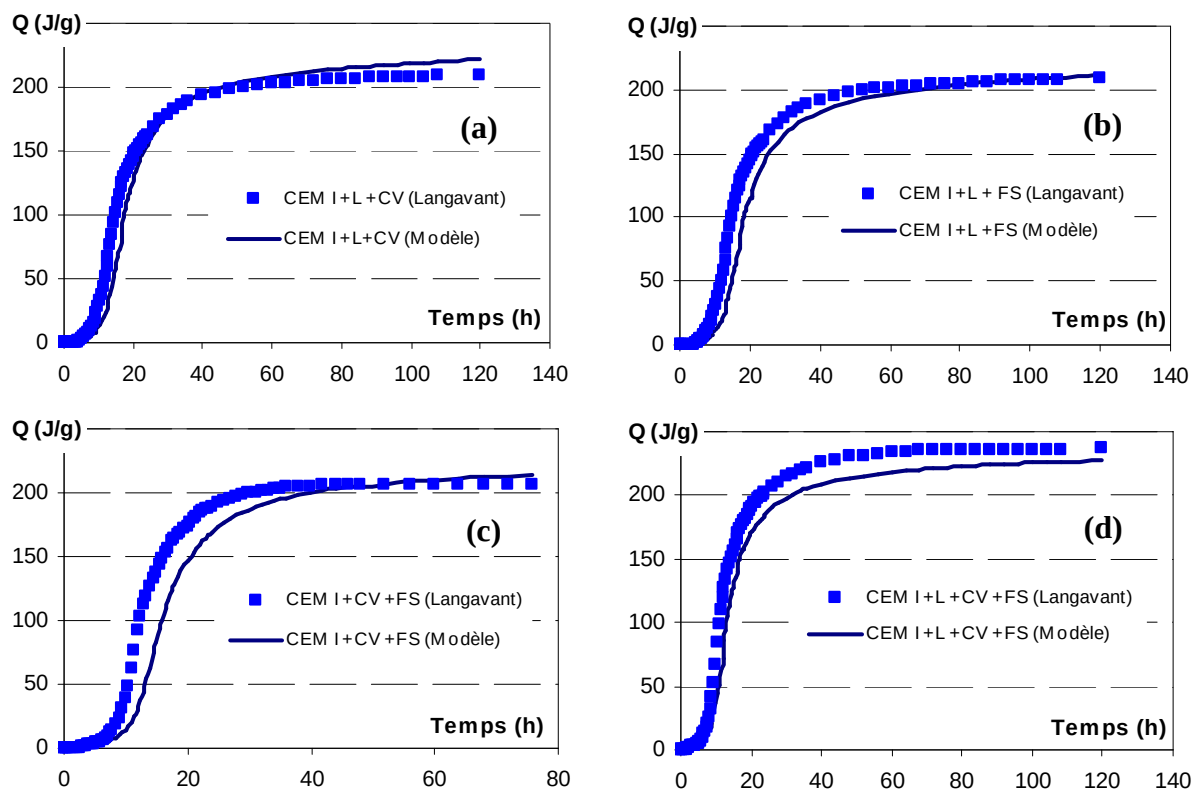
Figure II-12 : Dégagement de chaleur des liants composés ((a) C+L+CV, (b) C+L+FS, (c) C+CV+FS et (d) C+L+CV+FS)
