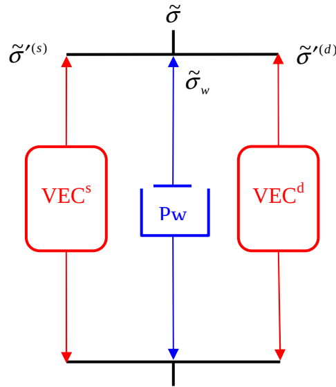
Figure III-2 : Schéma rhéologique du béton
