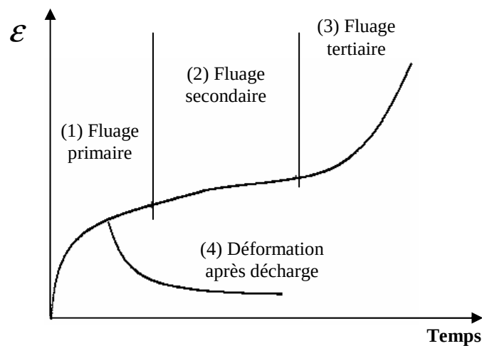
Figure I-20 : Définition des différents type de fluage
