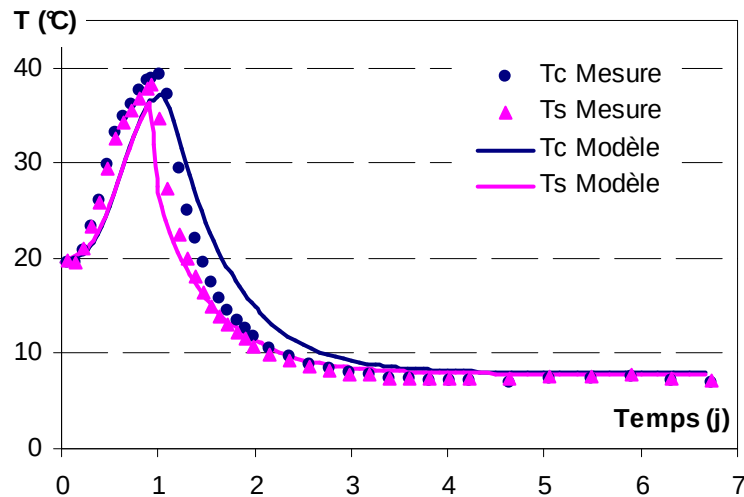
Figure III-31 : Evolution de la température de surface (Ts en rose) et au cœur (Tc en bleu) de la structure au cours du temps (trait continu = modélisation, marques = mesures)
