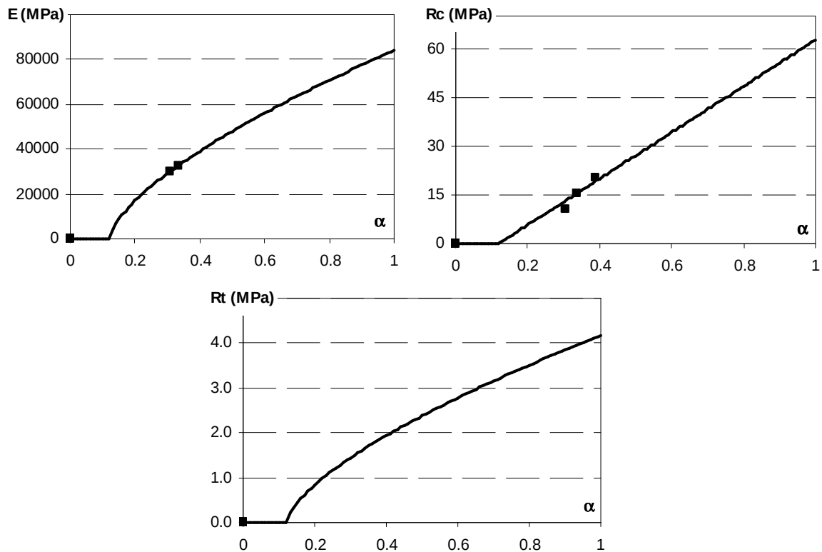
Figure III-30 : Evolution des caractéristiques instantanées au cours de l'hydratation
