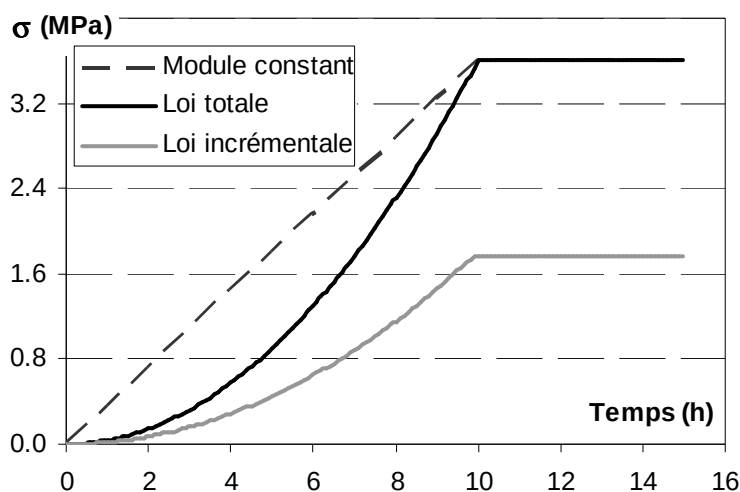
Figure D-4 : Evolution de la contrainte déterminée par les lois totale et incrémentale dans le cas d'un matériau en cours d'hydratation
