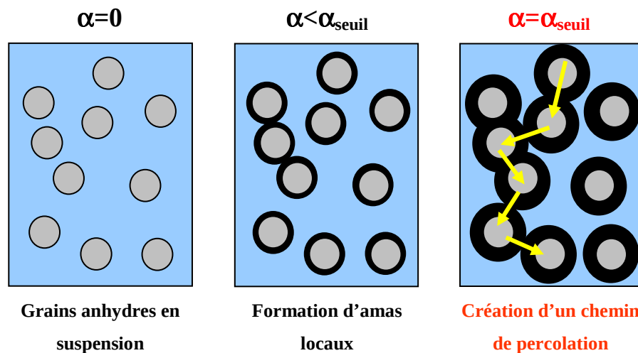
Figure I-10 : Illustration de la création d'un chemin de percolation entre phases solides
