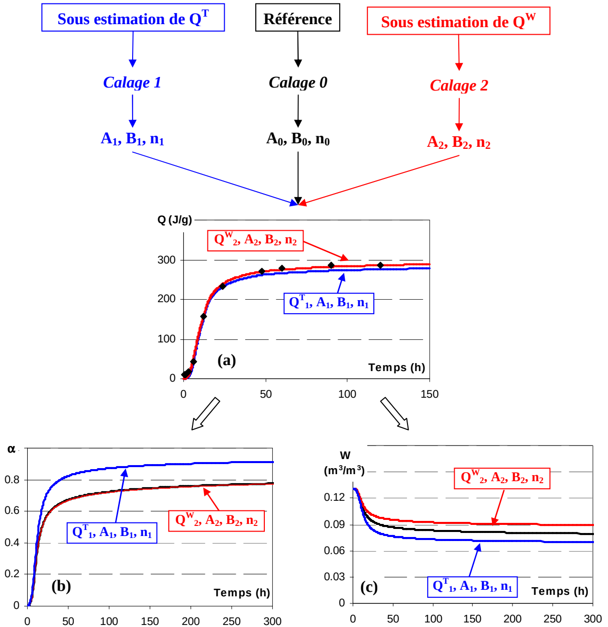
Figure II-10 : Influence des variations des paramètres sur T , \alpha et W .
