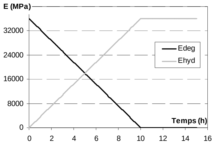
Figure D-1 : Evolutions des modules d'élasticités
