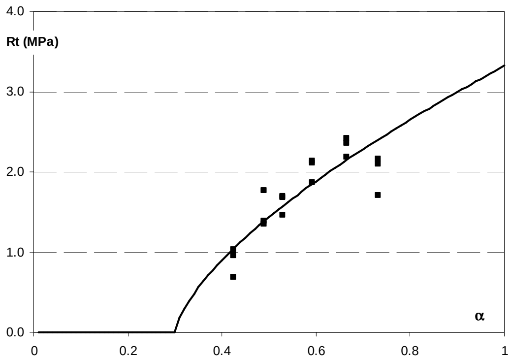
Figure III-16 : Evolution de la résistance en traction au cours de l'hydratation
