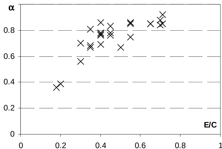
Figure I-3 : Valeurs du degré d'hydratation final d'un CEM I pour divers E/C [WALLER 99]
