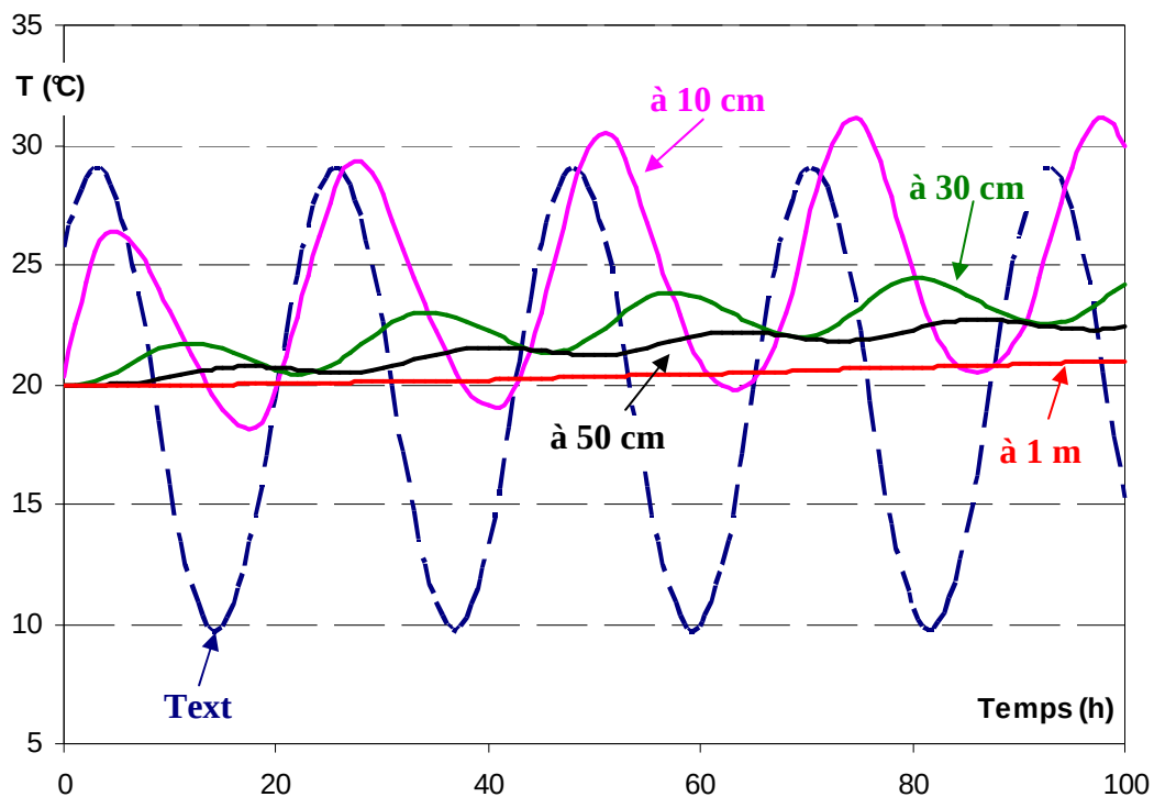
Figure II-5 : Evolution de la température d'un bloc de béton inerte soumis à une température extérieure variable (sinusoïdale) et à un flux solaire imposé (les distances indiquent les profondeurs des mesures par rapport à la surface horizontale supérieure)
