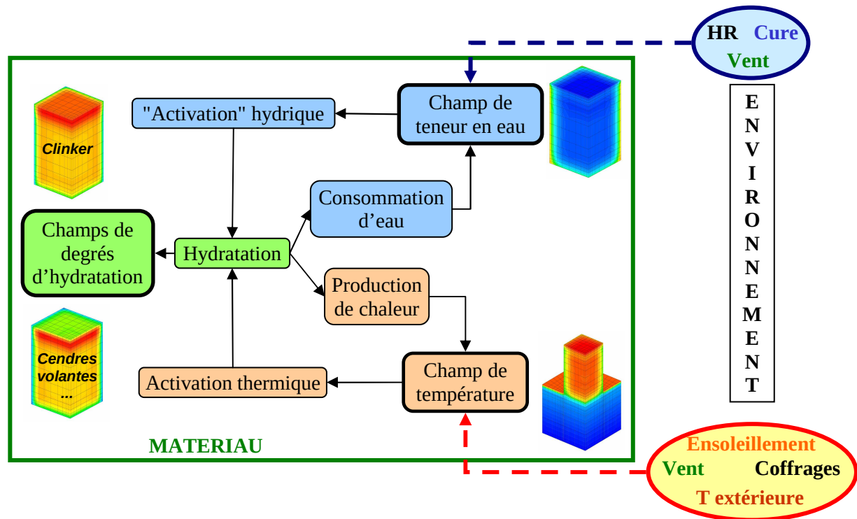
Figure II-1 : Principe des couplages du modèle multiphasique
