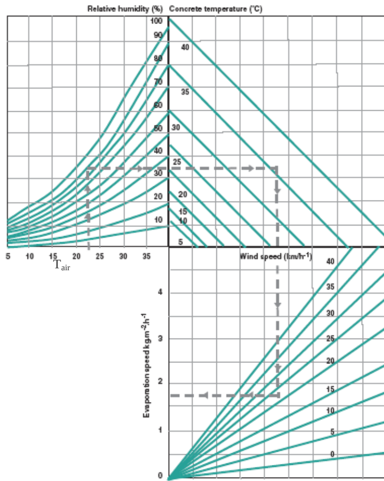
Figure I-6 : Abaque déterminant la vitesse d'évaporation de l'eau à la surface du béton [ACI 305R-99]
