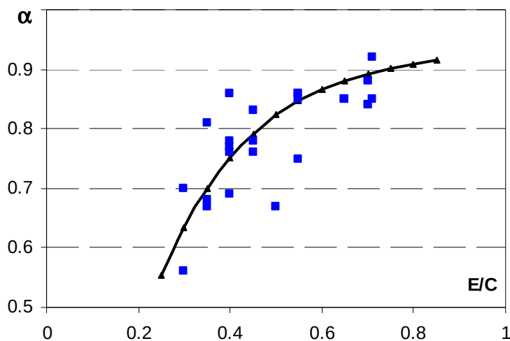
Figure II-13 : Valeurs atteintes par le degré d'hydratation à très long terme pour des pâtes à base de CEM I formulées avec plusieurs E/C (courbe = résultats modèle, marques = résultats donnés par [WALLER 99])
