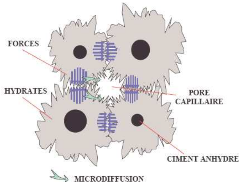
Figure I-21 : Phénomènes de microdiffusion à l'origine du fluage à court terme [ULM ET AL. 98b]
