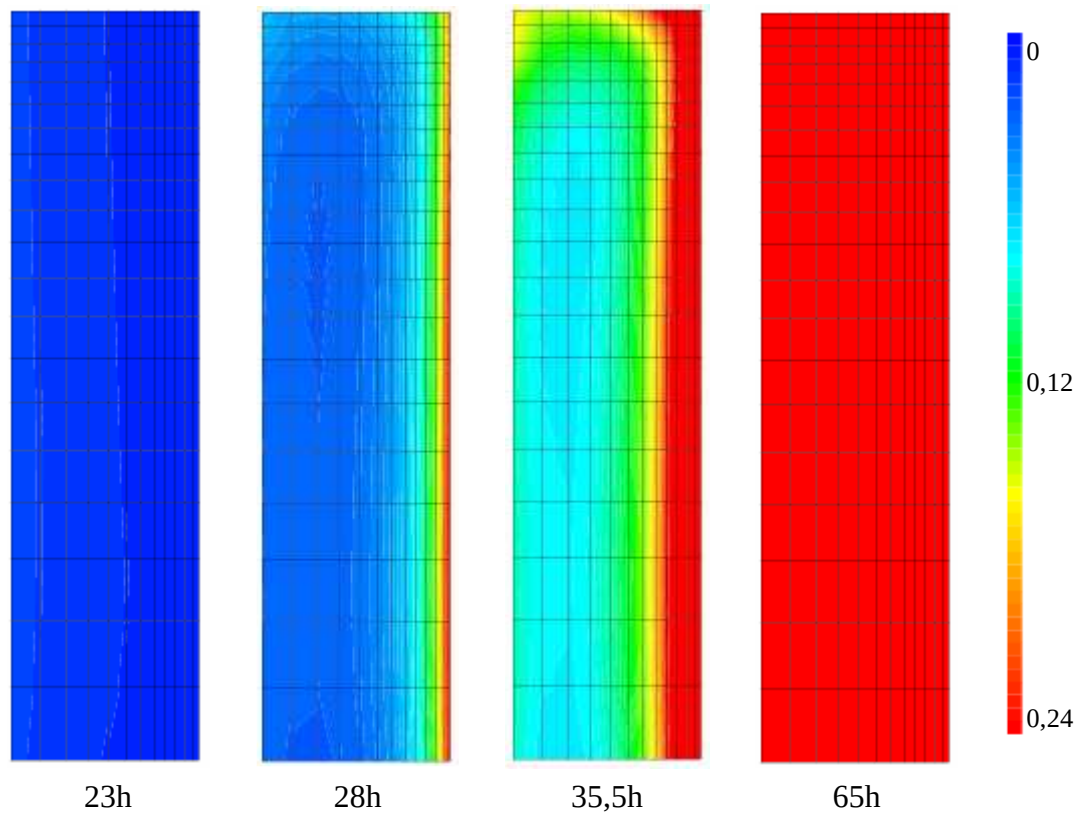
Figure III-26 : Evolution de l'indice de fissuration \beta_f^t dans l'anneau en béton (la valeur 0,24 correspondant à la localisation de la fissuration)
