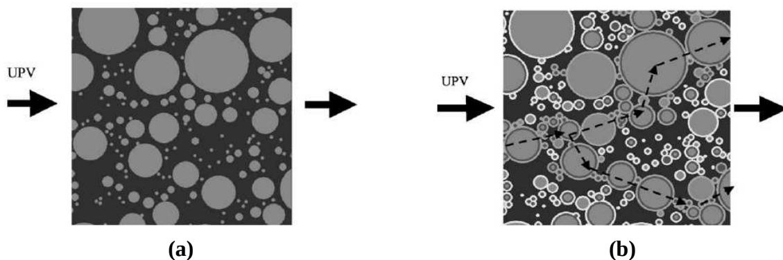
Figure I-11 : Illustration de la propagation des ondes acoustiques dans le béton avant le seuil de percolation (a) et après la création d'un chemin de percolation (b) [YE ET AL. 04]
