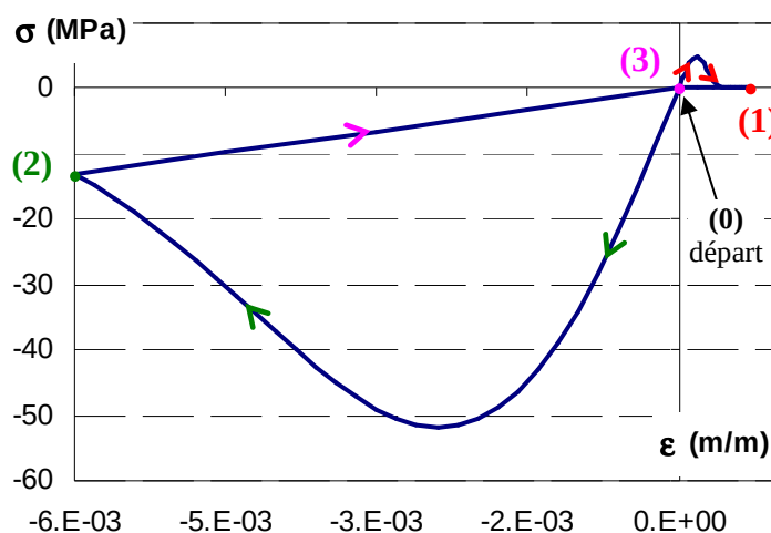
Figure III-6 : Réponse du modèle à un chargement cyclique
