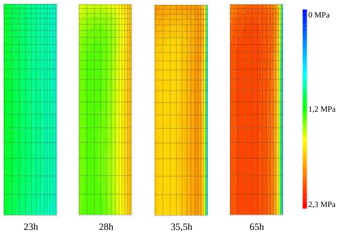
Figure III-25 : Evolution de la contrainte \sigma_{\theta\theta} dans l'anneau en béton
