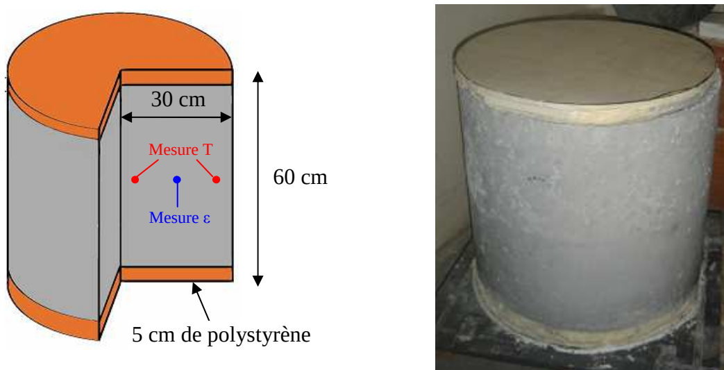
Figure III-28 : Structure décoffrée et à 7°C (21h à 7j)
