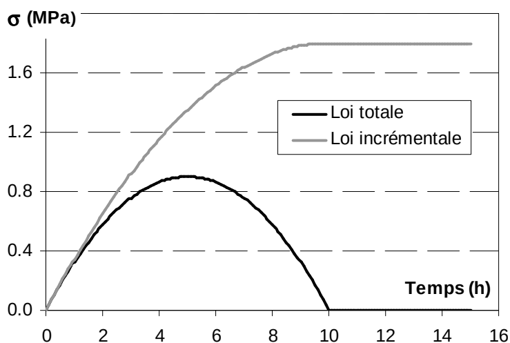
Figure D-3 : Evolution de la contrainte déterminée par les lois totale et incrémentale dans le cas d'un matériau en cours de dégradation
