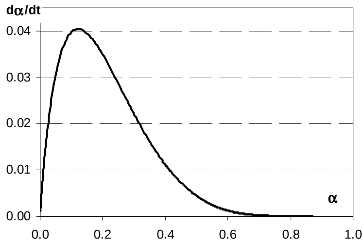
Figure II-3 : Variation de la loi cinétique pour un clinker (en conditions endogènes et isothermes)
