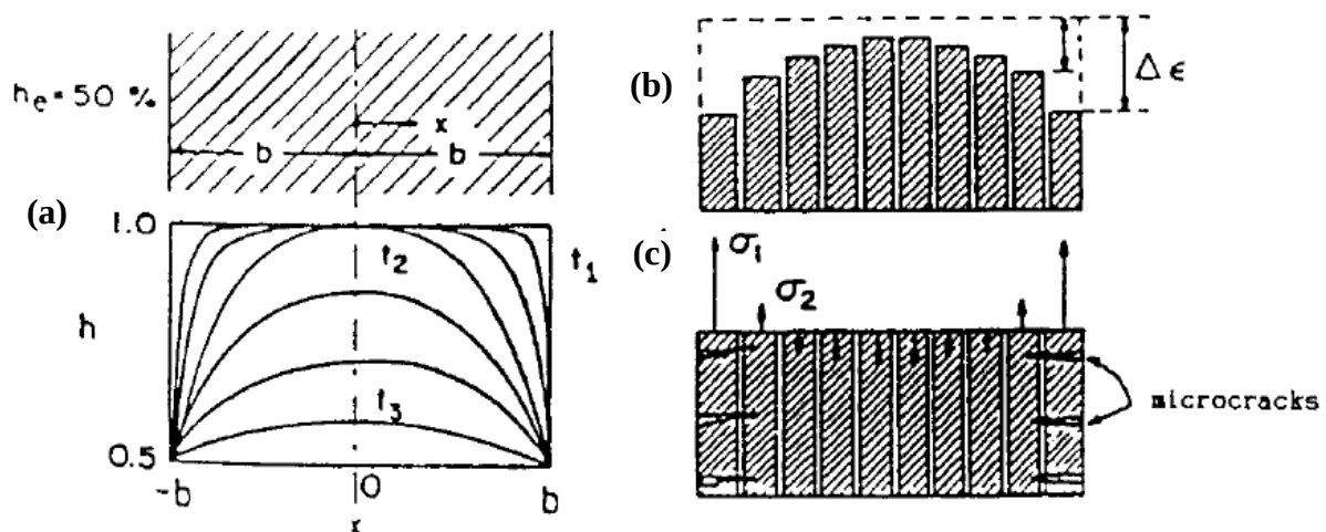
Figure I-18 : Profils d'humidité relative (a), retrait de dessiccation (b) et fissuration (c) induits (figure d'après Bazant reproduite dans [ACKER 97])
