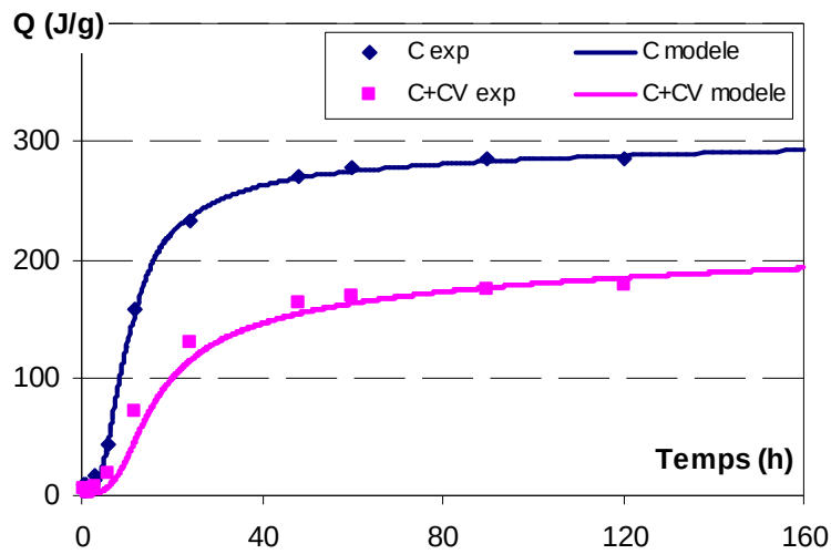
Figure II-16 : Calage de la loi de cinétique d'hydratation sur les mesures de dégagement de chaleur obtenues par l'essai de calorimétrie de Langavant
