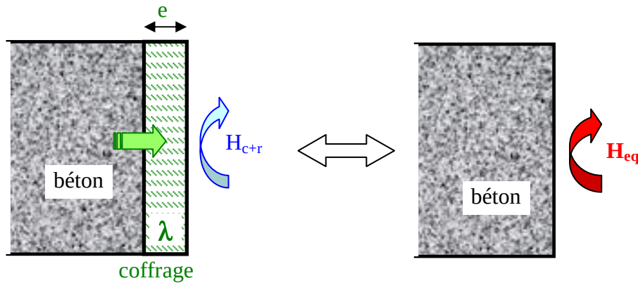
Figure II-4 : Principe du modèle série pour le calcul du coefficient d'échange équivalent
