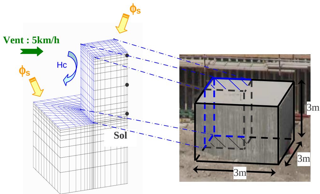
Figure II-15 : Présentation de la géométrie du quart de bloc modélisé
