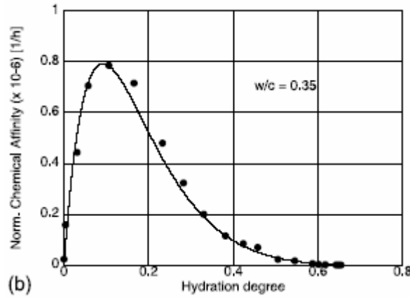
Figure I-2 : Evolution de l'affinité chimique A(\alpha) en fonction du degré d'hydratation [CERVERA ET AL. 02]
