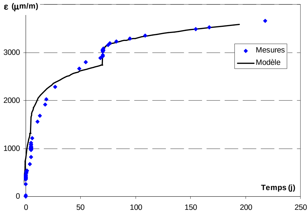
Figure III-20 : Déformation totale d'une éprouvette en fluage de dessiccation
