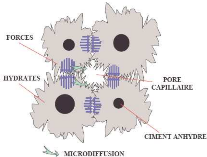
Figure I-21 : Phénomènes de microdiffusion à l'origine du fluage à court terme [ULM ET AL. 98b]
