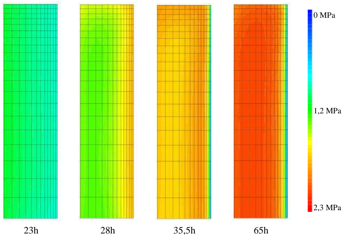
Figure III-25 : Evolution de la contrainte \sigma_{\theta\theta} dans l'anneau en béton
