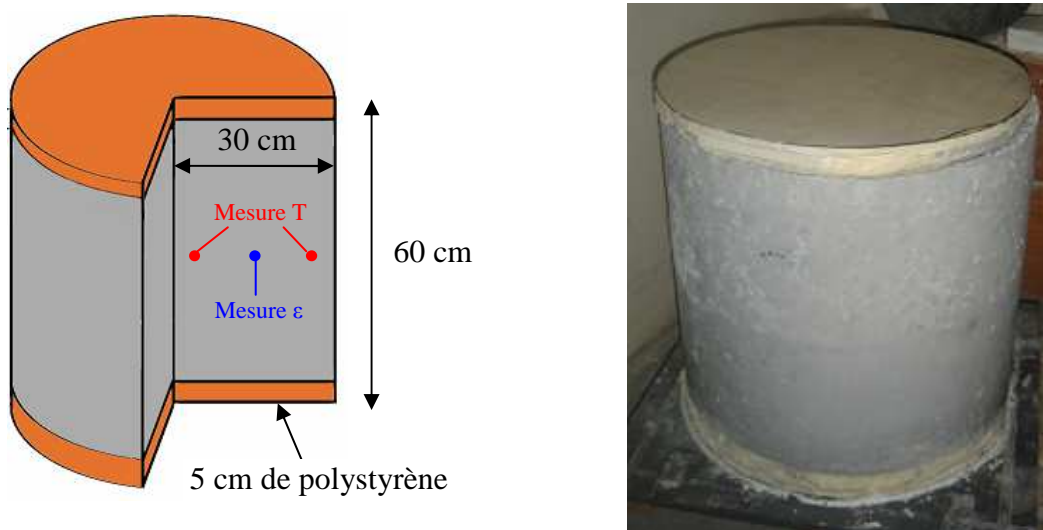
Figure III-28 : Structure décoffrée et à 7°C (21h à 7j)
