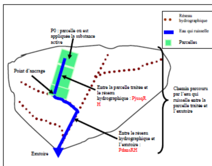
Figure 16 : description des 2 variables qui forment l'indice de connectivité, la variable P_{jusqRH} (rétention entre la sortie de la parcelle et le réseau hydrographique) et P_{dansRH} (rétention entre le point d'entrée dans le réseau hydrographique et l'exutoire) (Thiollet-Scholtus 2004)
