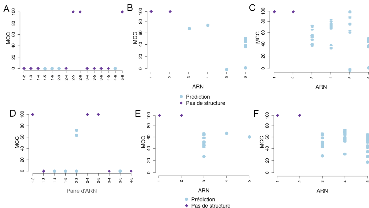
Figure 4.20 : MCC des interactions et des structures secondaires utilisées en entrée de C-RCPred pour les complexes B et C. A) Interactions prédites par l'outil RNAsubopt pour chaque paire d'ARN du complexe B. B) Structures secondaires prédites pour chaque ARN du complexe B par RME lorsque des données de PARS sont disponibles et par RNAsubopt et pKiss lorsqu'aucune donnée PARS est disponible. C) Structures secondaires prédites pour chaque ARN du complexe B par RNAsubopt et pKiss. D) Interactions prédites par l'outil RNAsubopt pour chaque paire d'ARN du complexe C. E) Structures secondaires prédites pour chaque ARN du complexe C par RME lorsque des données de PARS sont disponibles et par RNAsubopt et pKiss lorsqu'aucune donnée PARS est disponible. F) Structures secondaires prédites pour chaque ARN du complexe C par RNAsubopt et pKiss.
