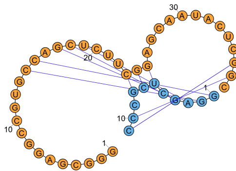
Figure 4.8 : Structure secondaire d'un exemple de pseudonœud de niveau 4 grâce à deux séquences d'ARN du complexe PDB_00851. Bleu : ARN 1, orange : ARN 2. Figure réalisée grâce à Ribosketch.
