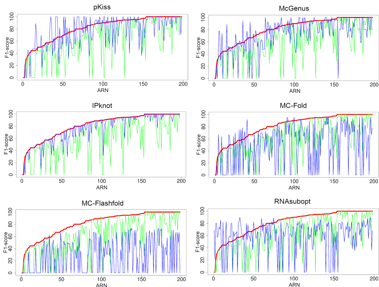
Figure 2.7 : F_1 -scores des solutions optimales obtenues par BiokoP comparé à pKiss, McGenus, IPknot, MC-Fold, MC-Flashfold et RNAsubopt sur le jeu de données B_{\text{nœud}} . Les F_1 -scores de BiokoP, minimum et maximum, sont respectivement en vert et en rouge, et celui des autres outils est en bleu.
