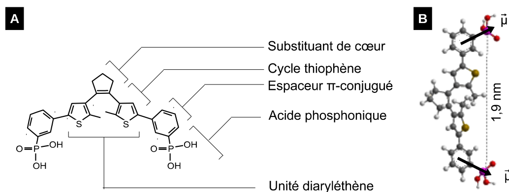
Figure 27: [A] : Représentation schématique de la molécule de DDA, [B] : Géométrie calculée par MOPAC et moments dipolaires de la molécule de DDA.
