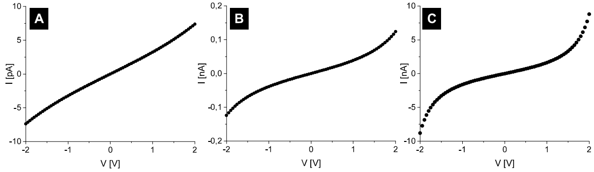
Figure 10: Caractéristiques I-V de jonctions moléculaires calculées à partir de l'équation 2.7 : [A] : où I @ \pm 2V = 7 pA ( \epsilon_F - \epsilon_{MO}(V=0) = 2,5 eV, \Gamma_1 = \Gamma_2 = 0,5 meV, T_m = 1 ), [B] : où I @ \pm 2V = 0,12 nA ( \epsilon_F - \epsilon_{MO}(V=0) = 1,5 eV, \Gamma_1 = \Gamma_2 = 1 meV, T_m = 1 ), [C] : où I @ \pm 2V = 9 nA ( \epsilon_F - \epsilon_{MO}(V=0) = 1,2 eV, \Gamma_1 = \Gamma_2 = 5 meV, T_m = 1 ).
