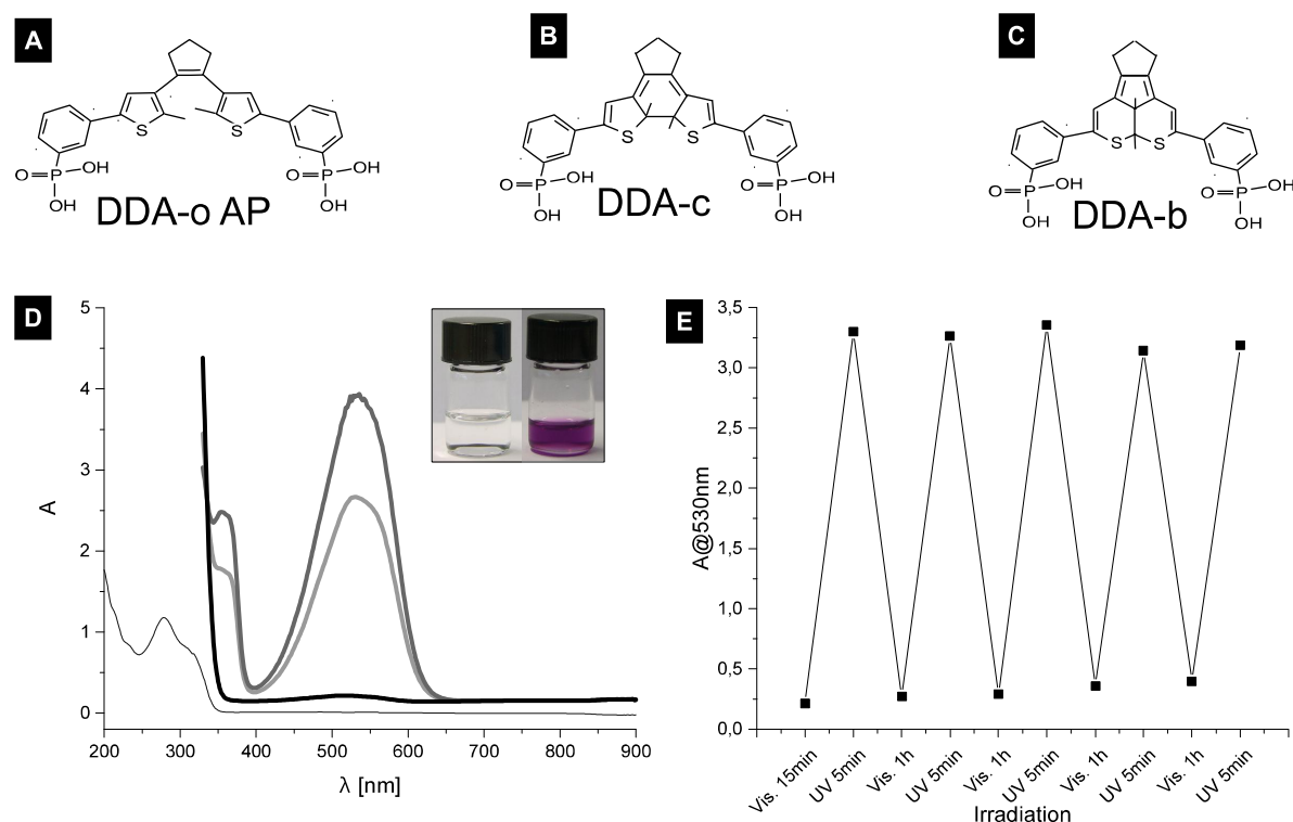
Figure 40: Représentations schématiques : [A] : du conformère DDA-o AP de la forme ouverte de DDA, [B] : isomère DDA-c et [C] : DDA-b, sous-produit de la réaction de photo-isomérisation DDA-o → DDA-c. [D] : Spectres d'absorbance optique de la solution éthanolique de DDA : trait fin : référence avant irradiation, trait épais, gris clair : après 2 min d'irradiation UV, gris foncé : après 3 min supplémentaires d'irradiation UV, noir : après 15 min d'irradiation Vis. Encart : Photographies d'une solution éthanolique de DDA avant (gauche) et après irradiation UV (droite). [E] : Absorbance optique à 530 nm au cours de 5 cycles UV/Vis.
