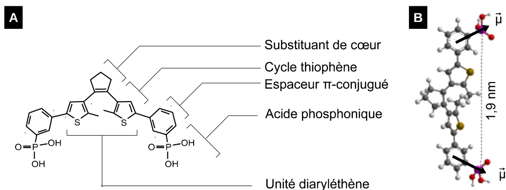
Figure 27: [A] : Représentation schématique de la molécule de DDA, [B] : Géométrie calculée par MOPAC et moments dipolaires de la molécule de DDA.
