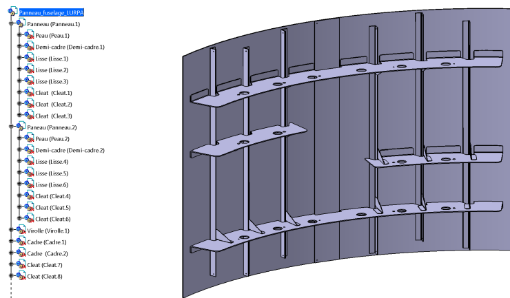
Figure 1.9 – Structure arborescente d'un panneau de fuselage assemblé
