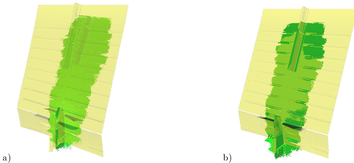
Figure 5.17 – Recalage entre les données mesurées et la géométrie du composant as-designed discrétisée (en jaune) : a) recalage grossier par ACP b) recalage fin par ICP
