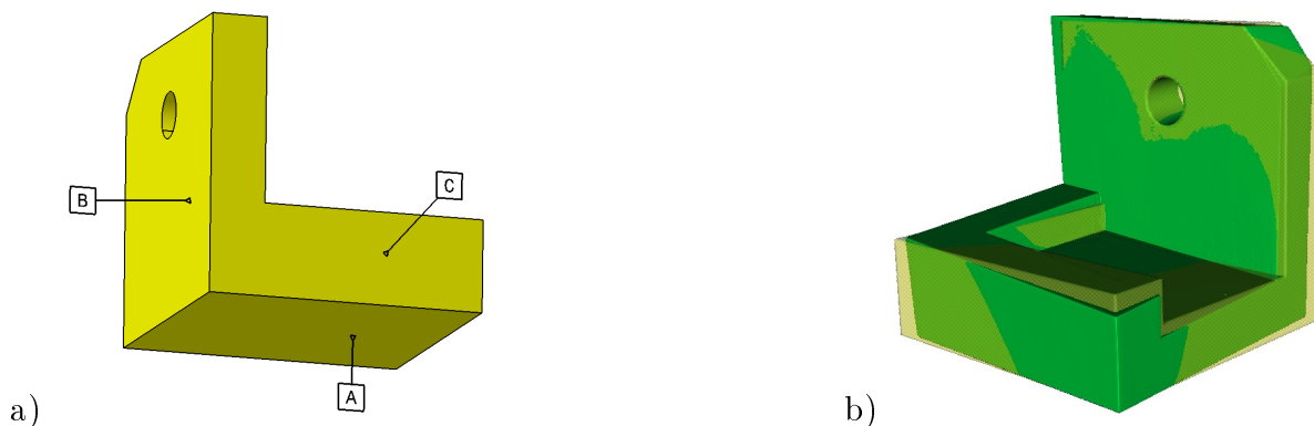
Figure 3.14 – Recalage des données mesurées sur les références globales
