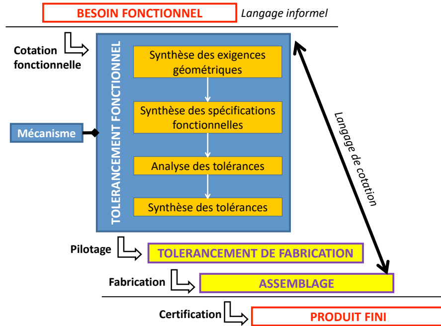
Figure 1.11 – Processus de tolérancement [Chavanne, 2011]
