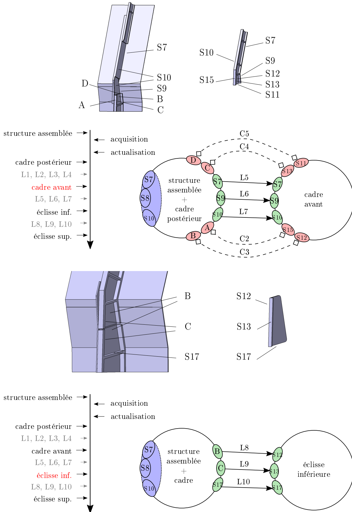
Figure 5.10 – Graphe Orienté Contact pour la 2 ème et la 3 ème étape de la séquence d'assemblage
