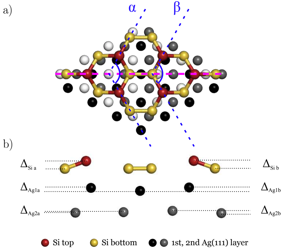
FIGURE 2: Vue de dessus (a) et latérale (b) de la reconstruction (4 \times 4) sur Ag(111). \alpha et \beta sont les angles indiqués par les lignes bleues. La représentation latérale correspondes à la ligne pointillée rose en (a).
