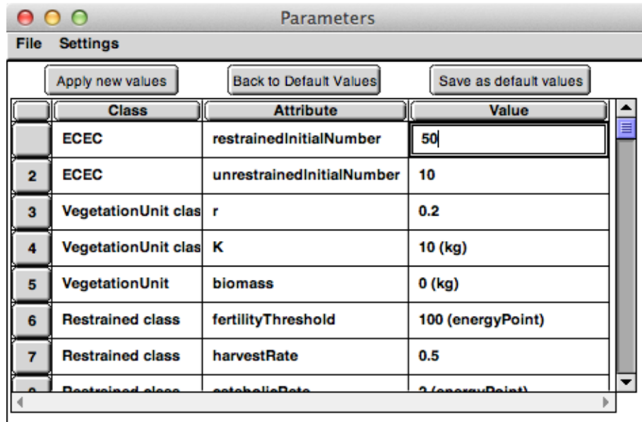
Figure 15: Parameter interface
